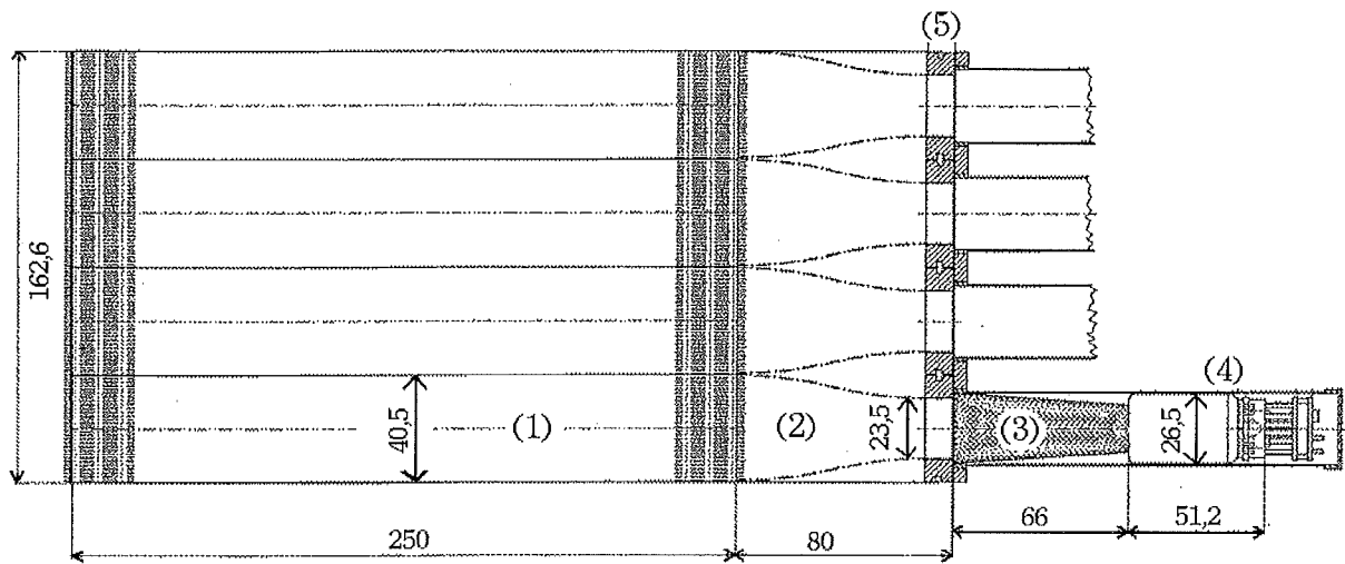
Abbildung 2.6: Longitudinaler Schnitt eines Supermoduls. Die untere Zelle ist komplett eingezeichnet mit dem Blei/Faser-Block (1), dem Faserbündel (2), dem Aluminiumrahmen (5), dem Lichtmischer (3) und dem Photomultiplier mit Basis (4). Alle Maßangaben in mm
