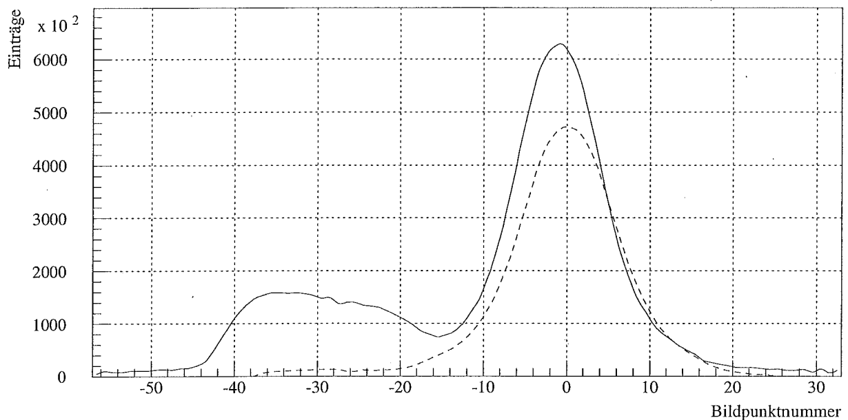
Abbildung 4.17: Dämpfung des Mantellichtes. Gezeigt ist jeweils ein Schnitt durch die Maxima der Signale aus Abbildung 4.16
