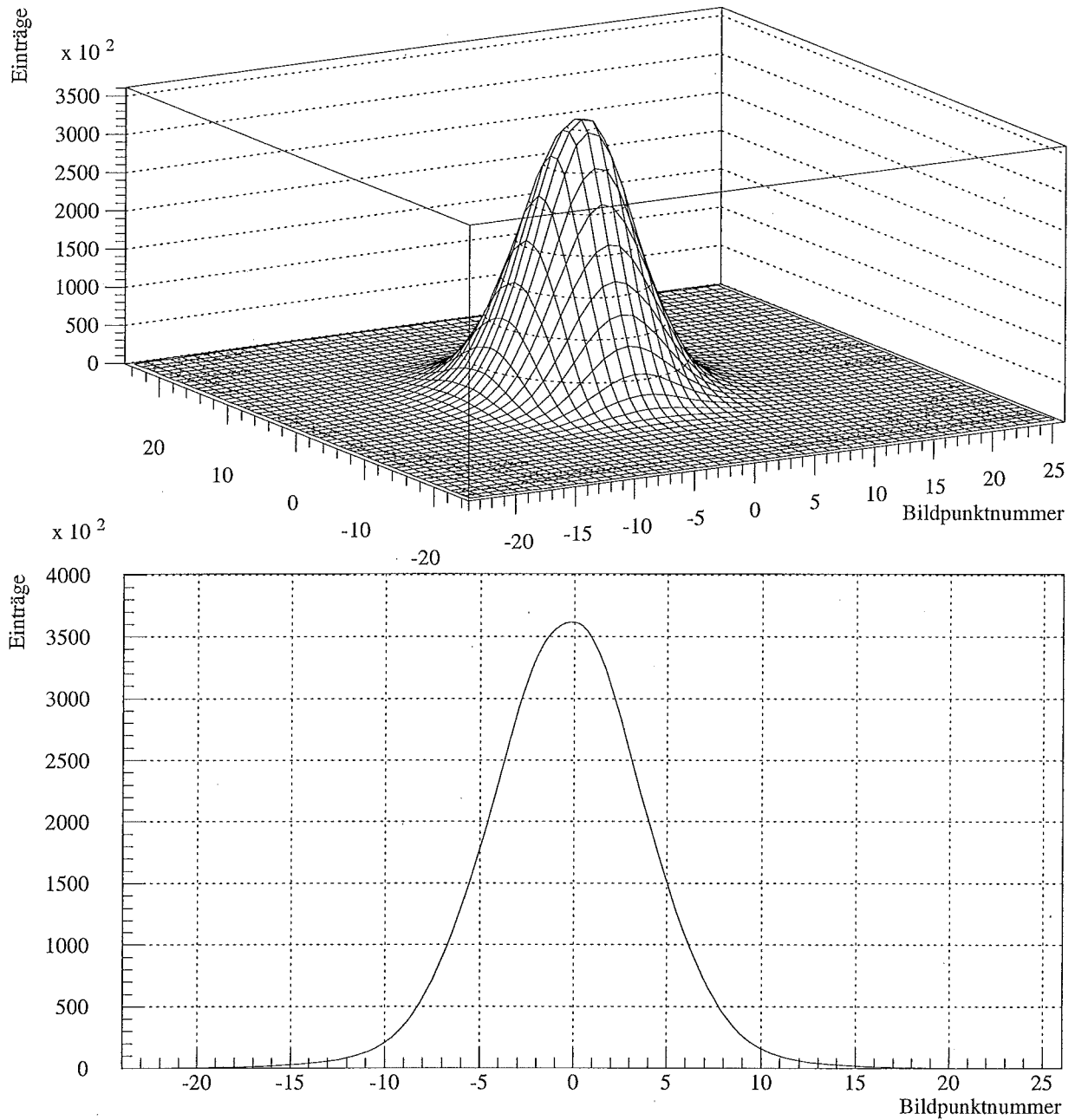
Abbildung 4.13: Darstellung eines typischen Fasersignals. Oben: dreidimensionale Graphik, unten: zweidimensionaler Schnitt durch das Signalmaximum
