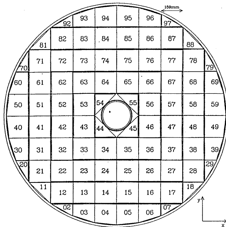
Abbildung 1.3: Schnitt durch das BEMC senkrecht zur Strahlachse [BEM 92]
