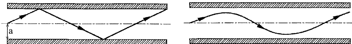
Abbildung 3.2: Lichtleitung in einer Faser mit Stufenprofil (links) bzw. Parabelprofil (rechts). Gezeigt ist jeweils ein Längsschnitt der Faser, wobei der schraffierte Bereich die Mantelschicht angibt [Ung 89]
