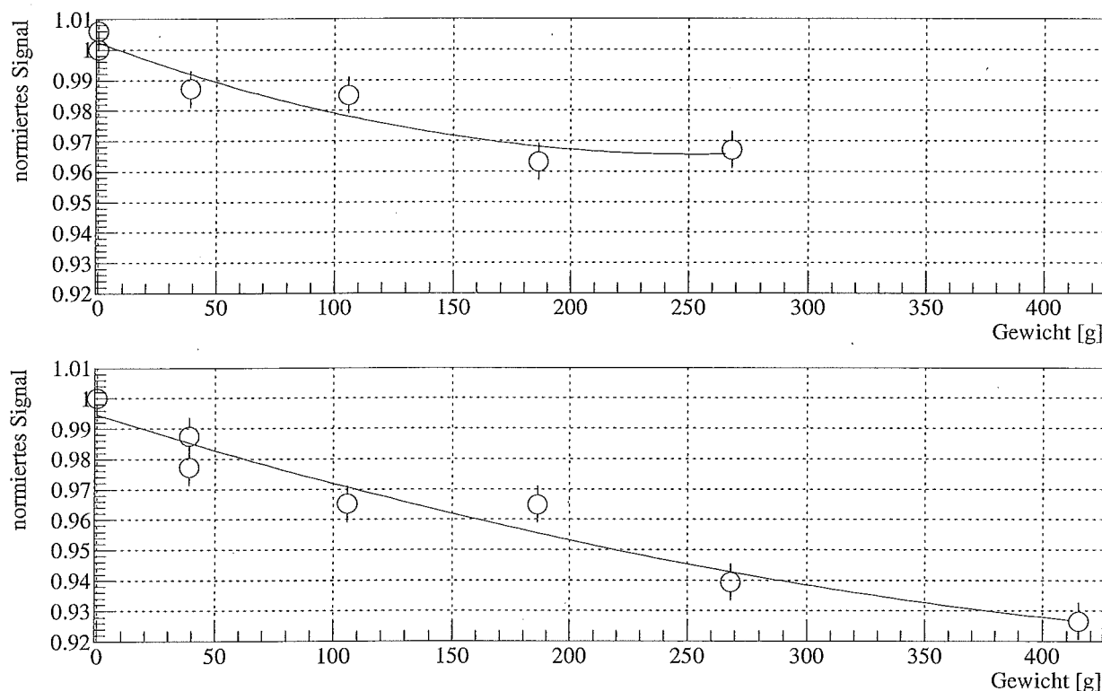
Abbildung 4.29: Einfluß von Druck auf die Intensität des Faserlichtes. Die Messungen wurden mit Aufbau 2 durchgeführt; auf Halterung 3 wurden verschiedene Gewichte gelegt und so Druck auf die Faser ausgeübt. Aufgetragen ist das Fasersignal in Abhängigkeit des aufgelegten Gewichtes. Oben: nur Kernlicht, unten: auch Mantellicht
