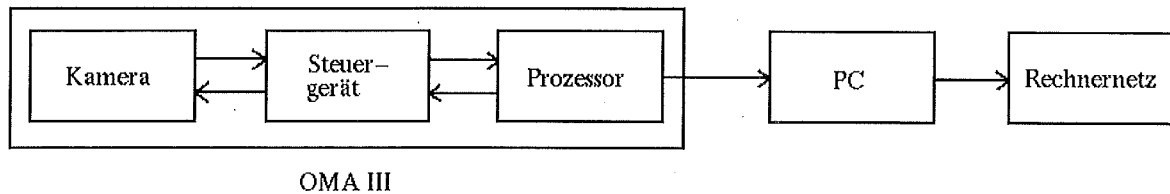
Abbildung 4.3: Die verwendeten Geräte zur Gewinnung und Auswertung der CCD-Daten
