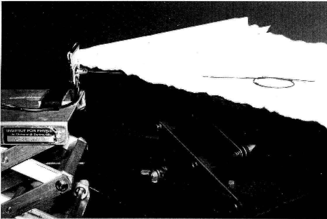
Abbildung 4.6: Das Prinzip des ersten Aufbaus. Das Photo zeigt zwei der drei Labortische. Auf dem rechten Tisch liegt eine zu einer Schleife gebundene Faser, die im gebogenen Teil geschwärzt ist. Auf dem linken Tisch ist eine LED montiert, die zur Lichteinkopplung in die Faser benutzt wird. Bei der abgebildeten LED handelt es sich um eine blau emittierende LED, die nur bei Aufbau 2 verwendet worden ist
