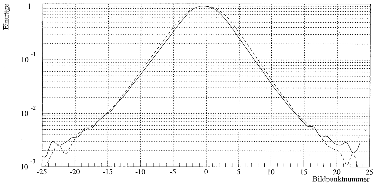
Abbildung 4.25: Einfluß einer Biegung auf die Winkelverteilung der Faser bei Lichteinkopplung mit der grünen LED. Die durchgezogene Linie gibt das Signal bei gerader Faser an, die gestrichelte Linie das bei gebogener Faser
