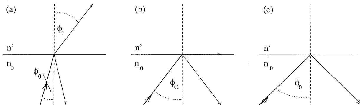
Abbildung 3.4: Das Verhalten eines Lichtstrahls an der Grenzschicht zweier Medien mit hohem und niedrigem Brechungsindex n_0 und n' . Der Strahl wird gebrochen (a), geht entlang der Grenzfläche (b) oder wird totalreflektiert (c)
