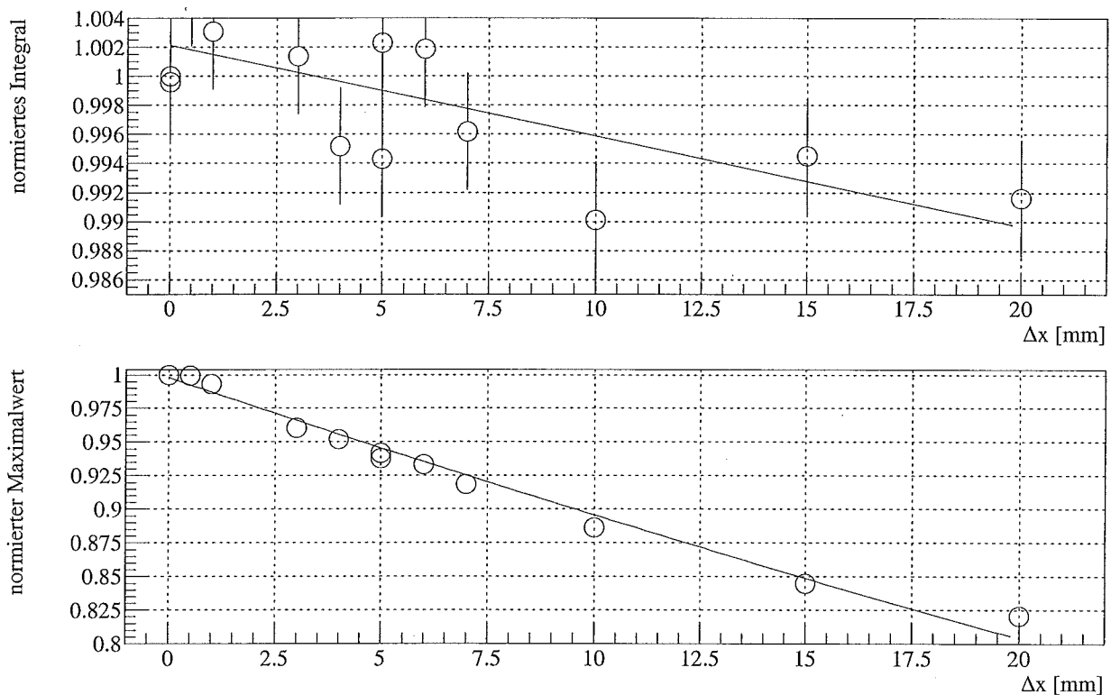
Abbildung 4.24: Einfluß einer Biegung auf die Intensität des Faserlichtes. Verwendet wurde Aufbau 2 mit der grünen LED zur Lichterzeugung
