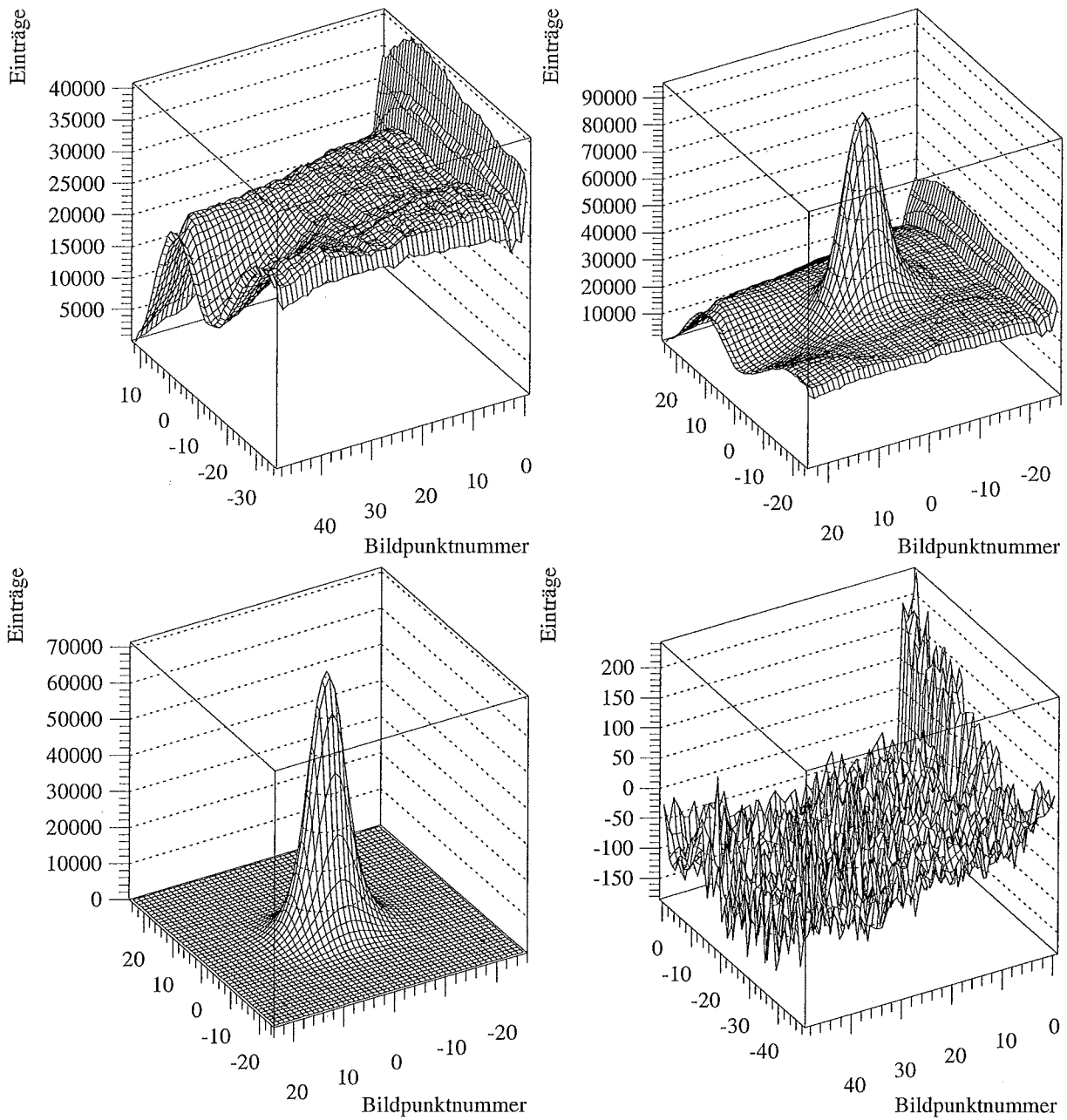
Abbildung 4.4: Gewinnung der Meßdaten mit der CCD-Kamera. Oben links: das Signal der Kamera bei einer Nullmessung. Oben rechts: das Kamerasignal bei Beleuchtung mit einer Faser. Unten links: die Differenz der beiden oberen Signale. Unten rechts: die Differenz zweier Nullmessungen mit zweiminütigem Abstand. Der Bildpunkt mit den meisten Einträgen hat jeweils die Nummer (0/0)
