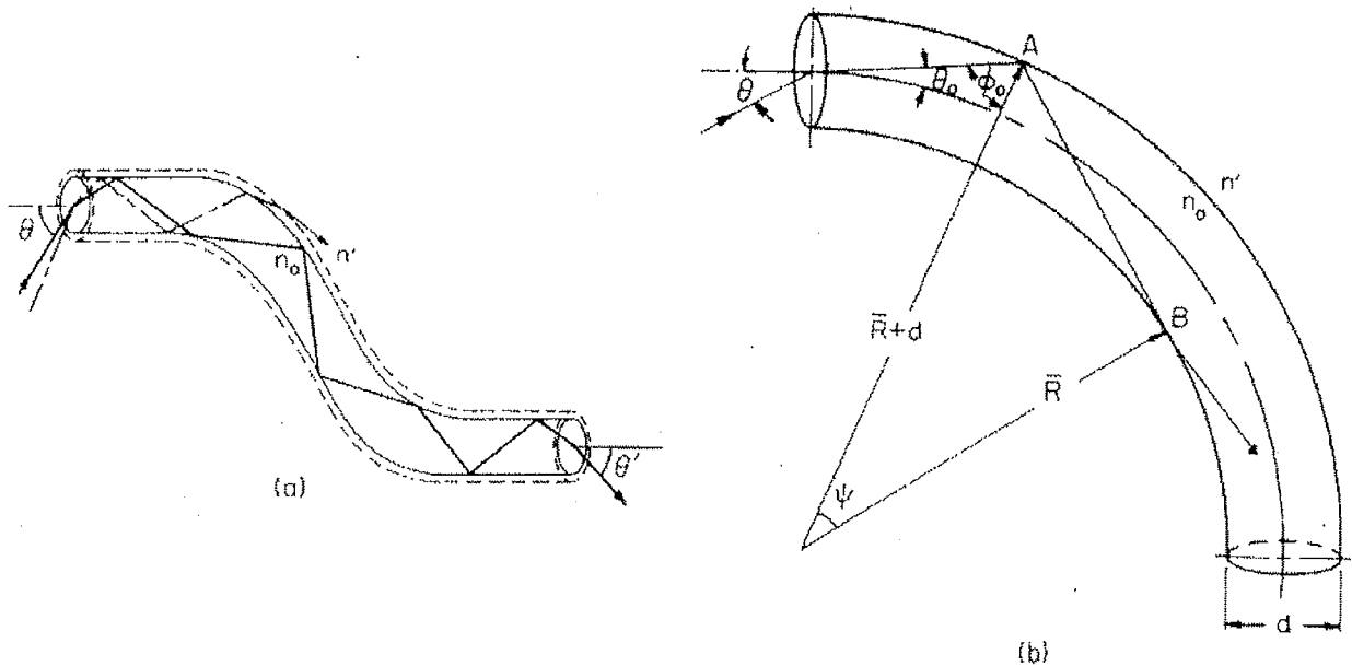
Abbildung 3.6: Strahlengang durch gebogene Fasern. (a): Ein Strahl wird aus der Faser herausgebrochen, der andere Strahl wird durch die Faser geleitet. Der Fasermantel ist gestrichelt eingezeichnet. (b): Eine zu einem Torusstück gebogene Faser; der Fasermantel ist nicht eingezeichnet. Zur Definition des Winkels \theta_0 Siehe Abb. 3.5 [Kap 67]
