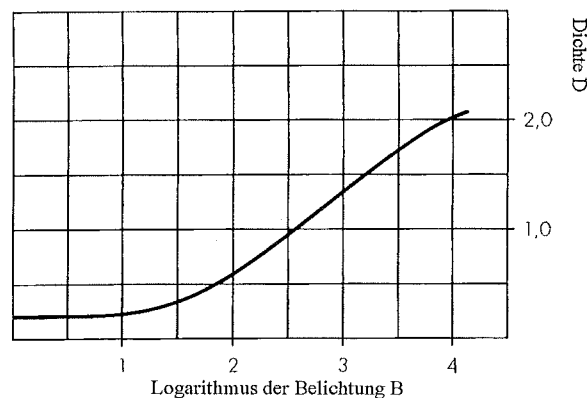
Abbildung 4.2: Schwärzungskurve eines Films [Ilf 93]
