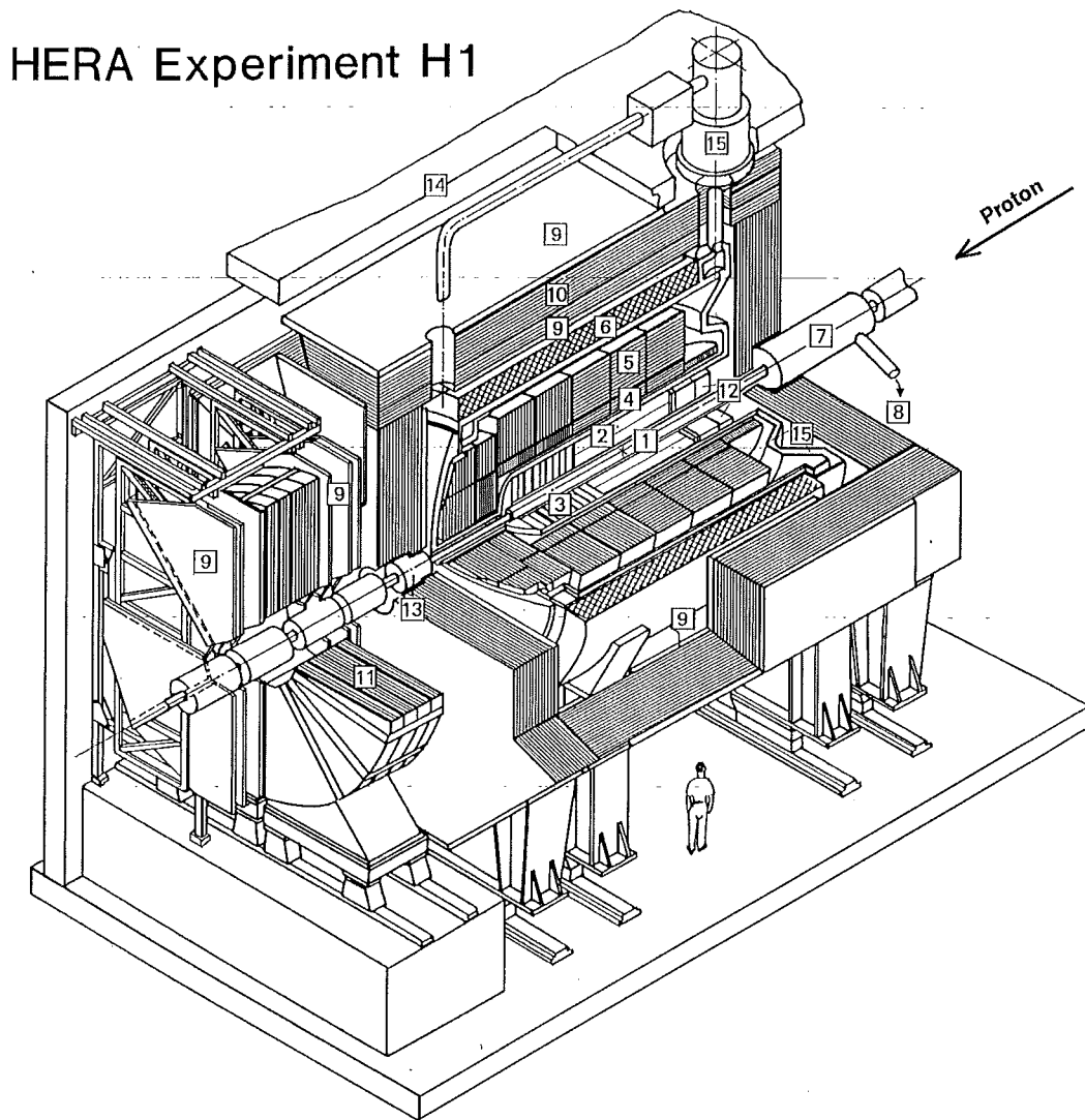
Abbildung 1.2: Perspektivische Ansicht des H1-Detektors
