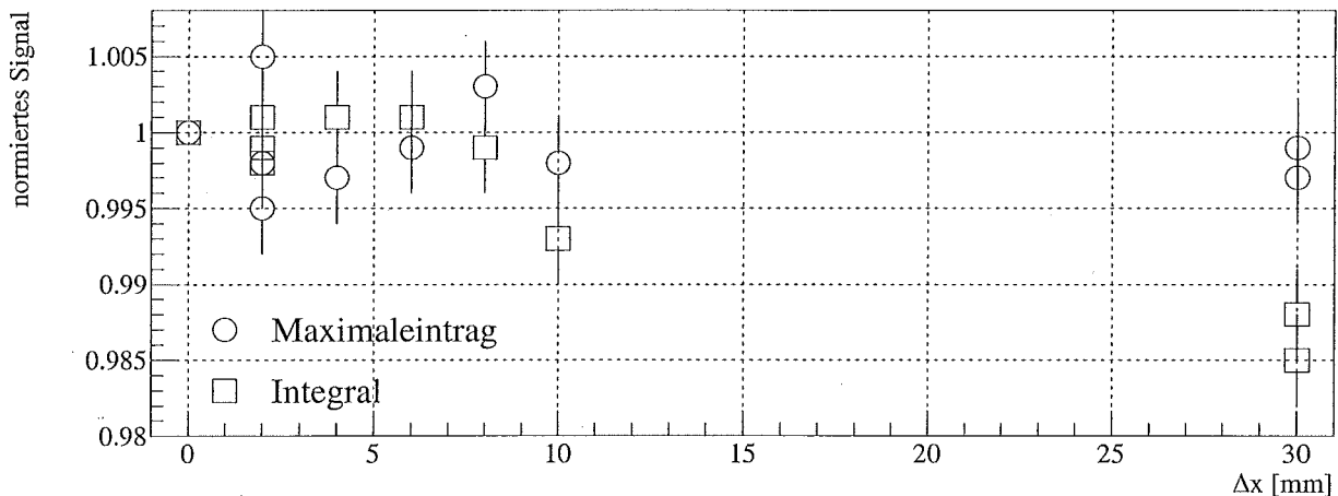
Abbildung 4.27: Einfluß der Integralgröße auf das Verhalten des Fasersignals bei einer Biegung bei Anregung der Faser mit UV-Licht. Aufgetragen ist das Fasersignal in Abhängigkeit von der Biegung
