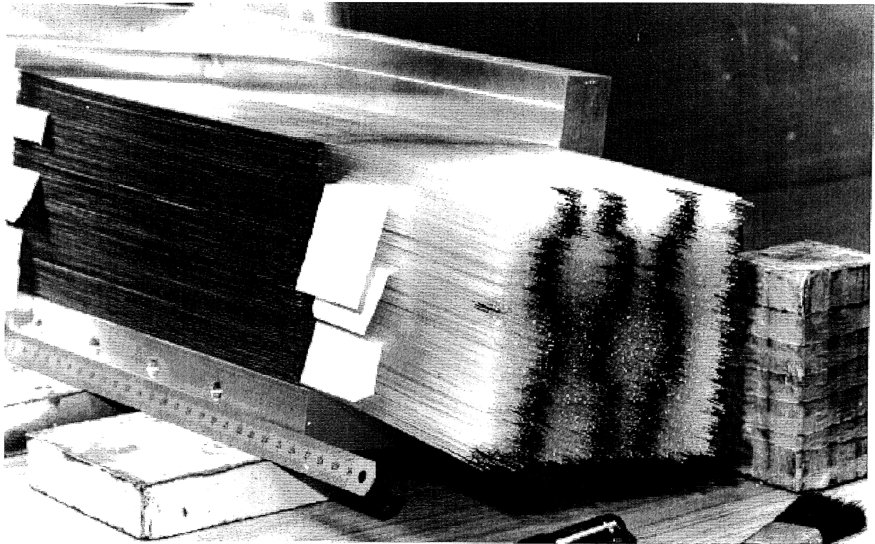
Abbildung 2.7: Photo der ersten Bauphase eines Prototypen. Zu sehen sind die zu einem Block gestapelten Bleiplatten, aus dem die Fasern austreten [Des 93]
