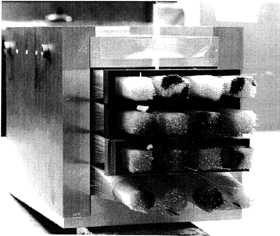
Abbildung 2.8: Photo der zweiten Bauphase eines Prototypen. Der Blei/Faser-Block wird durch ein Metallgehäuse gestützt, die Fasern sind bereits gebündelt und teilweise in Aluminiumrahmen befestigt [Des 93]
