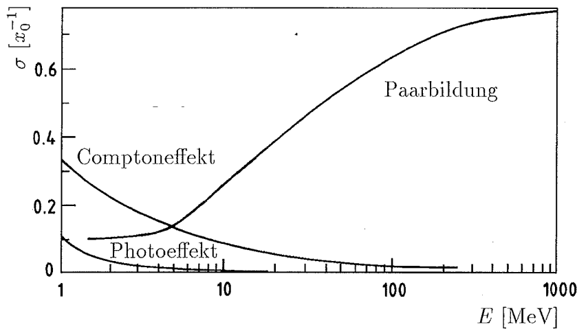
Abbildung 2.3: Wechselwirkungswahrscheinlichkeit pro Strahlungslänge X_0 eines Photons in Blei als Funktion der Energie [Par 90]
