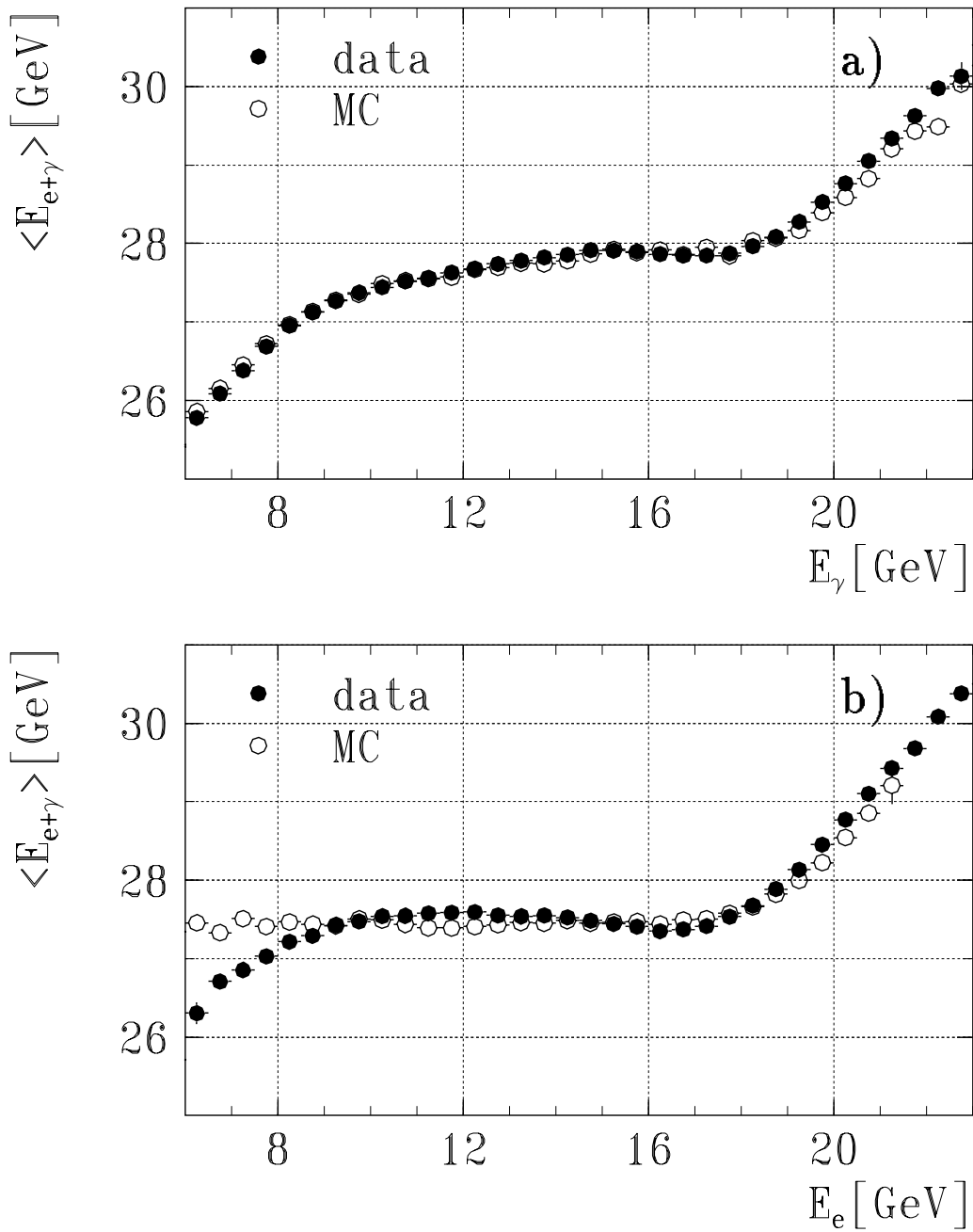
Abbildung 6.7: Überprüfung der Interkalibrierung zwischen Elektronendetektor und Photondetektor anhand von Bremsstrahlungsereignissen, entnommen aus [Gog96]. E_e bezeichnet die im Elektronendetektor rekonstruierte Energie E_{ET} und E_\gamma entspricht der Energiesumme E_{PD} + E_{VC} . Weiterhin gilt: E_{e+\gamma} = E_{ET} + E_{PD} + E_{VC} . Die Simulationrechnungen wurden mit dem Programmpaket H1LUMI [Lev93] durchgeführt.
