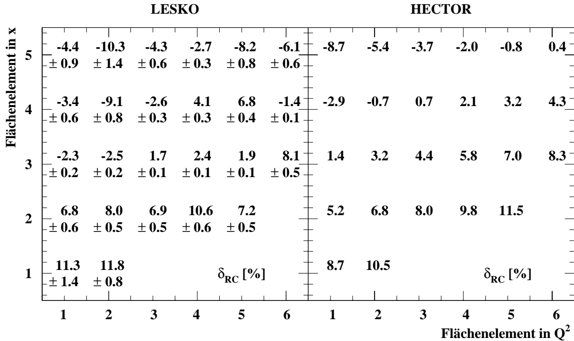
Abbildung 7.16: Strahlungskorrekturfaktor \delta_{RC} [\%] für die Elektron-Methode bei Verwendung der Programmpakete LESKO [Jad91] und HECTOR [Arb95]. Da das Programmpaket HECTOR keine Ereignisse erzeugt, sondern analytische Berechnungen durchführt, können keine statistischen Fehler angegeben werden.
