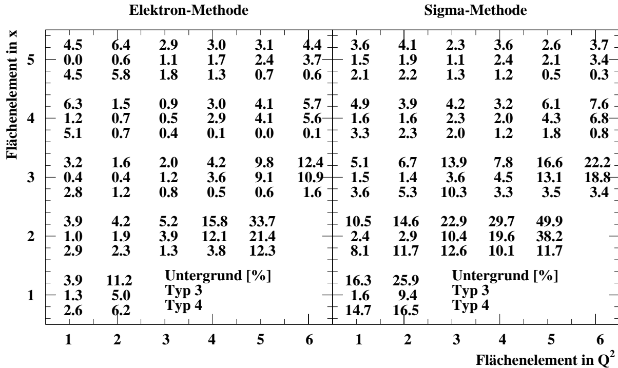
Abbildung 7.15: Prozentualer Anteil an Untergrundereignissen für die selektierten Flächenelemente bei Verwendung der Elektron- und der Sigma-Methode. Die obere Zahl gibt den gesamten Untergrundanteil an, der sich aus Zufallskoinzidenzen tiefinelastischer Ereignisse (mittlere Zahl) und Photoproduktionsereignissen (untere Zahl) mit Bremsstrahlungereignissen zusammensetzt.
