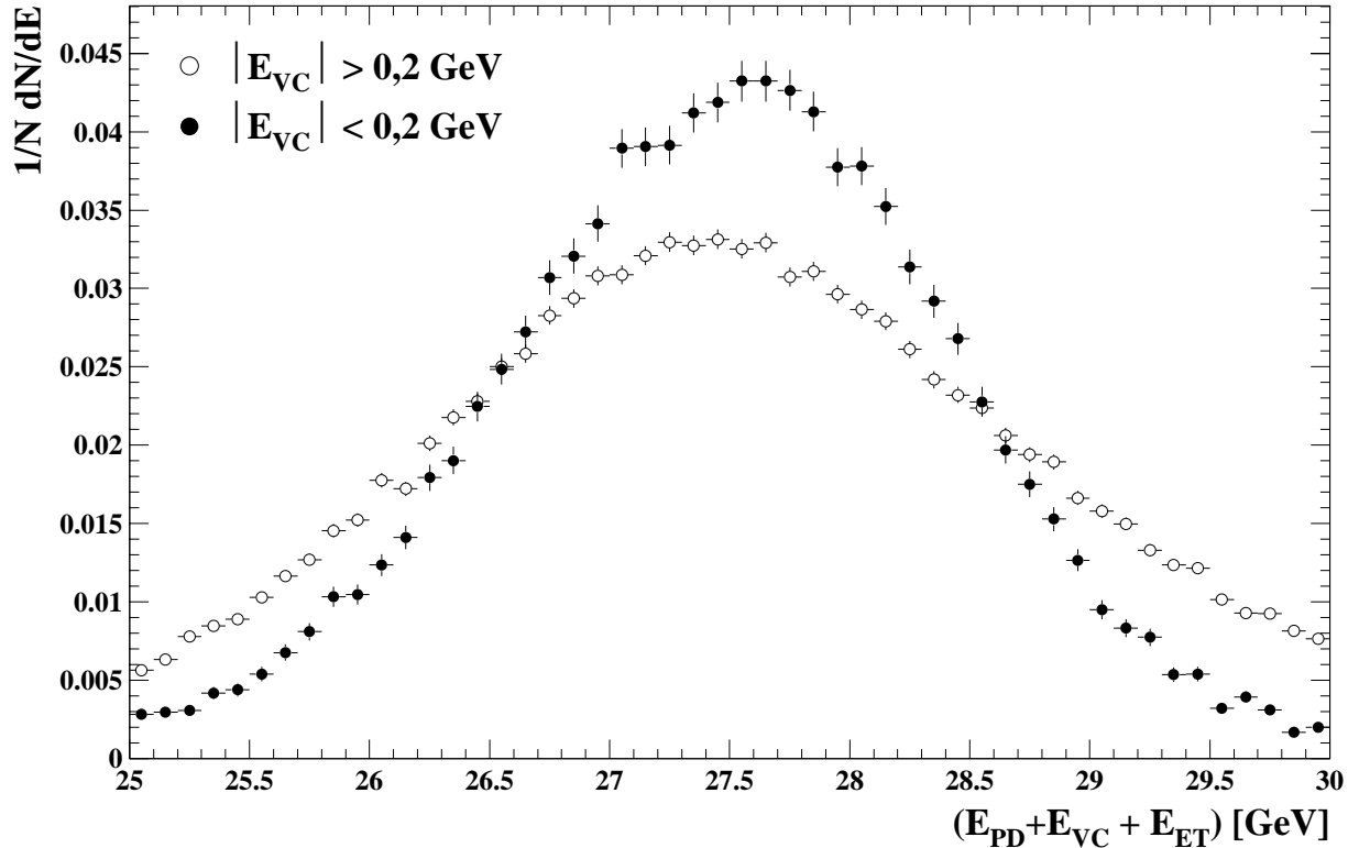
Abbildung 6.3: Verteilung der Energiesumme ( E_{PD} + E_{VC} + E_{ET} ) für die zwei Stichproben von Bremsstrahlungsereignissen mit E_{VC} > 0,2 \text{ GeV} und E_{VC} < 0,2 \text{ GeV} . Die Histogramme sind auf die Anzahl der Einträge normiert. Es ist deutlich zu erkennen, daß die Energiemessung mit dem Veto­zähler zu einer Verschlechterung der Auflösung führt.
