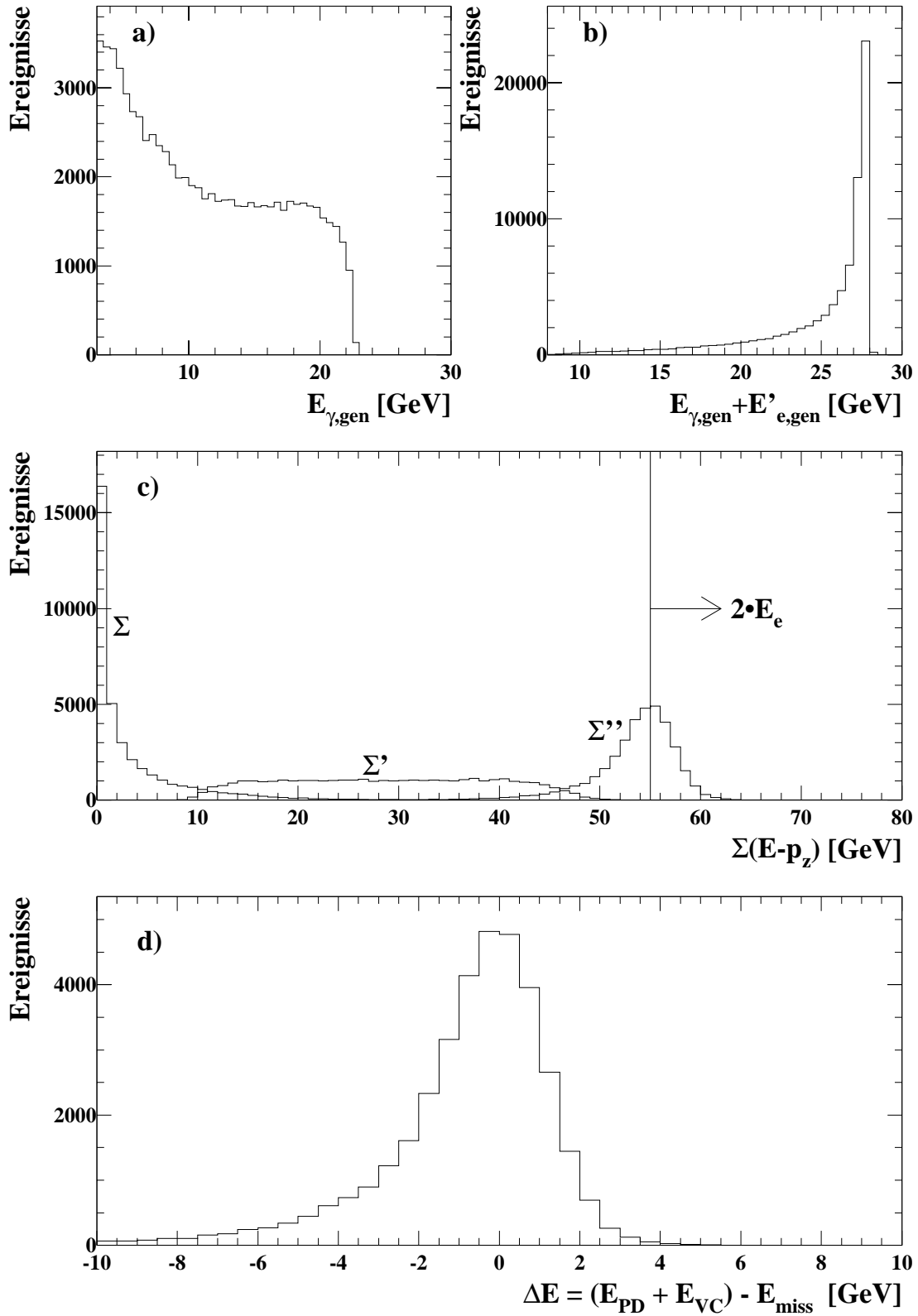
Abbildung 5.4: Verteilung der Größen E_\gamma , E_\gamma + E'_e , \Sigma , \Sigma' , \Sigma'' und \Delta E für simulierte tiefinelastische Ereignisse mit ISR, die im Akzeptanzbereich des BEMC liegen: 160^\circ < \theta_{e, \text{gen}} < 174^\circ .
