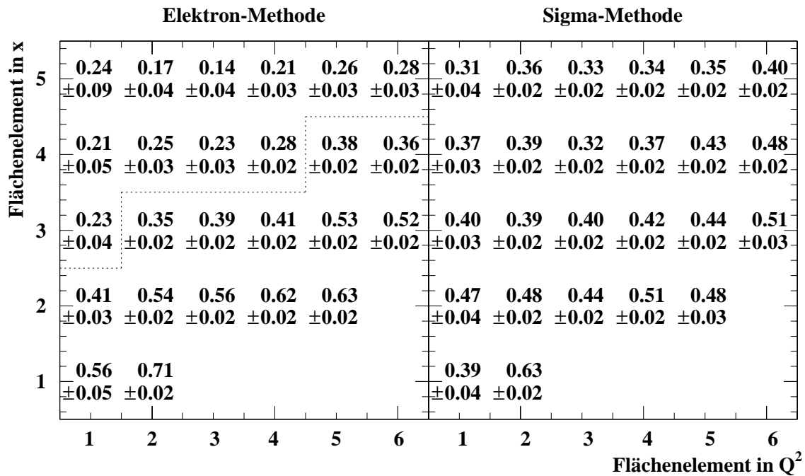
Abbildung 7.3: Aus der Simulation erhaltene Reinheit der Flächenelemente für die Elektron-Methode links und für die Sigma-Methode rechts. Die statistischen Fehler sind ebenfalls angegeben. Die Trennlinie zwischen Flächenelementen mit einer Reinheit oberhalb und unterhalb von 30% ist als gepunktete Linie eingezeichnet.
