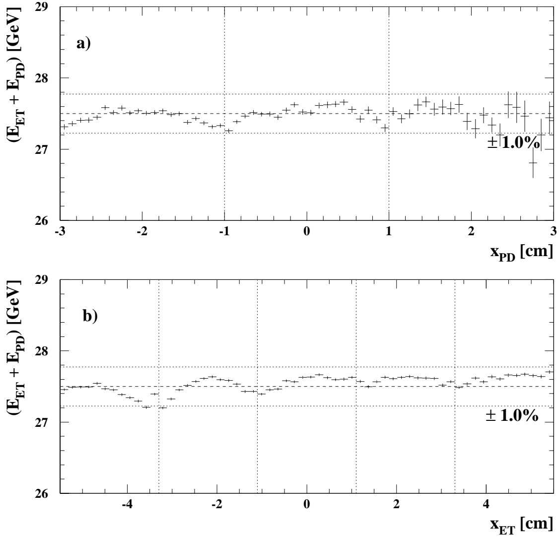
Abbildung 6.8: Überprüfung der Homogenität der Detektoren des Luminositätssystems. Es wurden Bremsstrahlungseignisse mit E_{VC} < 0,1 \text{ GeV} selektiert und die Energiesumme (E_{PD} + E_{ET}) als Funktion von x_{PD} in a) und als Funktion von x_{ET} in b) dargestellt. Die gepunkteten vertikalen Linien deuten die Grenzen zwischen den einzelnen Kristallen der Detektoren an. Die horizontalen Linien geben den erwarteten Wert von 27,5 \text{ GeV} und ein Fehlerband von \pm 1\% an.
