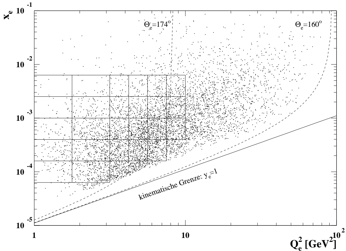
Abbildung 7.1: Einteilung der kinematischen Ebene in Flächenelemente, wie sie in der vorliegenden Arbeit verwendet wurde. Ebenfalls eingezeichnet ist die Verteilung der tiefinelastischen Ereignisse mit ISR. Der Akzeptanzbereich des BEMC für tiefinelastische Ereignisse ohne ISR liegt in dem Bereich 160^\circ < \theta < 174^\circ , der durch gestrichelte Linien angedeutet ist.
