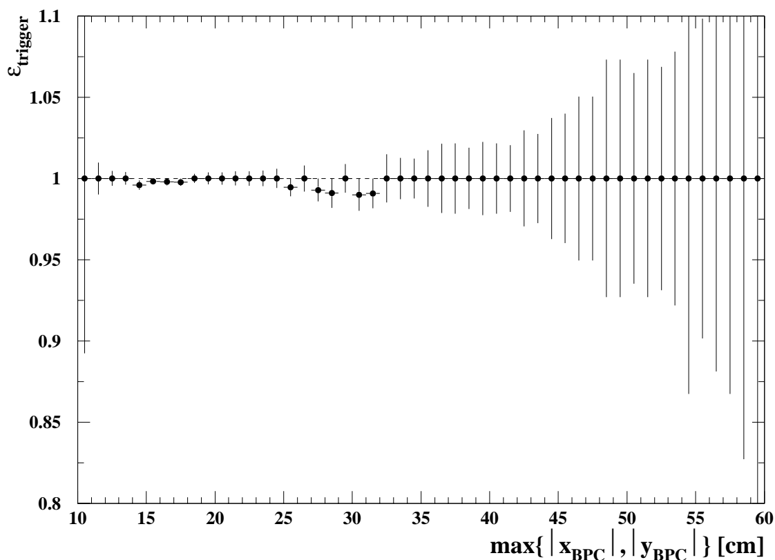
Abbildung 7.4: Überprüfung der Ortsabhängigkeit des Subtriggers S_0 für Runs, bei denen die inneren Dreiecksmodule des BEMC für das Triggersignal berücksichtigt wurden. Die Energie der ausgewählten Ereignisse ist größer als 11 GeV und liegt somit weit oberhalb der Energieschwelle des Triggers von 7,7 GeV.
