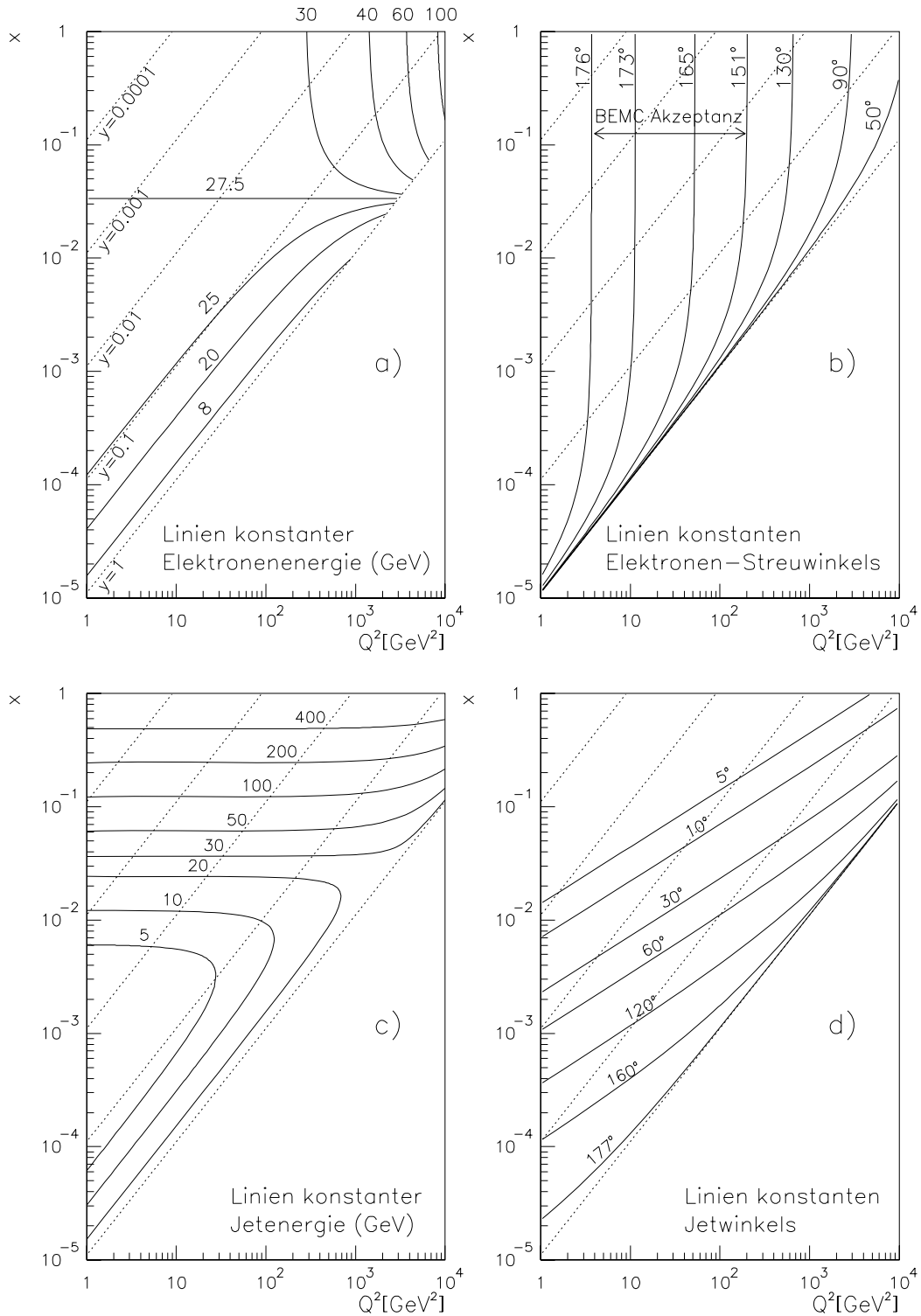
Abbildung 2.2: Zusammenhang direkt messbarer Größen mit den in diesem Abschnitt definierten lorentzinvarianten Größen x , y und Q^2 . Linien mit konstanten und jeweils gleichen Werten von y sind in allen Abbildungen als gestrichelte Linien eingezeichnet. In a) und b) sind Linien konstanter Energie und konstanten Streuwinkels des Elektrons abgebildet. In c) und d) sind Linien konstanter Jetenergie und konstanten Jetwinkels dargestellt.
