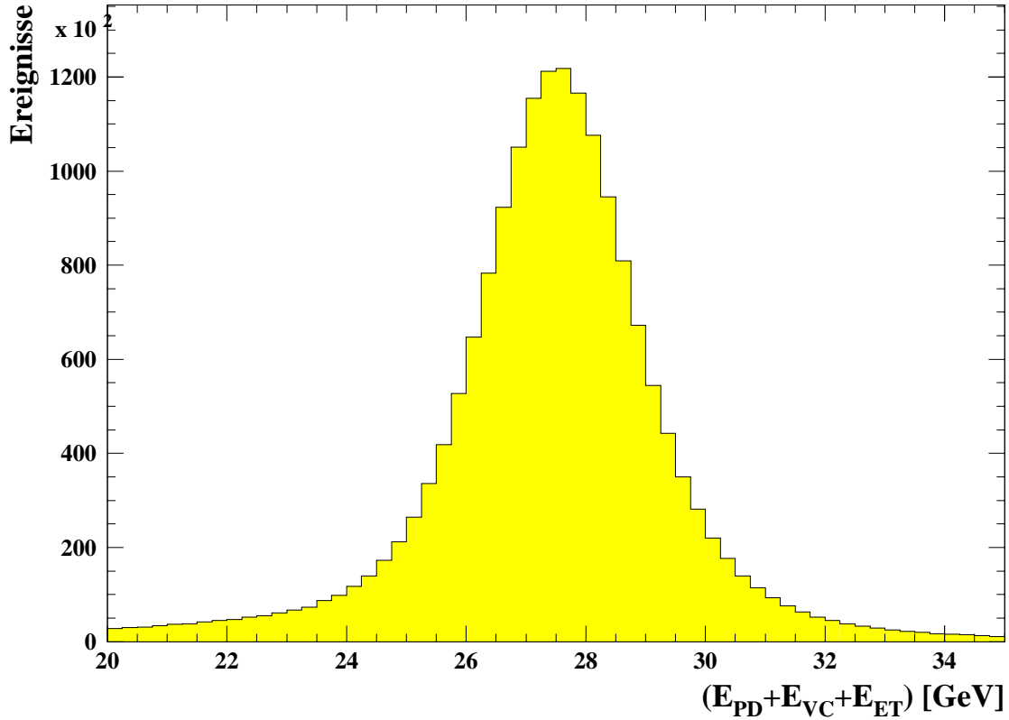
Abbildung 5.12: Summe der Energien ( E_{\text{PD}} + E_{\text{VC}} + E_{\text{ET}} ) im Photondetektor, im Veto­zähler und im Elektron­detektor für selektierte Bremsstrahlungseignisse.
