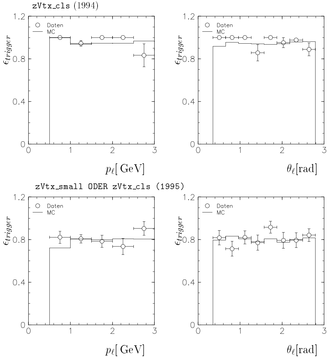
Abbildung 5.3: zVertex-Trigger: Triggerwahrscheinlichkeiten für das Triggererelement zVtx_cls für Zwei-Spur Kandidaten für die Datennahmeperiode 1994 (oben) sowie für die logische Kombination der Triggererelemente zVtx_small ODER zVtx_cls für Zwei-Spur Kandidaten für die Datennahmeperiode 1995 (unten) verglichen mit der Monte-Carlo-Simulation als Funktion von Impuls und Polarwinkel der beiden Leptonen. Die Triggerwahrscheinlichkeit wurde in der Monte-Carlo-Simulation für das Jahr 1995 um 5% vermindert.
