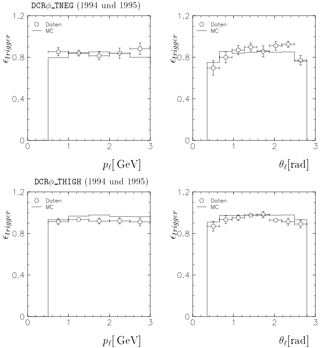
Abbildung 5.6: DCR \phi -Trigger: Triggerwahrscheinlichkeit für die Triggerelemente \text{DCR}\phi_{\text{TNEG}} (oben) und \text{DCR}\phi_{\text{THIGH}} (unten) in Abhängigkeit von Impuls und Polarwinkel des entsprechenden Zerfallsleptons analog zu Abbildung 5.5.
