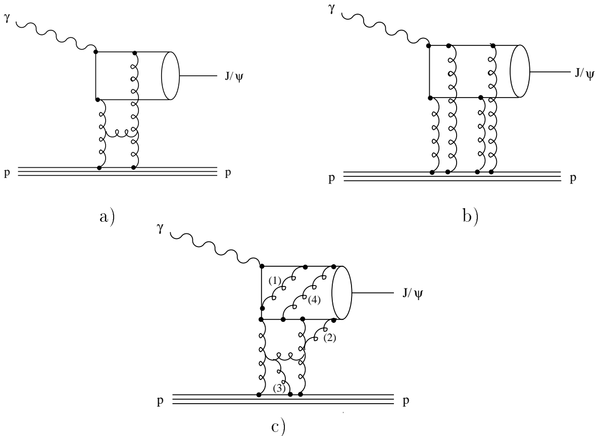
Abbildung 2.6: Korrekturen höherer Ordnung im Ryskin-Modell: a) Leiterdiagramm, b) Streuung und Absorption von c\bar{c} -Paaren und c) vier verschiedene Arten von Strahlungskorrekturen in nächstführender Ordnung, die mit (1) bis (4) bezeichnet sind.
