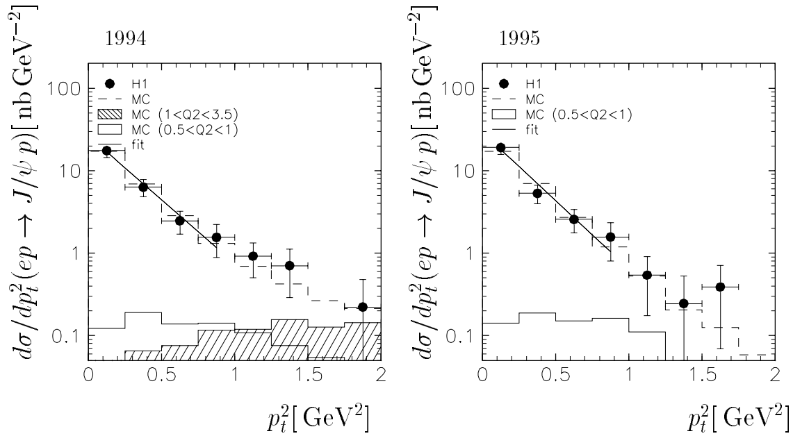
Abbildung 8.6: Elastische J/\psi -Produktion: Differentieller Wirkungsquerschnitt d\sigma/dp_t^2(ep \rightarrow J/\psi p) für elastische J/\psi -Produktion getrennt für die Datennahmeprioden 1994 und 1995. Dargestellt sind die H1-Messpunkte, wobei statistische und systematische Fehler quadratisch addiert wurden, die Log-Likelihood-Anpassung der Form \exp(-bp_t^2) sowie die Monte-Carlo-Vorhersage (DIFFVM) für Photoproduktion mit Q^2 < 3.5 \text{ GeV}^2 für die Datennahmepriode 1994 und Q^2 < 1 \text{ GeV}^2 für die Datennahmepriode 1995 sowie für eingeschränkte Bereiche von hohen Q^2 . Für diese Bereiche wurde 0.5 \text{ GeV}^2 \leq Q^2 \leq 1 \text{ GeV}^2 (offenes Histogramm) und 1.0 \text{ GeV}^2 \leq Q^2 \leq 3.5 \text{ GeV}^2 (schraffiertes Histogramm) gewählt.
