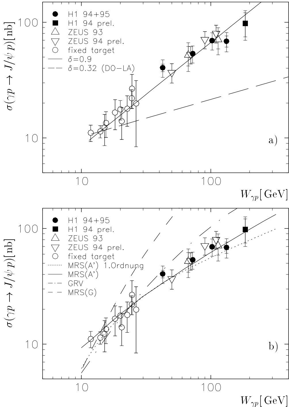
Abbildung 8.5: Totaler Wirkungsquerschnitt für elastische J/\psi -Produktion: H1-Messungen der Datennahmep perioden 1994 und 1995 (● diese Analyse) und der Datennahmep perioden 1994 (■ H1-Analyse in Rückwärtsrichtung bei W_{\gamma p} = 185 GeV) im Vergleich mit Messungen der ZEUS-Kollaboration (△▽) und verschiedener Niederenergieexperimente (○). Die inneren Fehlerbalken berücksichtigen die statistischen Fehler, die äußeren Fehlerbalken berücksichtigen statistischen und systematischen Fehler quadratisch addiert. Die Daten werden verglichen mit theoretischen Vorhersagen a) im Donnachie-Landshoff-Modell und b) im Ryskin-Modell mit verschiedenen Strukturfunktionen (MRS(A'), GRV, MRS(G)) sowie für Rechnungen erster Ordnung, wobei die Gluondichte MRS(A') Verwendung findet.
