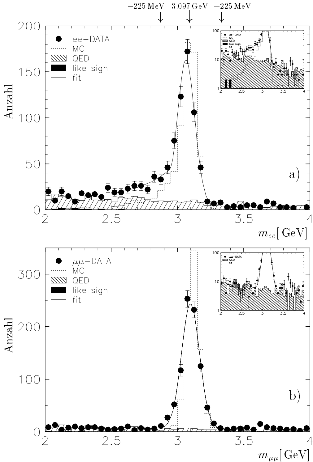
Abbildung 7.9: Zwei-Spur J/\psi -Kandidaten: Invariante Masse für a) Elektronenpaare und b) Myonpaare für die Datenmeperioden 1994 und 1995 kombiniert. Dargestellt sind neben den Daten die Vorhersage der Monte-Carlo-Simulation, der erwartete Untergrund an Ereignissen aus Photon-Photon-Wechselwirkungen (QED) und der Untergrund an gleichnamig geladenen Leptonpaaren (like-sign, nur bei e^+e^- sichtbar). An die Daten wurde eine Gaußfunktion zusammen mit einem Polynom zweiten Grades für den myonischen Zerfallskanal und einer exponentiell ansteigenden Funktion für den elektronischen Zerfallskanal angepaßt (fit). Rechts oben ist jeweils die Massenverteilung mit logarithmischer y-Achse dargestellt.
