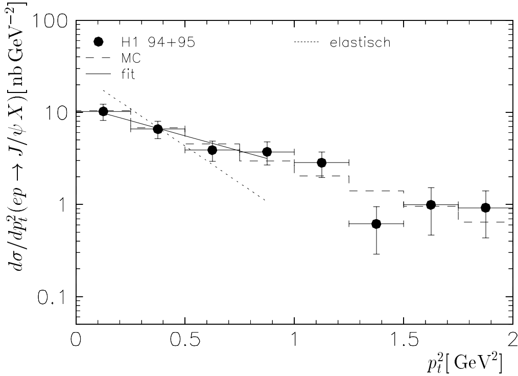
Abbildung 8.13: J/\psi -Produktion mit Proton-Dissoziation: Differentieller Wirkungsquerschnitt d\sigma/dp_t^2 für J/\psi -Produktion mit Proton-Dissoziation. Dargestellt sind die Meßpunkte dieser Analyse, die Log-Likelihood-Anpassung der Form \exp(-bp_t^2) sowie die Monte-Carlo-Vorhersage. Die Fehler beinhalten statistischen und systematischen Fehler quadratisch addiert. Zum Vergleich ist die Steigung des Wirkungsquerschnittes für elastische J/\psi -Produktion als gestrichelte Linie abgebildet.
