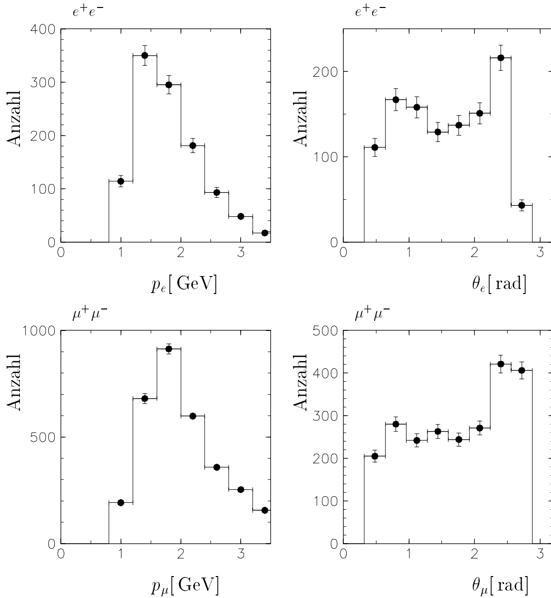
Abbildung 6.3: Impuls- und Polarwinkelverteilung der Zerfallsleptonen der Ein-Lepton J/\psi -Kandidaten für den elektronischen und myonischen Zerfallskanal. Diese Kandidaten werden für die Überprüfung der Nachweiswahrscheinlichkeiten verwendet.
