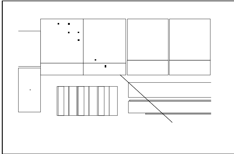
Abbildung 6.7: Identifikation von Myonen: Myonsignatur im LAr-Kalorimeter. Die rekonstruierte Driftkammerspur hat einen Impuls von 2.3 GeV, die Energiedeposition im LAr-Kalorimeter beträgt 1.6 GeV, es sprechen 4 verschiedene hadronische Lagen des LAr-Kalorimeters an.
