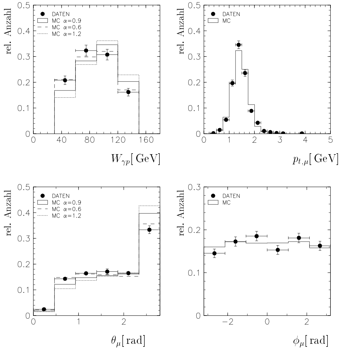
Abbildung 7.13: Zwei-Spur J/\psi -Kandidaten J/\psi \rightarrow \mu^+\mu^- : Vergleich zwischen den kombinierten Daten der Datennahmeperiode 1994 und 1995 und der Monte-Carlo-Simulation (DIFFVM) für die Zwei-Spur J/\psi -Selektion. Für die Verteilung der Schwerpunktsenergie W_{\gamma p} und des Polarwinkels \theta der Zerfallselektronen wurde zusätzlich zu \sigma \propto W_{\gamma p}^{0.9} eine Abhängigkeit des Wirkungsquerschnitts von der Schwerpunktsenergie der Form \sigma \propto W_{\gamma p}^{0.6} und \sigma \propto W_{\gamma p}^{1.2} verwendet.
