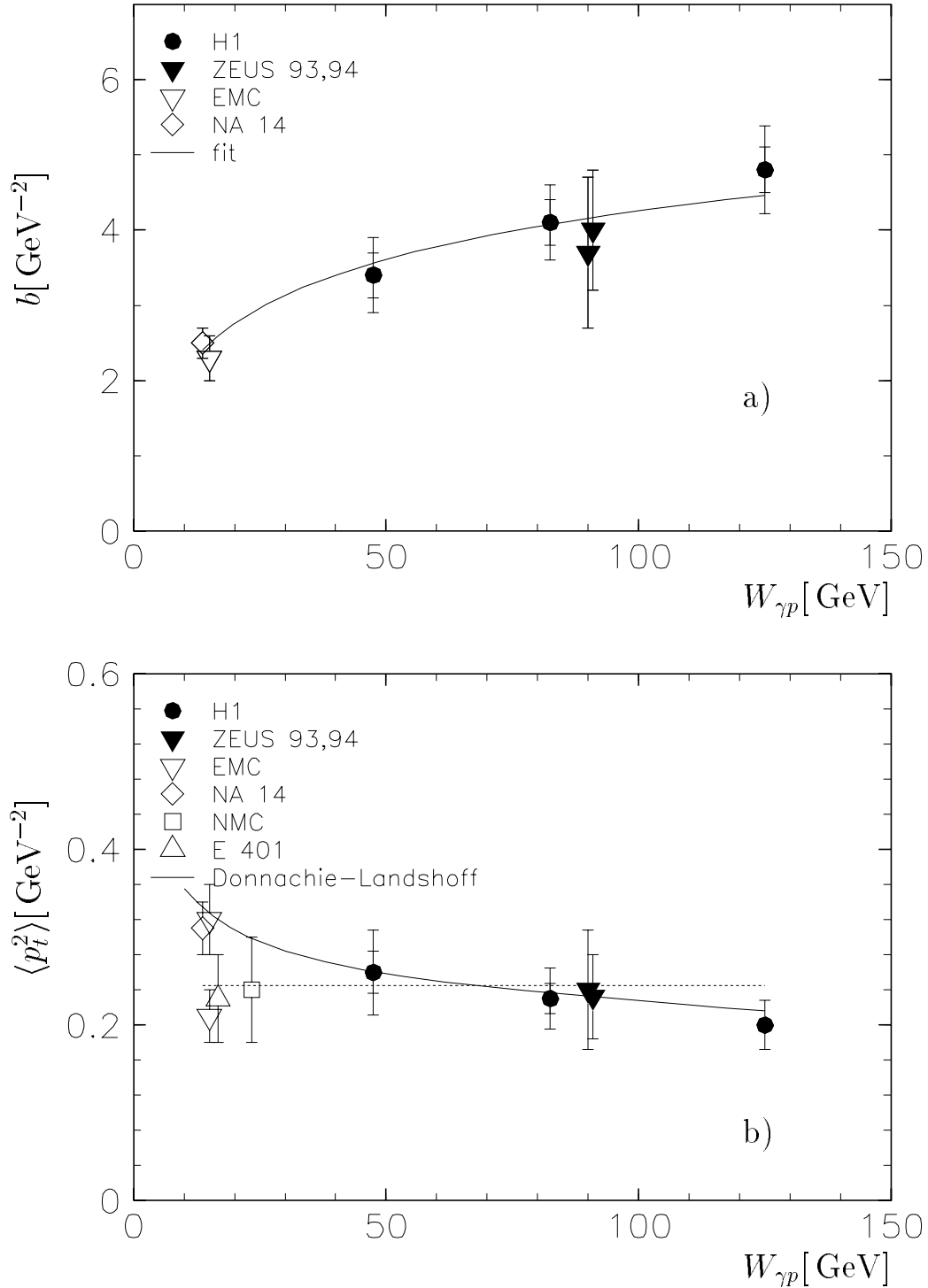
Abbildung 8.8: Elastische J/\psi -Produktion: a) Steigungsparameter b der p_t^2 -Verteilung für verschiedene Werte der Schwerpunktsenergie W_{\gamma p} dargestellt für diese Analyse (Datennahmeperioden 1994 und 1995 kombiniert) sowie für Messungen der ZEUS-Kollaboration und verschiedener Experimente bei niedrigeren Schwerpunktsenergien. An alle hier angegebenen experimentellen Werte wurde eine Funktion der Form \text{const} + 2\alpha' \ln W_{\gamma p}^2 mit \alpha' = (0.23 \pm 0.05) \text{ GeV}^{-2} angepasst. b) Mittleres p_t^2 im Bereich 0 \leq p_t^2 \leq 1 \text{ GeV}^2 für diese Analyse im Vergleich mit anderen Experimenten und der theoretischen Vorhersage des Donnachie-Landshoff-Modells sowie einer flachen Verteilung.
