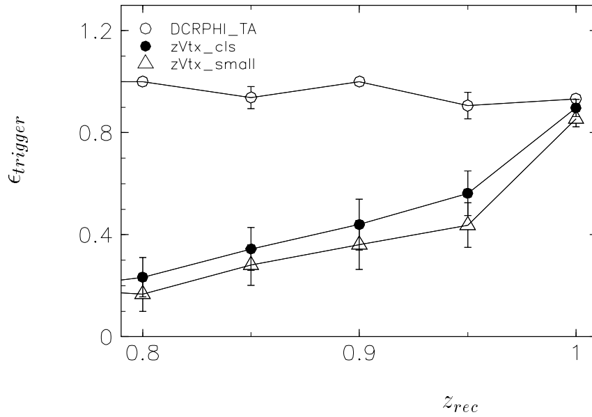
Abbildung 5.7: Spurkammertrigger: Triggerwahrscheinlichkeit der Triggerelemente DCR \phi _TA, zVtx_cls und zVtx_small als Funktion der aus den Daten rekonstruierten Elastizität z_{rec} , bestimmt mit Hilfe von J/\psi -Kandidaten der Datennahmeperiode 1994 mit invarianter Masse \pm 125 MeV um die nominelle J/\psi -Masse. Als unabhängige Trigger wurden BEMC- und Elektron-Tagger-Trigger verwendet.
