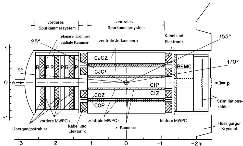
Abbildung 3.4: Das H1-Spurkammersystem
