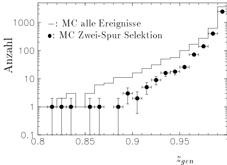
Abbildung 7.4: Simulation von J/\psi -Produktion mit Proton-Dissoziation (DIFFVM) : Elastizität z für alle generierten Ereignisse (Histogramm) und für alle Ereignisse mit 30 \text{ GeV} \leq W_{\gamma p} \leq 150 \text{ GeV} , die genau zwei rekonstruierte Spuren im Akzeptanzbereich ( 20^\circ \leq \theta \leq 160^\circ für den Polarwinkel der Zerfallsleptonen) haben.
