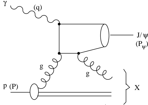
Abbildung 2.8: Inelastische Erzeugung von J/\psi -Mesonen durch Photon-Gluon-Fusion im Colour-Singlet-Modell. Dargestellt ist der Graph erster Ordnung.
