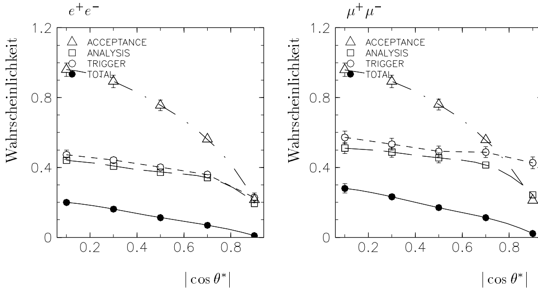
Abbildung 8.15: Quasi-elastische J/\psi -Produktion: Akzeptanz ( \triangle ), Selektionswahrscheinlichkeit ( \square ) und Triggerwahrscheinlichkeit ( \circ ) sowie das Produkt dieser drei Wahrscheinlichkeiten ( \bullet ) als Funktion von \cos \theta^* für J/\psi \rightarrow e^+e^- und J/\psi \rightarrow \mu^+\mu^- gemittelt über die Datennahmepereoden 1994 und 1995. Die Akzeptanz ist für beide Kanäle gleich. Die Fehlerbalken beinhalten quadratisch addiert systematische und statistische Fehler.
