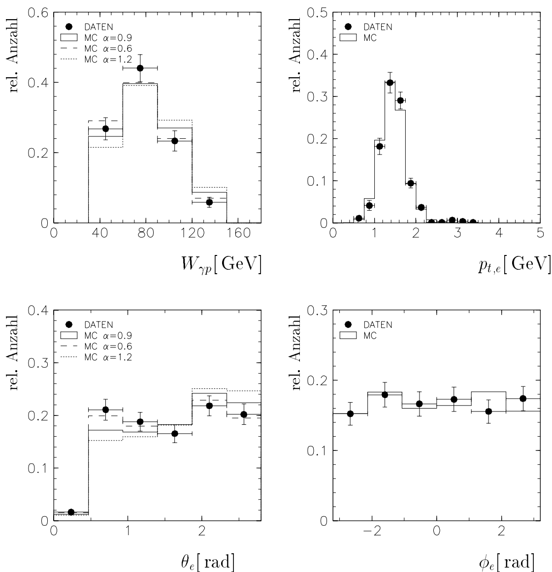
Abbildung 7.12: Zwei-Spur J/\psi -Kandidaten J/\psi \rightarrow e^+e^- : Vergleich zwischen den kombinierten Daten der Datennahmepériode 1994 und 1995 und der Monte-Carlo-Simulation (DIFFVM). Für die Verteilung der Schwerpunktsenergie W_{\gamma p} und des Polarwinkels \theta der Zerfallselektronen wurde zusätzlich zu \sigma \propto W_{\gamma p}^{0.9} eine Abhängigkeit des Wirkungsquerschnitts von der Schwerpunktsenergie der Form \sigma \propto W_{\gamma p}^{0.6} und \sigma \propto W_{\gamma p}^{1.2} verwendet.
