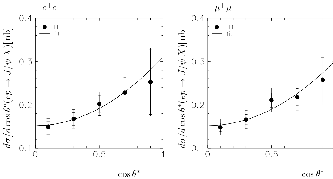
Abbildung 8.16: Quasi-elastische J/\psi -Produktion: Differentieller Wirkungsquerschnitt als Funktion von \cos \theta^* für den elektronischen und myonischen Zerfallskanal gemittelt für die Datennahmepereoden 1994 und 1995. Die inneren Fehlerbalken beinhalten die statistischen Fehler, die äußeren Fehlerbalken beinhalten statistischen und systematischen Fehler quadratisch addiert.
