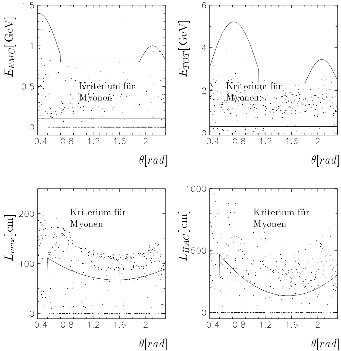
Abbildung 6.8: Identifikation von Myonen: Schnitte auf die Energiesummen E_{EMC} und E_{TOT} (untere und obere Grenze) und die Spurlängen L_{max} und L_{HAC} (nur untere Grenze) für die Identifikation von Myonen des Datensatzes von Ein-Myon J/\psi -Kandidaten. Eingezeichnet sind die Schnitte für Impulse p = 1 \text{ GeV} in Abhängigkeit des Polarwinkels. Die Schnitte wurden mit Hilfe einzelner simulierter Myonen eingestellt [84]. Die Schnitte sind dabei nicht scharf, sondern als fuzzy-Schnitte gemäß Abschnitt 6.4 zu verstehen.
