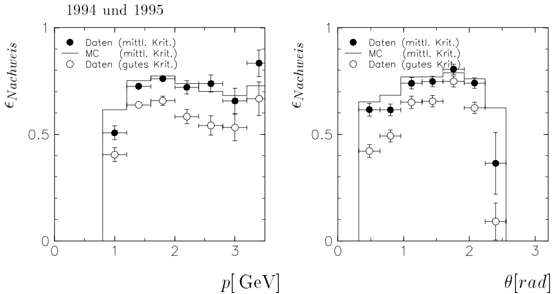
Abbildung 6.9: Identifikation von Myonen: Identifikationswahrscheinlichkeit für Myonen im LAr-Kalorimeter als Funktion von Impuls und Polarwinkel für Ein-Myon J/\psi -Kandidaten der Datennahmeperioden 1994 und 1995 (● mittleres Kriterium und ○ gutes Kriterium) im Vergleich mit der Detektorsimulation (– mittleres Kriterium). Die Identifikationswahrscheinlichkeit wurde in der Simulation um 15% vermindert.
