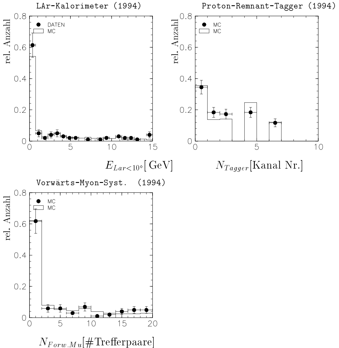
Abbildung 7.16: Zwei-Spur J/\psi -Kandidaten: Überprüfung der Signale in den Vorwärtsdetektoren für Daten (1994) und die Monte-Carlo-Simulation (DIFFVM). Das Verhalten des LAr-Kalorimeters und des Proton-Remnant-Taggers werden mit einem Datensatz mit Signal im Vorwärtsmyonsystem überprüft, das Verhalten des Vorwärtsmyonsystems mit einem Datensatz mit Signal im Proton-Remnant-Tagger. Für den Proton-Remnant-Tagger bedeutet ein Eintrag bei Null, daß keiner der Kanäle angesprochen hat. Für alle drei Detektoren wird das erste Bin für den elastischen J/\psi -Datensatz ausgewählt.
