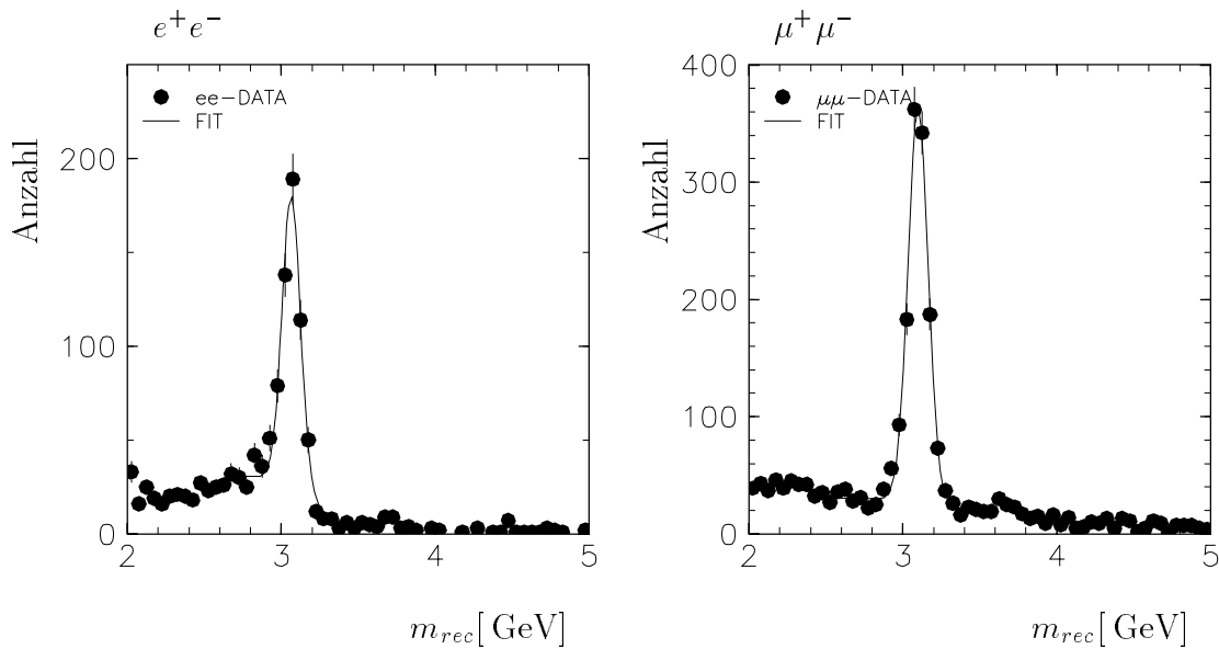
Abbildung 7.7: Zwei-Lepton J/\psi -Kandidaten: Invariante Masse für Elektronen- und Myonpaare der Datennahmeperioden 1994 und 1995 mit einem Schnitt auf die Elastizität z > 0.3 . Man erhält 678 J/\psi -Kandidaten im elektronischen Zerfallskanal und 1372 Kandidaten im myonischen Zerfallskanal in einem Massenfenster \pm 225 MeV um die nominelle J/\psi -Masse. Die Kurven stellen die Anpassung einer Gaußfunktion dar.
