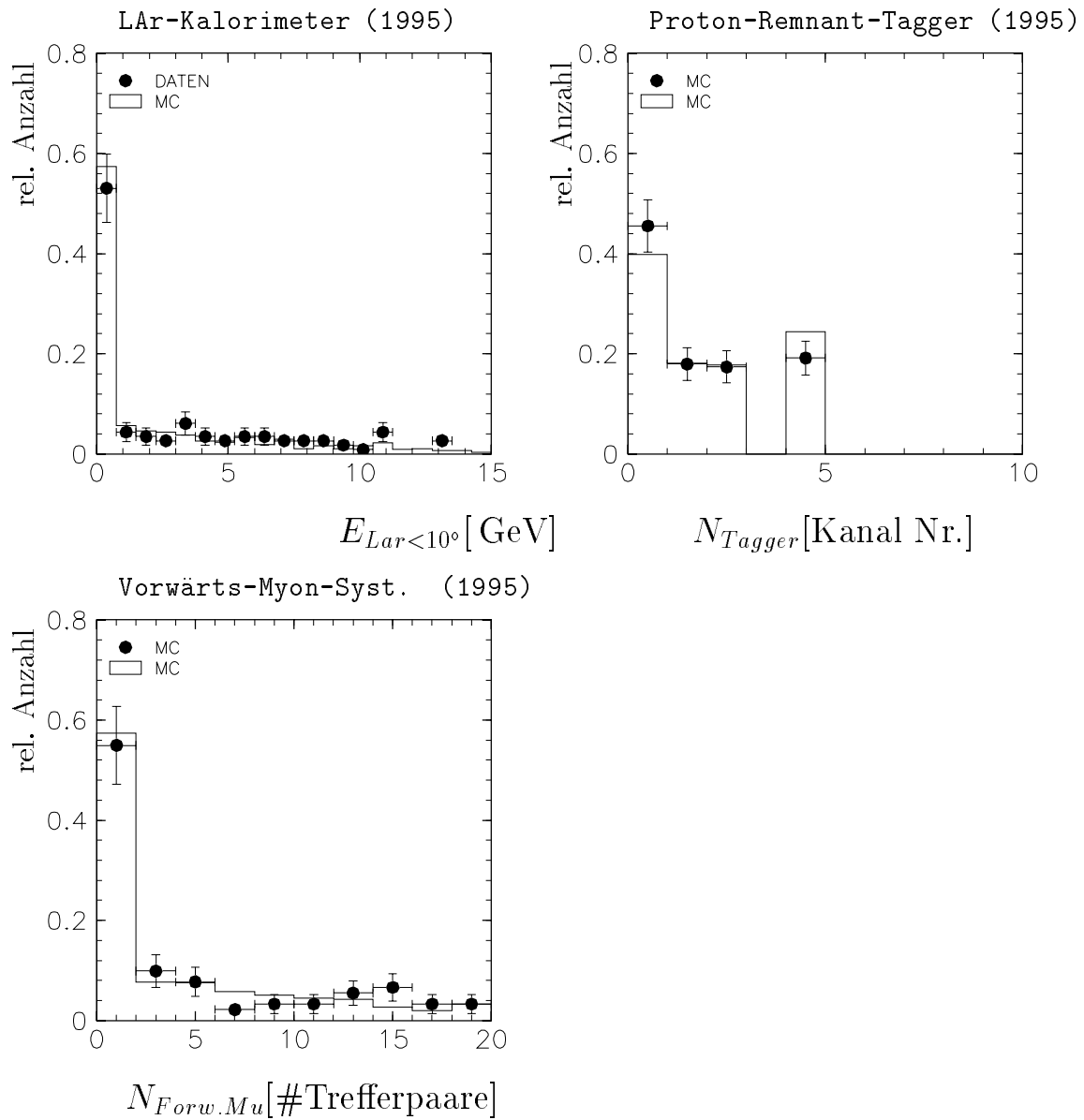
Abbildung 7.17: Zwei-Spur J/\psi -Kandidaten: Überprüfung der Signale in den Vorwärtsdetektoren für Daten (1995) und die Monte-Carlo-Simulation (DIFFVM) gemäß Abbildung 7.16.
