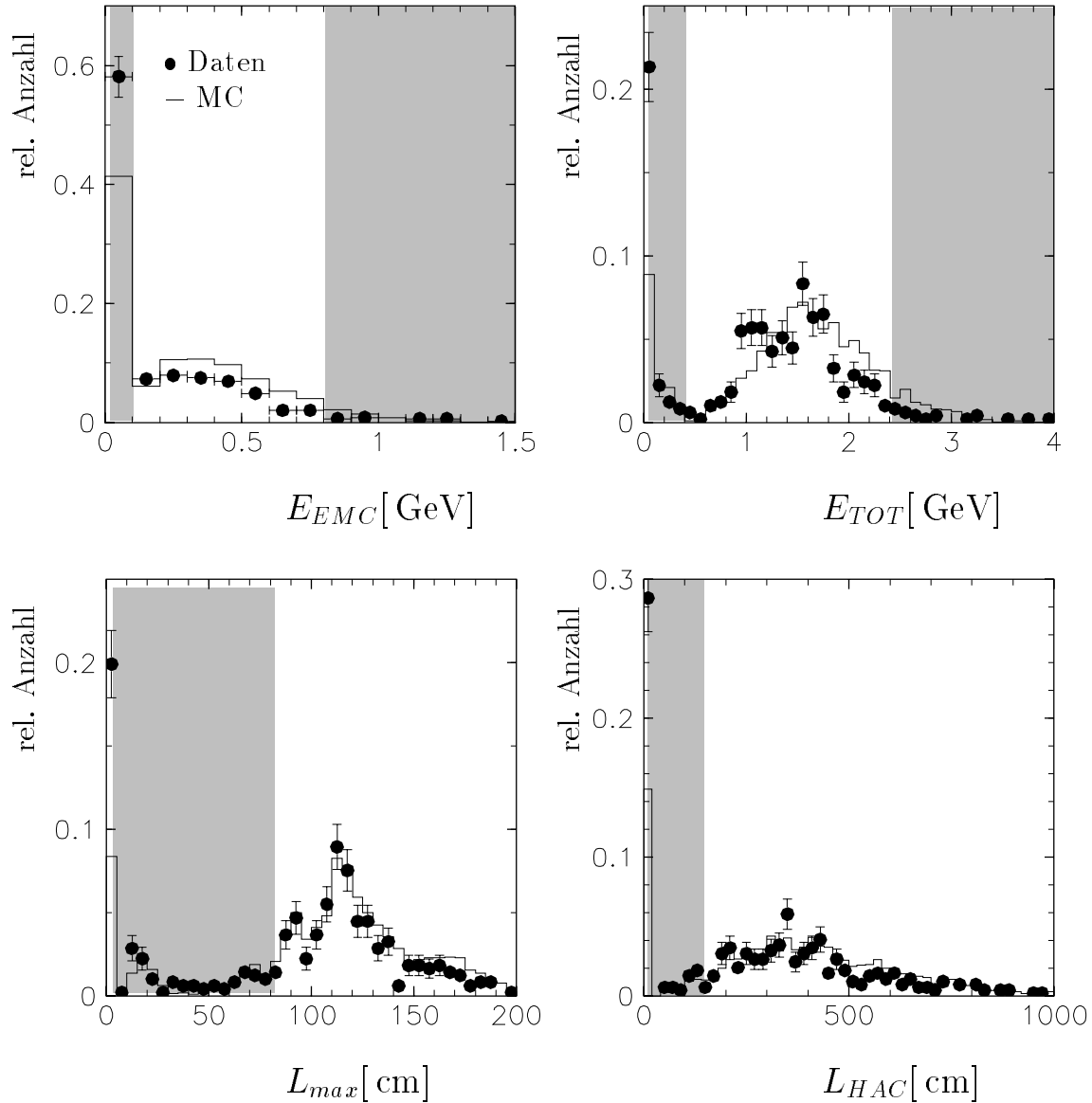
Abbildung 6.10: Identifikation von Myonen: Vergleich der Energiesummen und Spurlängen in Daten (Ein-Myon J/\psi -Kandidaten der Datennahmepériode 1994) und Monte-Carlo-Simulation für die Erkennung von Myonen. Die Bereiche, die für die Erkennung von Myonen im Zentralbereich des H1-Detektors ausgeschlossen werden, sind grau schraffiert. Es werden für die Darstellung die Mittelwerte der Schnitte verwendet. Die Schnitte sind dabei nicht scharf, sondern als fuzzy-Schnitte gemäß Abschnitt 6.4 zu verstehen.
