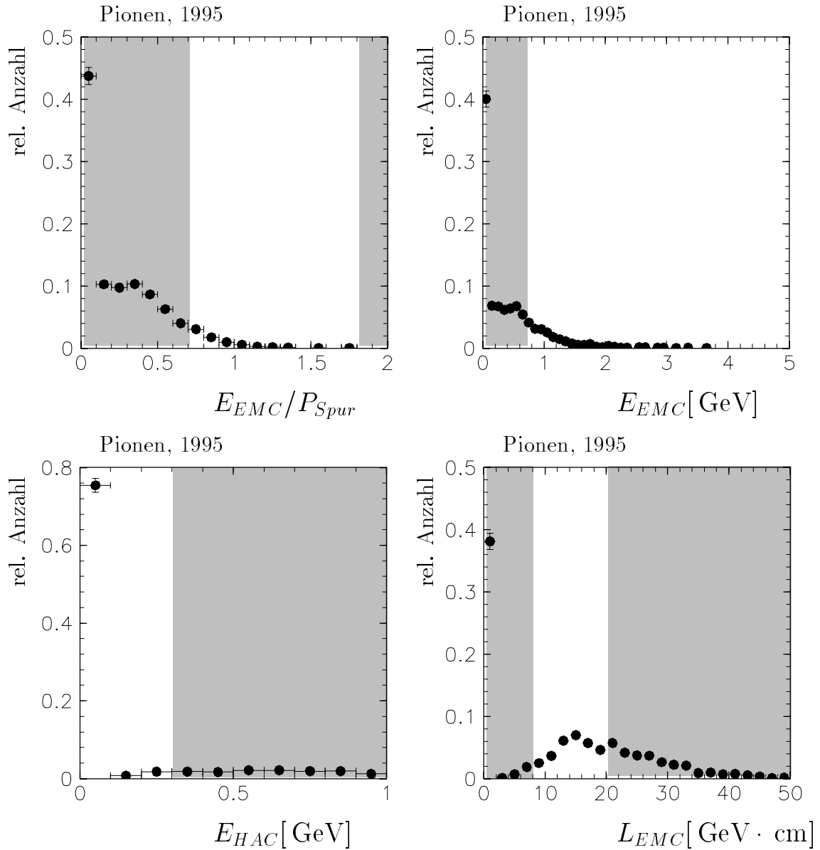
Abbildung 6.12: Fehlidentifikation von Pionen als Elektronen: Schnittgrößen analog Abbildung 6.5 für Pionen aus dem Zerfall von \rho -Mesonen der Datennahmeperiode 1995. Die Schnitte auf die verschiedenen Größen sind durch Schraffur gekennzeichnet.
