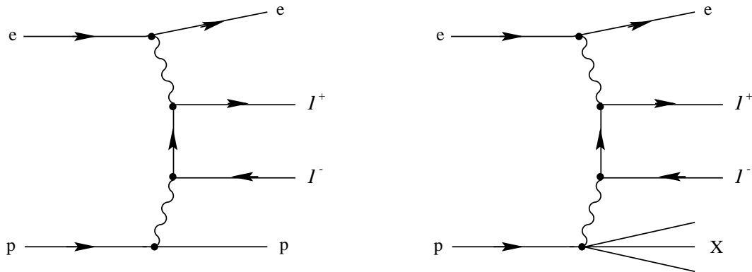
Abbildung 7.10: Elastische und inelastische Lepton Paar Erzeugung durch Photon-Photon-Wechselwirkung
