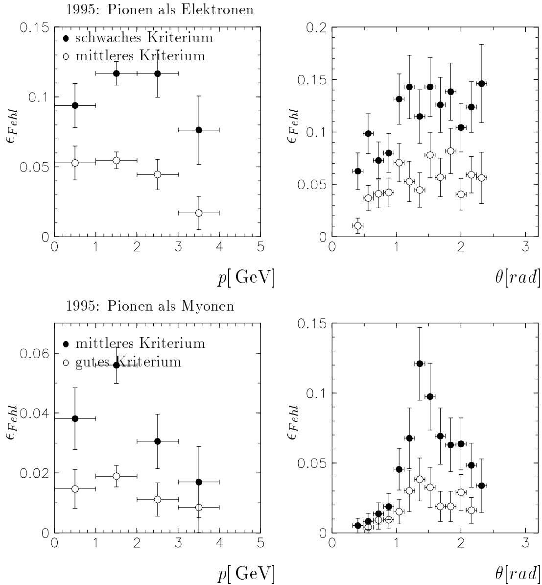
Abbildung 6.13: Fehlidentifikation von Pionen: Fehlidentifikationswahrscheinlichkeit von Pionen aus dem Zerfall von \rho -Mesonen (1995) für die schwache (●) sowie die mittlere (○) Elektron-Qualität (oben) bzw. für die mittlere (●) sowie die gute (○) Myon-Qualität (unten) als Funktion von Impuls und Polarwinkel.
