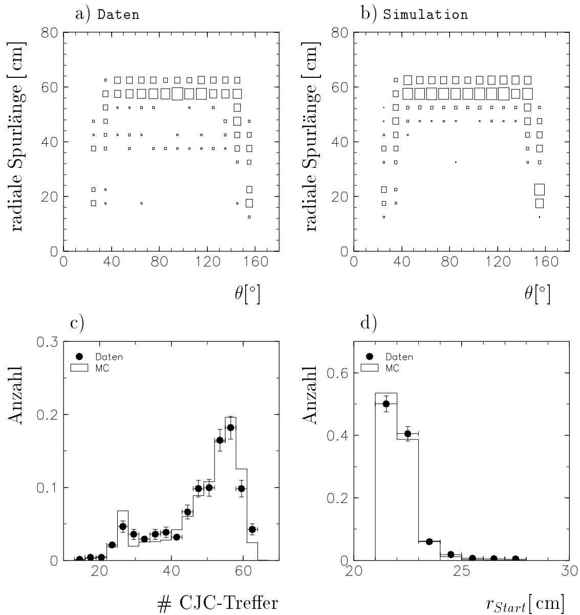
Abbildung 6.1: Rekonstruktion im zentralen Spurkammersystem: Vergleich wichtiger Spurparameter in Daten der Datennahmepereoden 1994 und 1995 ( J/\psi -Kandidaten) und der Monte-Carlo-Simulation: radiale Spurlänge als Funktion des Polarwinkels in Daten (a) und der Monte-Carlo-Simulation (b) sowie die Verteilung der Anzahl der Treffer (c), die zu einer rekonstruierten Spur in der CJC gehören, und der Radius r_{Start} (d), bei dem die rekonstruierte Spur in der zentralen Driftkammer beginnt.
