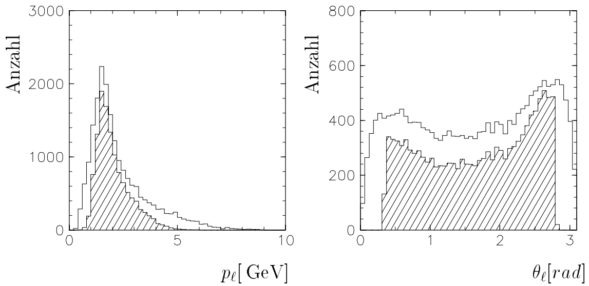
Abbildung 4.2: DIFFVM Monte-Carlo-Simulation: Impuls und Polarwinkelverteilung der Zerfallsleptonen im Bereich 30 \text{ GeV} \leq W_{\gamma p} \leq 150 \text{ GeV} (offenes Histogramm) und zusätzlich im Akzeptanzbereich 20^\circ \leq \theta \leq 160^\circ (schraffiertes Histogramm).
