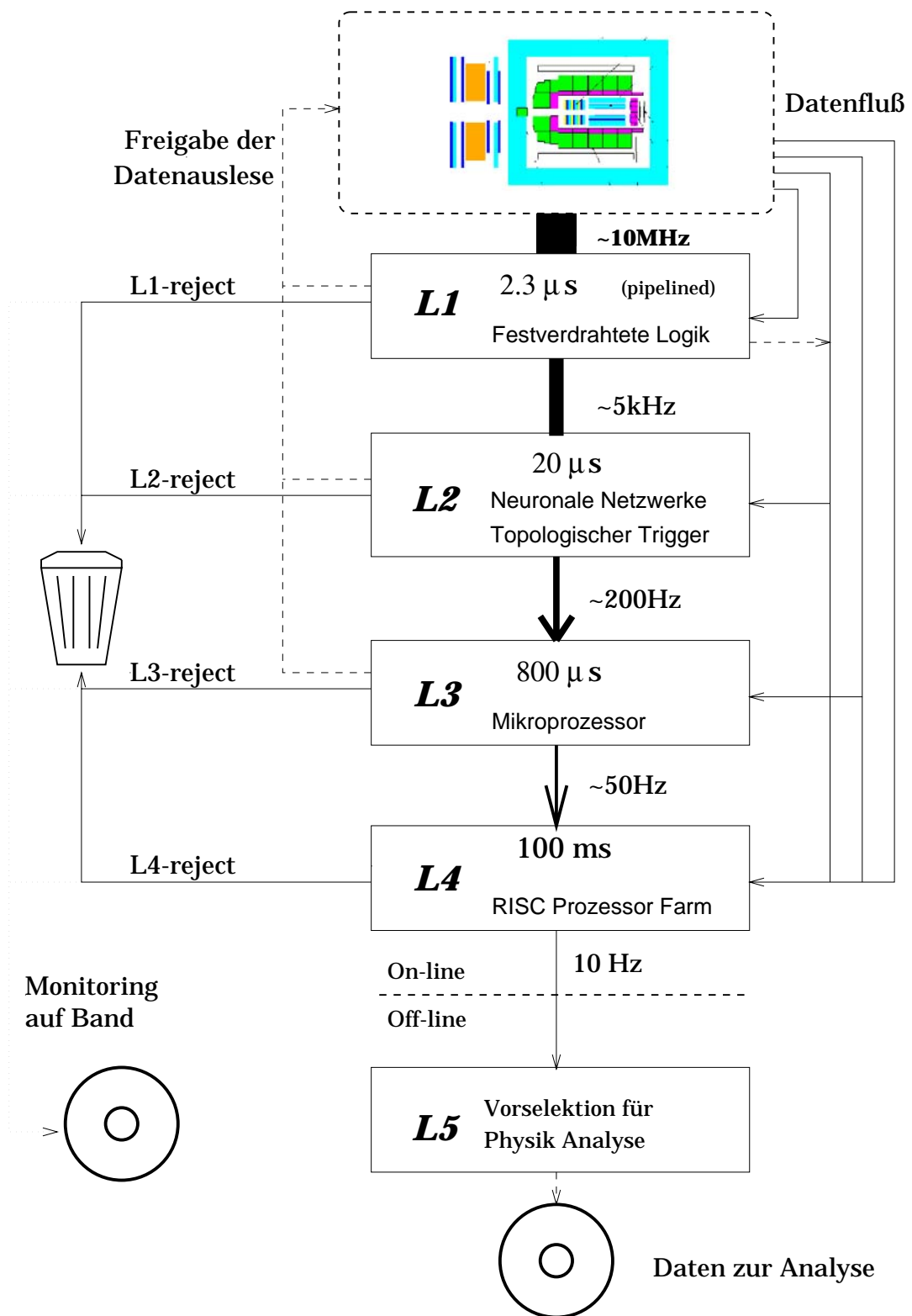
Abbildung 4.1: Schematischer Aufbau des H1-Triggersystems.
