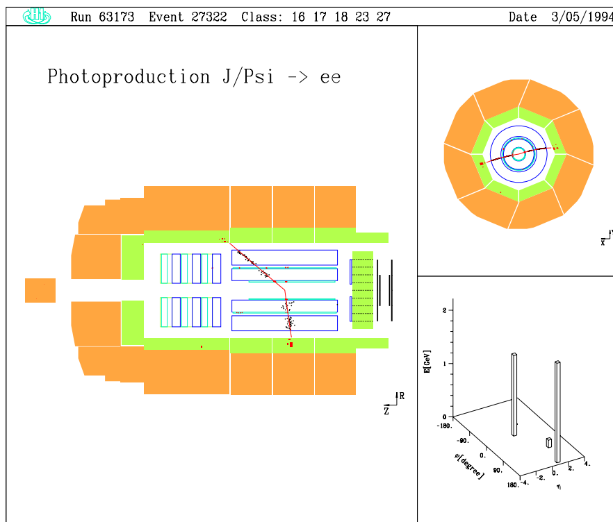
Abbildung 3.4: Ein J/\psi zerfällt in ein e^+e^- Paar.
