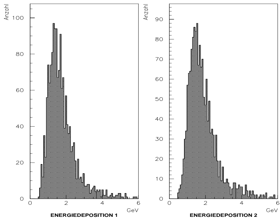
Abbildung 6.1: J/\psi invariante Masse (oben) und Energiedepositionen in dem Flüssig-Argon-Kalorimeter der beiden Zerfallselektronen (unten).
