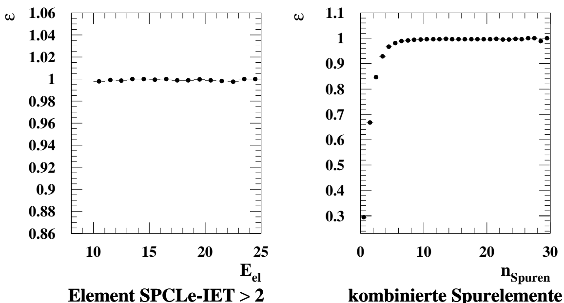
Abbildung 4.3: Trigger-Effizienzen des Physik-Triggers, aufgespalten in das Triggerelement SPCLe\_IET und die kombinierten Spurbedingungen für alle Daten der Analyse. Die Berechnung der Effizienz und die Erläuterung der Elemente befindet sich im Text.
