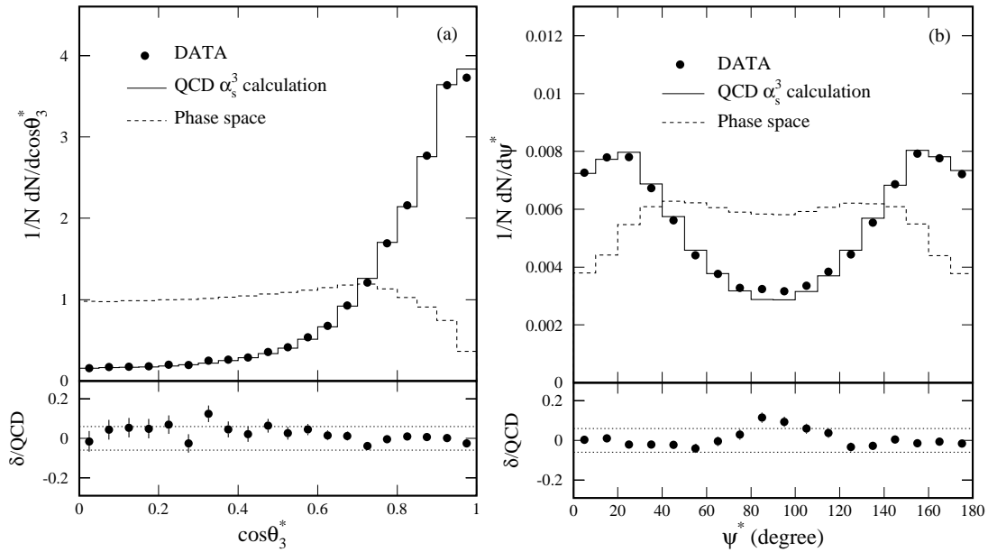
Abbildung 6.13: Daten der p\bar{p} -Streuung bei D0 gemessen. Für die Analyse [D0 96] wurde gefordert: M_{3jet} > 200 GeV, -3 < \eta < 3 , Transversalenergie der Jets (1,2,3) größer (60,20,20) GeV und sonst keine weiteren Schnitte auf das 3-Jet-System.
