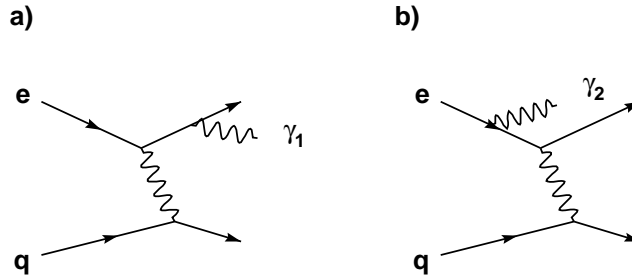
Abbildung 2.4: Berücksichtigung der radiativen Korrekturen zur e - p -Streuung: das Elektron kann vor oder nach der Streuung am Quark ein Photon aussenden, wie in b) bzw. a) dargestellt ist. Solche Ereignisse werden vom Monte Carlo-Generator DJANGO erzeugt und zur Korrektur der Daten auf radiative Effekte verwendet
