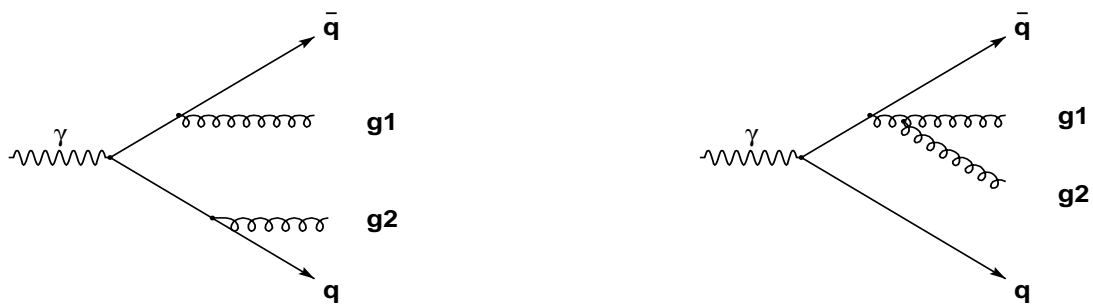
Abbildung 2.2: Feynmangraphen zur Dipolemission in ARIADNE: Erzeugung von q\bar{q}gg im Endzustand
