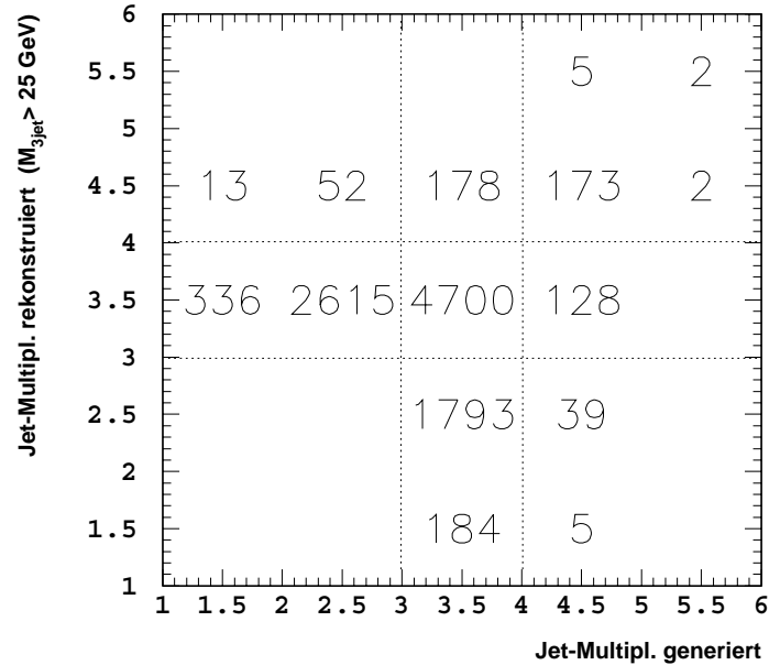
Abbildung 5.13: Migrationen der Jetmultiplizitäten für 3-Jet-Ereignisse mit einem Massenschnitt von M_{3jet} > 25 GeV und den Standardschnitten der Jetselektion aus der Vorhersage von RAPGAP. Die Zahlen sind absolute Ereignisanzahlen. Daraus kann man eine Reinheit von 69 % und eine Effizienz von 60 % für die Identifikation von 3 Jets bestimmen.
