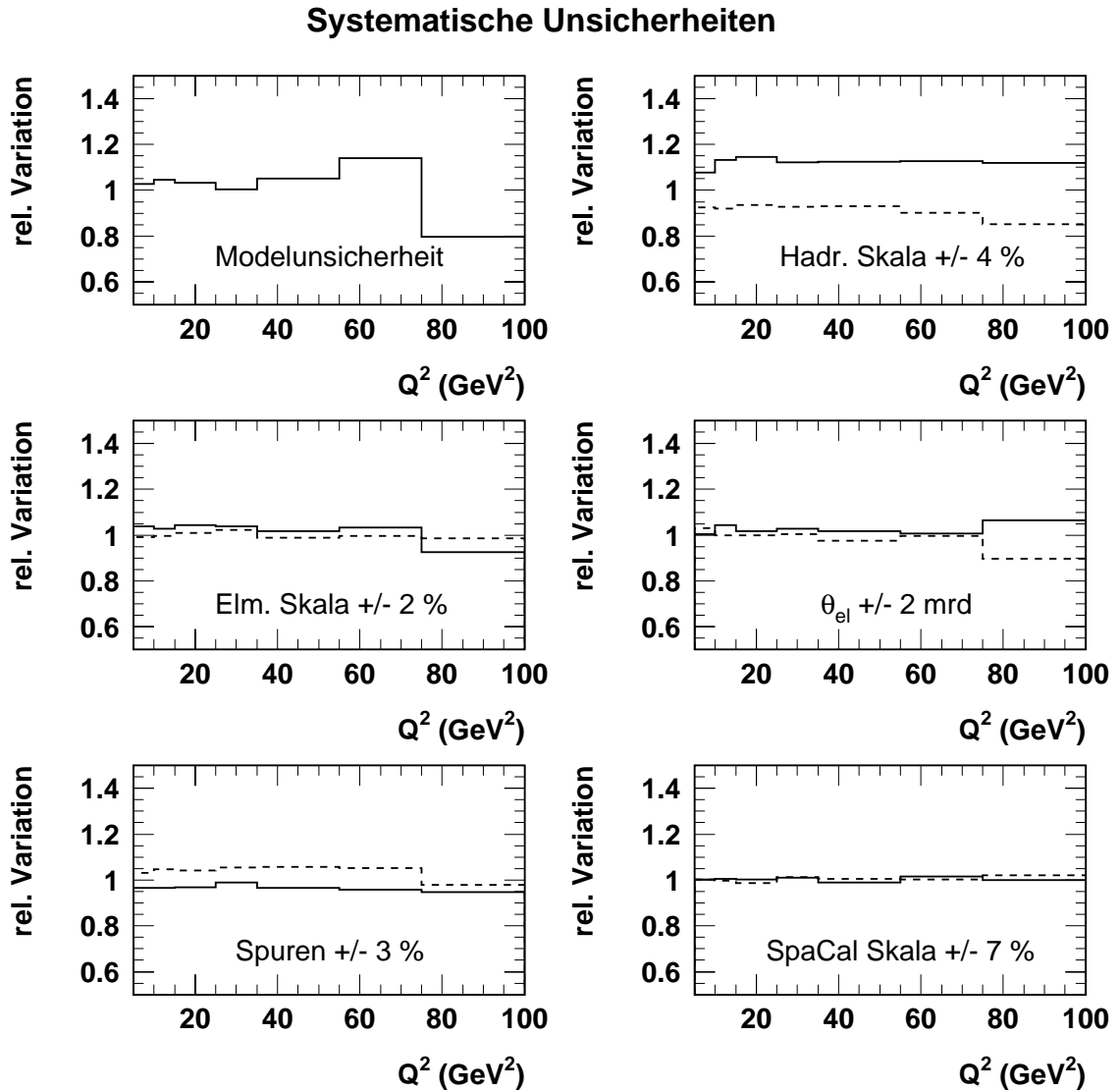
Abbildung 5.22: Systematische Unsicherheiten der Q^2 -Verteilung. Gezeigt ist die relative Variation der Daten, für verschiedene systematische Fehlerquellen, s. Text. Bis auf die Kurve der Modellunsicherheit oben links bedeutet die durchgezogene (gestrichelte) Linie immer die Variation um den aufgeführten positiven (negativen) Wert in Prozent.
