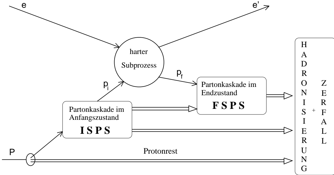
Abbildung 2.1: Schematische Darstellung der Simulation tiefunelastischer Ereignisse durch RAPGAP. Das Ereignis ist aufgeteilt in die Berechnung des Matrix-Elementes am Photonvertex, dem harten Subprozeß und dem Partonschauer, der im Anfangs- und Endzustand auftreten kann. Anschließend gehen alle Partonen in die Phase der Hadronisierung über.
