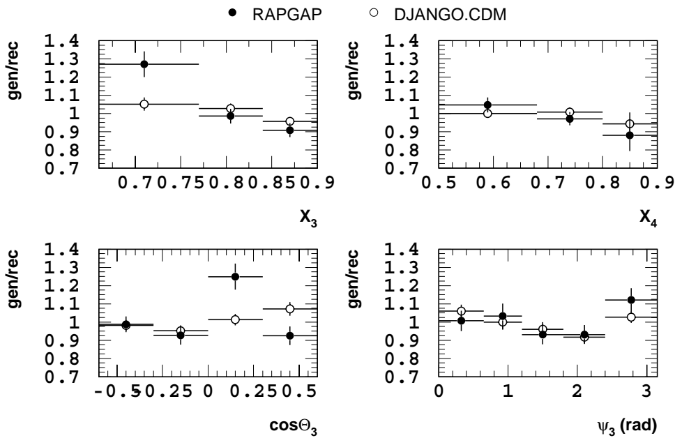
Abbildung 5.20: Dargestellt sind die Korrekturfaktoren nach Gl. 5.19 der Variablen des 3-Jet-Schwerpunktsystems, berechnet mit Hilfe von RAPGAP (geschlossenen Punkte) und DJANGO.CDM (offene Punkte). Man beachte, daß die y-Achse erst bei 0.7 beginnt.
