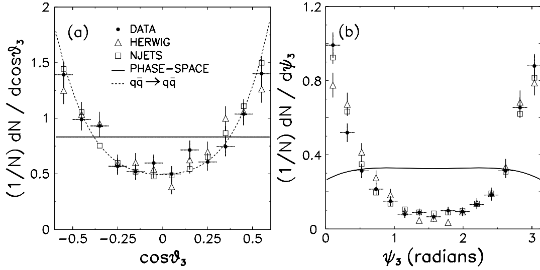
Abbildung 6.12: Daten der p\bar{p} -Streuung vom CDF-Experiment aus der Analyse [CDF96]. Es wurde gefordert M_{3jet} > 600 GeV, E_{T,jet} > 20 GeV, \sum E_{T,jets} > 420 GeV, -4.2 < \eta < 4.2 und X_3 < 0.9 , |\cos \Theta_3| < 0.6 .
