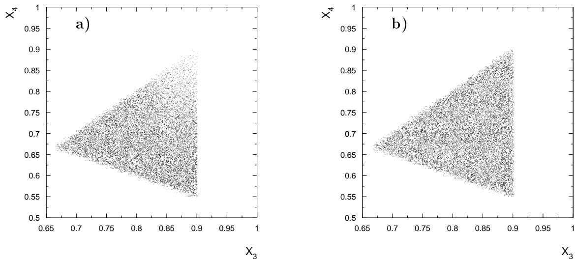
Abbildung 5.6: Dargestellt ist die Phasenraumdichte in der X_3 - X_4 -Ebene für verschiedene Schnitte. a) zeigt die Verteilung mit allen Anforderungen an die Energie und die Lage der Jets nach Gl. 5.1, 5.2 im Meßbereich von X_3 und X_4 . Eine gleichmäßige Phasenraumdichte in allen Ecken, s. Abb. b), erreicht man durch eine Lockerung des Schnittes auf E_{T, Breit} > 2 GeV. Denselben Effekt hat eine Erhöhung des Massenschnittes auf M_{3\text{jet}} > 50 GeV.
