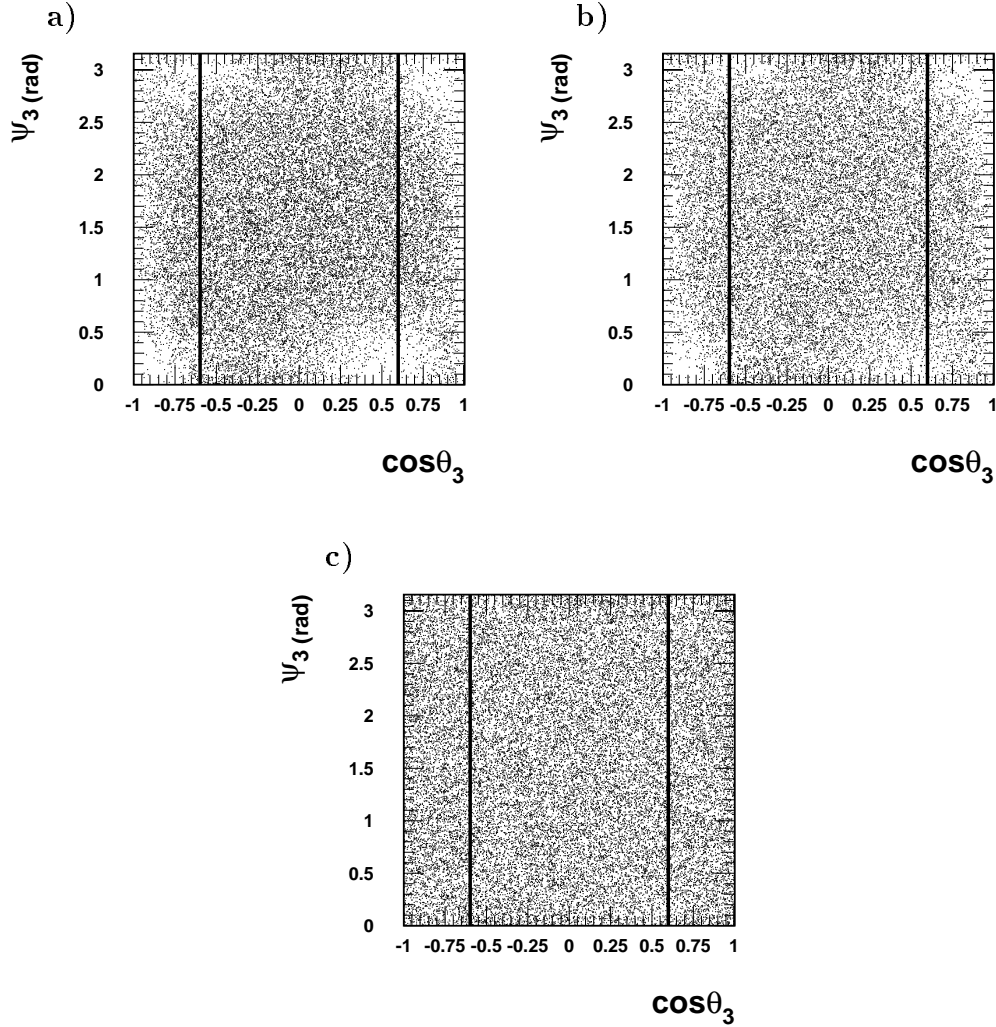
Abbildung 5.9: Dargestellt ist die Phasenraumdichte in der \cos\Theta_3 - \Psi_3 -Ebene. a) zeigt die Verteilung nach der Jetselektion. Der Bereich von \cos\Theta_3 , in dem gemessen wird, ist jeweils durch die senkrechten Linien gekennzeichnet. b) zeigt eine gleichmäßigere Dichteverteilung, die man erreicht, wenn man den Schnitt auf E_{T,Breit} > 2 GeV herabsetzt. Die vollständig gleichmäßig bevölkerte Ebene findet man, wenn man zusätzlich die Akzeptanz der Jets auf -4 < \eta_{lab} < 4 erweitert.
