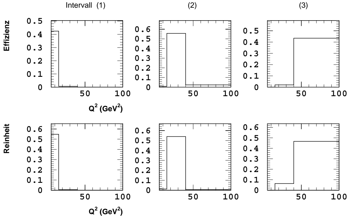
Abbildung 5.27: Effizienz und Reinheit der Q^2 -Verteilung von 4-Jet-Ereignissen in den gewählten Intervallen.
