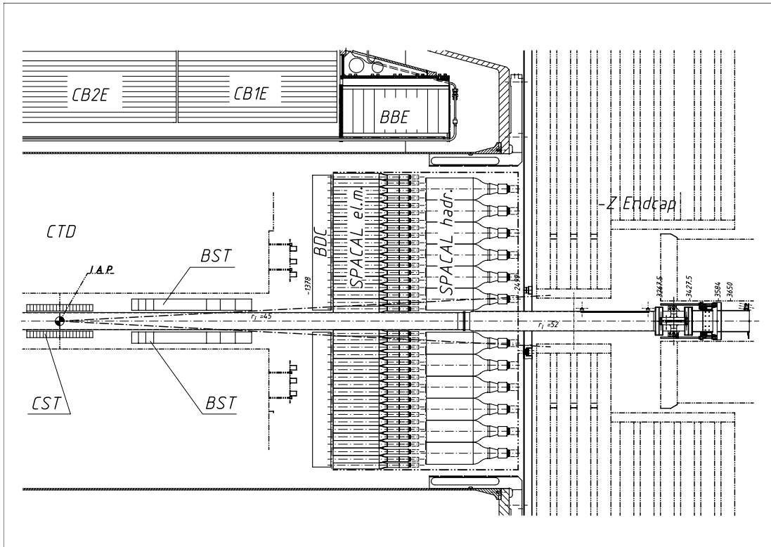
Abbildung 2.4: Seitenansicht des SpaCal im Rückwärtsbereich des H1-Detektors.
