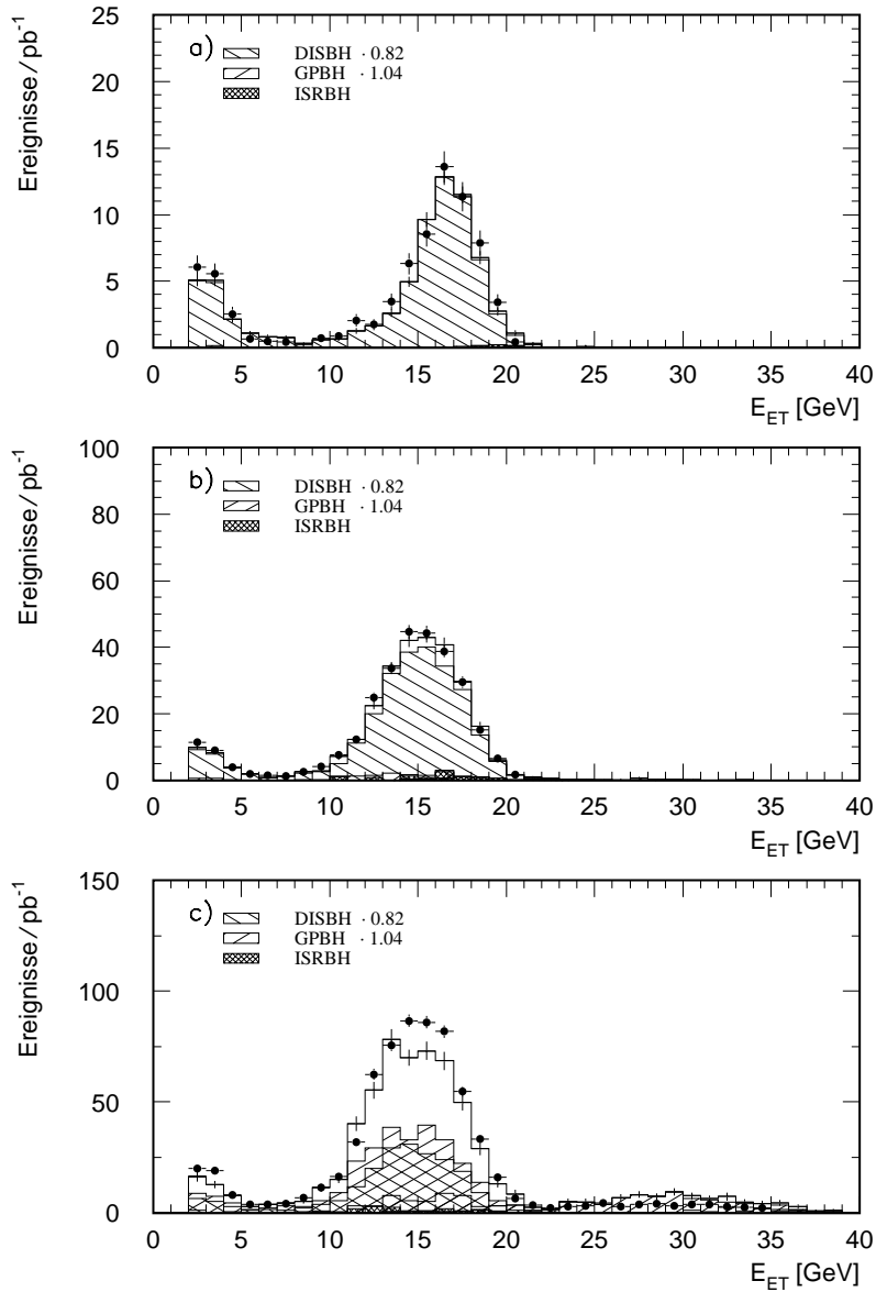
Abbildung 3.17: Energiespektrum im Elektronendetektor für Ereignisse aus Abbildung 3.16 in den drei Energiebereichen: a) 22.0 < E_e < 30.0 GeV, b) 12.0 < E_e < 22.0 GeV und c) 5.0 < E_e < 12.0 GeV. Die Punkte repräsentieren die Daten und die durchgezogene Linie ist die Summe der Untergrund-MC, wobei die Kreuze auf dieser Linie den statistischen Fehler des MC anzeigen. Zu sehen sind außerdem der DISBH-, GPBH- und ISRBH-Untergrund (schraffierte Histogramme). Die gezeigten Verteilungen sind absolut normiert, wobei die DISBH- und GPBH-Verteilung auf ihre systematische Abweichung von den Daten korrigiert worden sind (siehe Text).
