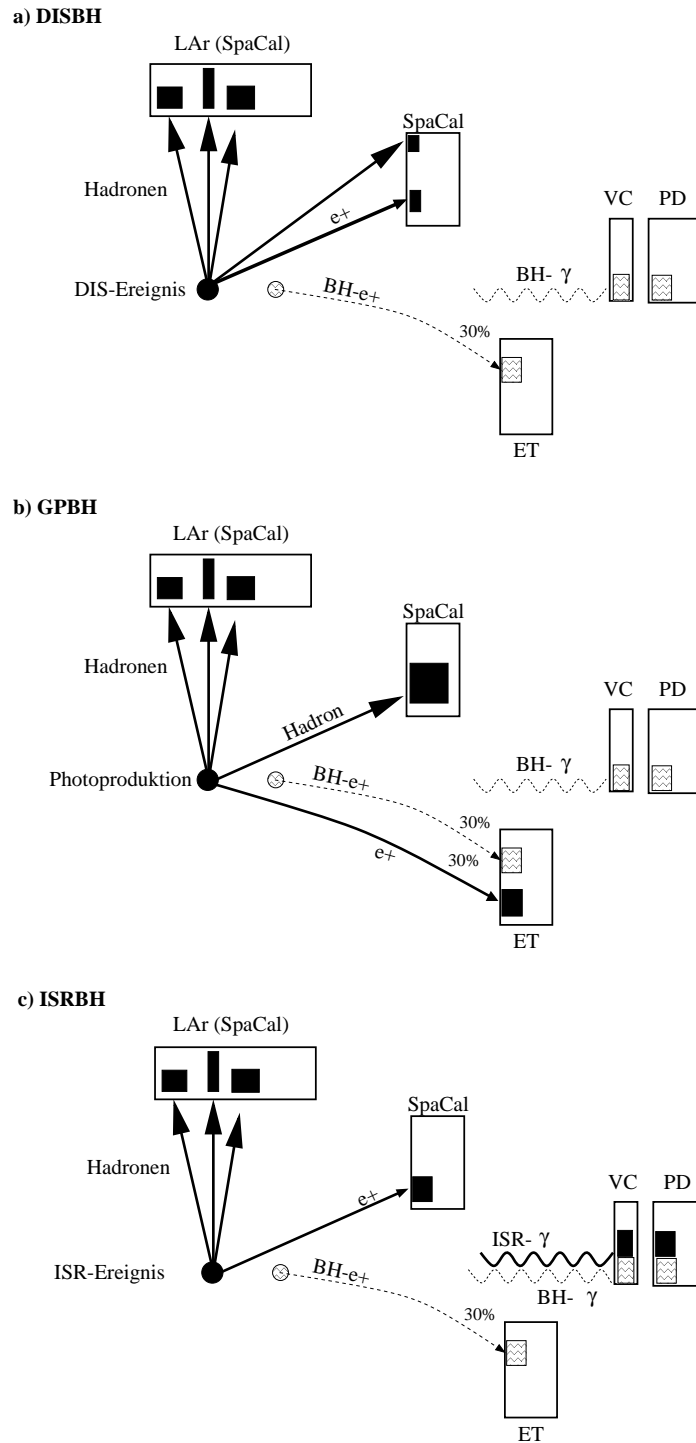
Abbildung 3.2: a) Signatur eines DISBH-Ereignisses, b) Signatur eines GPBH-Ereignisses und c) Signatur eines ISRBH-Ereignisses. Die Teilchen der tiefinelastischen Streuevents sind mit durchgezogenen Linien angedeutet. Das überlagerte BH-Ereignis ist gestrichelt dargestellt. Erläuterungen siehe Text.
