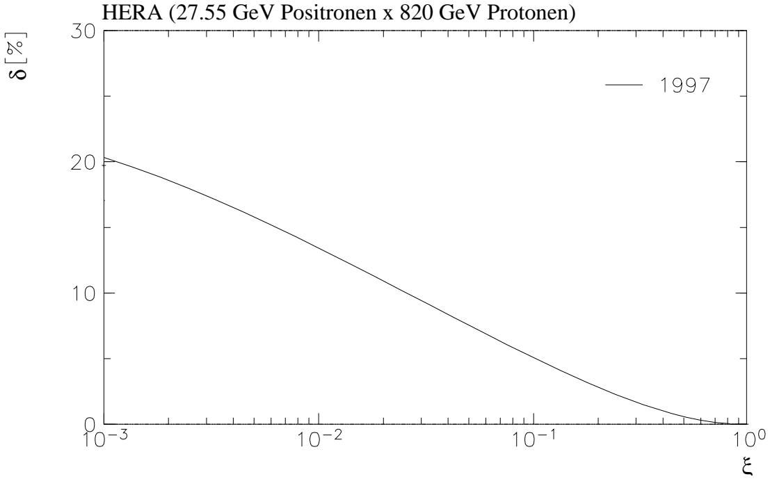
Abbildung 1.7: Korrektur \delta aufgrund der Strahlausdehnung zum BH-Wirkungsquerschnitt in Gleichung (1.34) für Stahlbedingungen des Jahres 1997 [ser98].
