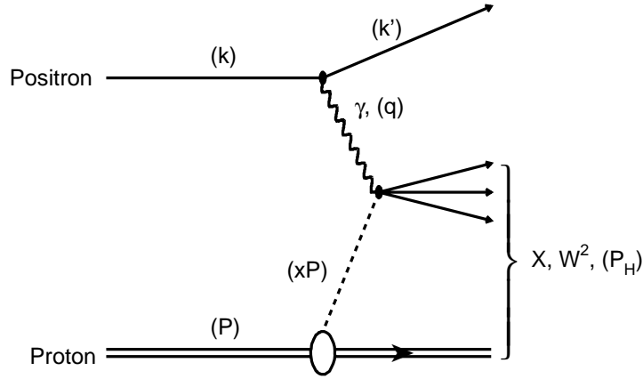
Abbildung 1.1: Schematische Darstellung des Positron-Proton-Streuprozesses mit Photonaustausch ( \gamma ) und hadronischem Endzustand ( X ) mit invarianter Masse W . Die eingeklammerten Größen bezeichnen die Viererimpulse der ein- und auslaufenden Teilchen. q ist die Virtualität des ausgetauschten Photons.
