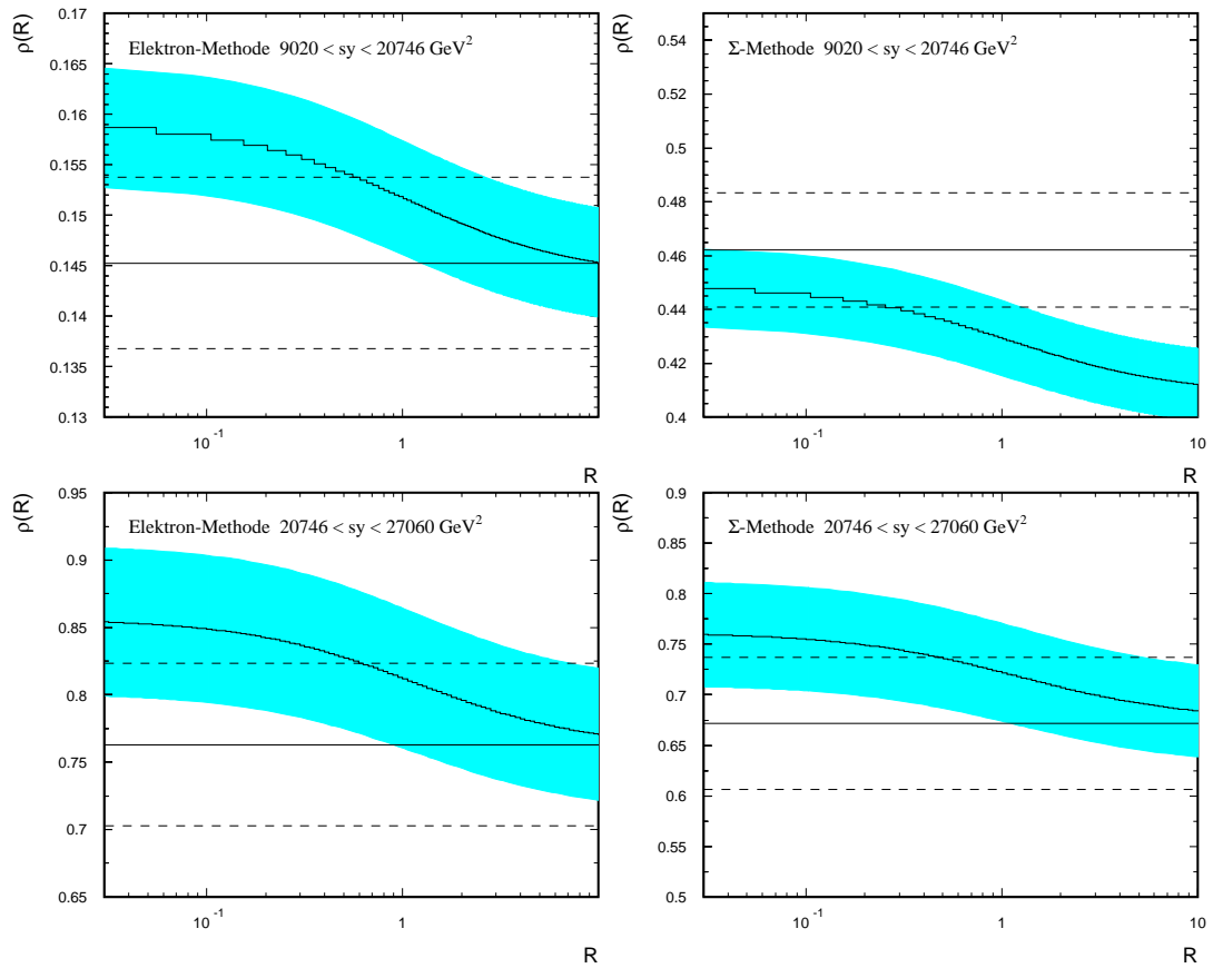
Abbildung 5.3: Vergleich der \rho_{dat} -Werte (durchgezogene Linie) für das Intervall 9020 < s_y < 20746 \text{ GeV}^2 (obere Abbildungen) und für 20746 < s_y < 27060 \text{ GeV}^2 (untere Abbildungen) jeweils mit der Elektron- und \Sigma -Methode mit der \rho(R) -Abhängigkeit aus der Simulation. Die gepunktete Linie und das Band entsprechen dem statistischen Fehler von \rho_{dat} bzw. von \rho(R) .
