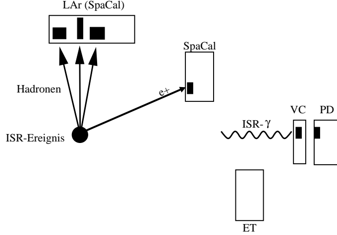
Abbildung 3.1: Schematische Darstellung der ISR-Signatur im H1-Detektor. Eingezeichnet sind das LAr-Kalorimeter (LAr), das SpaCal, der Photonarm bestehend aus Veto-Counter (VC) und Photondetektor (PD) und der Elektronendetektor (ET). Die Rechtecke in den Detektoren symbolisieren die Energiedepositionen in den jeweiligen Komponenten; dabei sei darauf hingewiesen, daß ein Teil des hadronischen Endzustandes auch im SpaCal nachgewiesen werden kann, wie entsprechend angedeutet.
