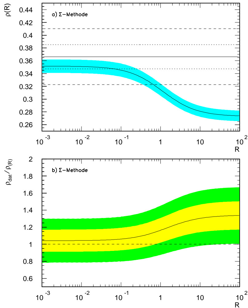
Abbildung 5.7: a) Zu sehen ist der gemessene \rho_{\text{dat}} -Wert (durchgezogene Linie) mit statistischen (gepunktete Linie) und totalen Fehler (gestrichelte Linie) im Intervall Bin3 für die \Sigma -Methode. Des weiteren ist die \rho(R) -Abhängigkeit mit ihrem statistischen Fehlerband gezeigt. b) Verhältnis aus \rho_{\text{dat}} und Funktion \rho(R) . Das Band entspricht dem totalen Fehler (hell 1\sigma , dunkel 2\sigma ).
