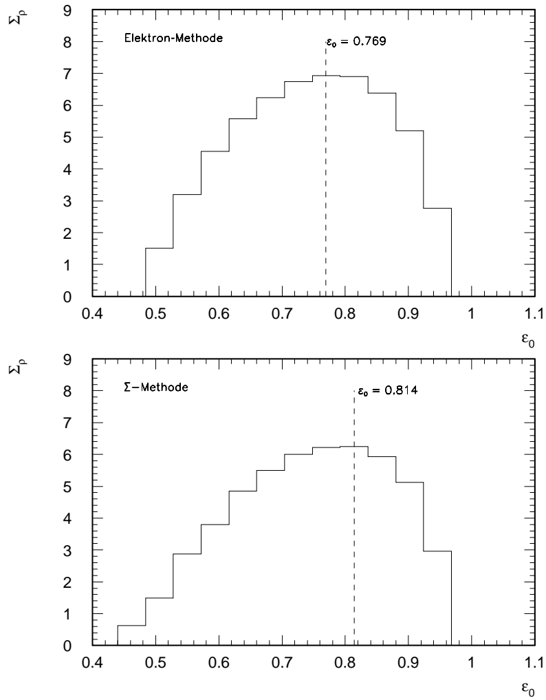
Abbildung 5.5: Signifikanz \Sigma_\rho in Abhängigkeit von \epsilon_0 im Intervall Bin3 für die Rekonstruktion mit der Elektron- und \Sigma -Methode. Die gestrichelten Linien zeigen jeweils das Maximum der Verteilung.
