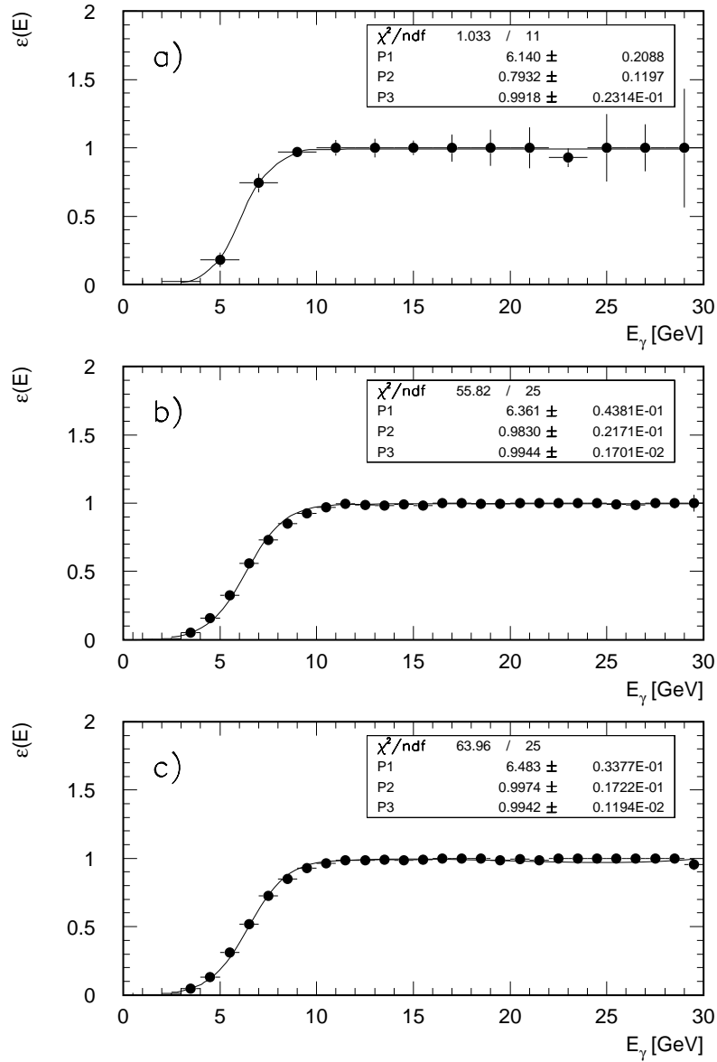
Abbildung 3.8: Effizienz des Triggerelementes LUPD_{LOW} in Abhängigkeit von der Energie im Photonarm E_\gamma für drei verschiedene Datennahmebeiche a) am Beginn, b) in der Mitte und c) am Ende des Jahres 1997. Die durchgezogene Linie ist das Ergebnis der Anpassung in Gleichung (3.24), mit P1 = E_S , P2 = B und P3 = \varepsilon_{max} .
