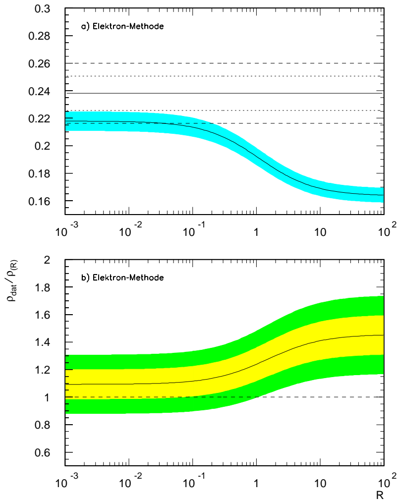
Abbildung 5.6: a) Zu sehen ist der gemessene \rho_{\text{dat}} -Wert (durchgezogene Linie) mit statistischen (gepunktete Linie) und totalen Fehler (gestrichelte Linie) im Intervall Bin3 für die Elektron-Methode. Des weiteren ist die \rho(R) -Abhängigkeit mit statistischem Fehlerband gezeigt. b) Verhältnis aus \rho_{\text{dat}} und Funktion \rho(R) . Das Band entspricht dem totalen Fehler (hell 1\sigma , dunkel 2\sigma ).
