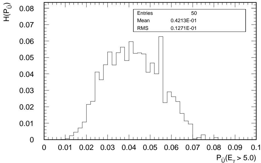
Abbildung 3.13: Häufigkeitsverteilung H(P_{\tilde{U}}) der BH-Überlappwahrscheinlichkeit mit E_\gamma > 5 \text{ GeV} für den in dieser Analyse verwendeten ISR-Datensatz.
