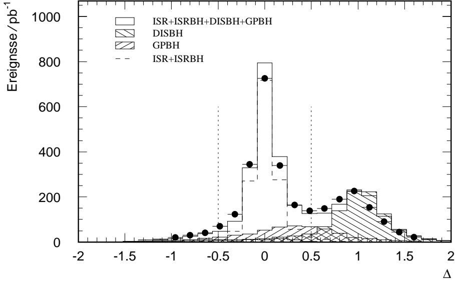
Abbildung 3.22: Verteilung der Größe \Delta für Daten (Punkte) und MC (Histogramme). Das Histogramm mit der durchgezogenen Linie ist die Summe aus den Untergrund- und ISR-Monte-Carlo-Verteilungen. Das gestrichelte Histogramm stellt die radiativen ISR-Ereignisse und ISRBH-Ereignisse dar und die beiden gefüllten Histogramme geben den GPBH- und DISBH-Untergrund an. Die senkrechten Linien kennzeichnen die Schnitte auf die Größe \Delta .
