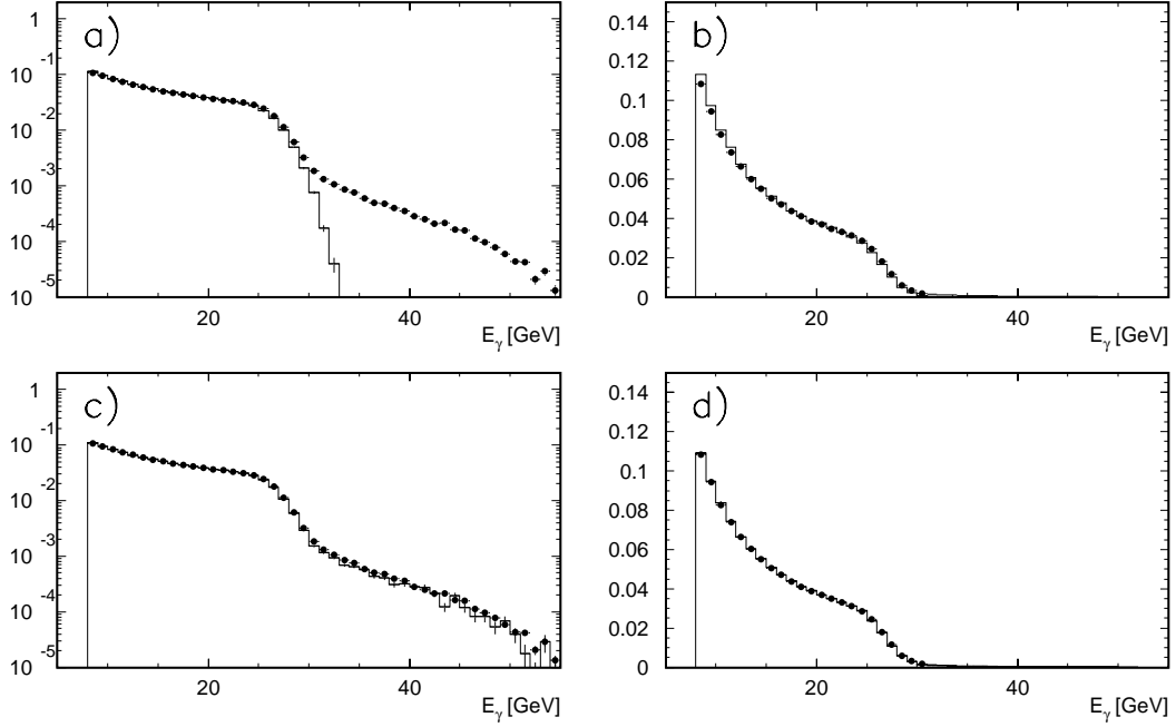
Abbildung 3.18: BH-Photonenenergieverteilung für Daten (Punkte) und generierte BH-Ereignisse (durchgezogene Linie), links logarithmisch und rechts linear aufgetragen. a),b) zeigt den Vergleich von Daten mit der BH-Simulation ohne Zufallskoinzidenz mehrerer BH-Photonen und c),d) mit Zufallskoinzidenz von ein, zwei und drei BH-Photonen.
