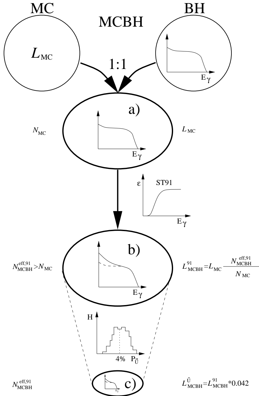
Abbildung 3.14: Schematische Darstellung der Arbeitsschritte a), b) und c) zur Simulation des DISBH- und GPBH-Untergrundes; Beschreibung siehe Text.
