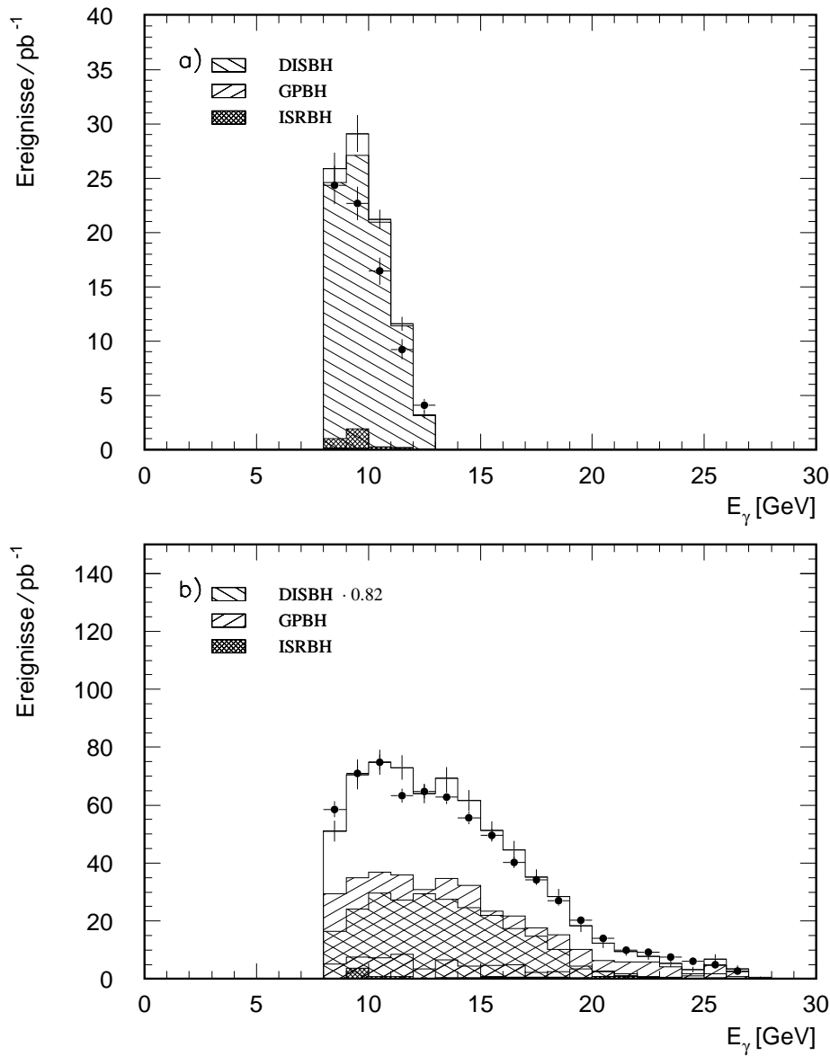
Abbildung 3.15: Photonenergiespektrum für Ereignisse mit ISR-Signatur und einer Energiedeposition im Elektrodendetektor für a) 22.0 < E_e < 30.0 GeV und b) 5.0 < E_e < 12.0 GeV. In der Abbildung b) ist der DISBH-Untergrund mit dem Normierungsfaktor 0.82 herunterskaliert (Erläuterung siehe Text). Die Punkte repräsentieren die Daten, die durchgezogene Linie ist die Summe der Untergrundsimulationen, wobei die Kreuze auf dieser Linie den statistischen Fehler des MC anzeigen. Zu sehen sind außerdem der DISBH-, GPBH- und ISRBH-Untergrund (schraffierte Histogramme).
