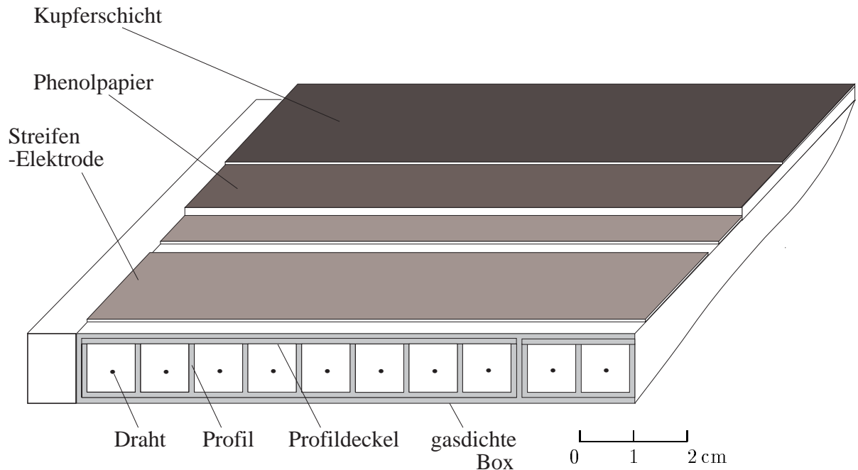
Abbildung 4.2: Schematischer Aufbau einer Streamerrohrkammer (maßstabsgetreu).
