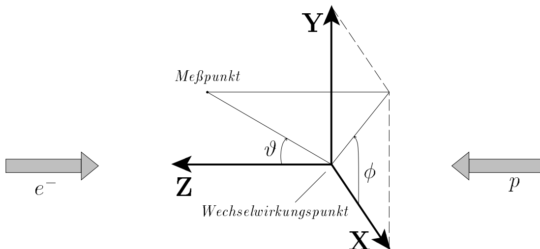
Abbildung 3.2: Das H1-Koordinatensystem.
