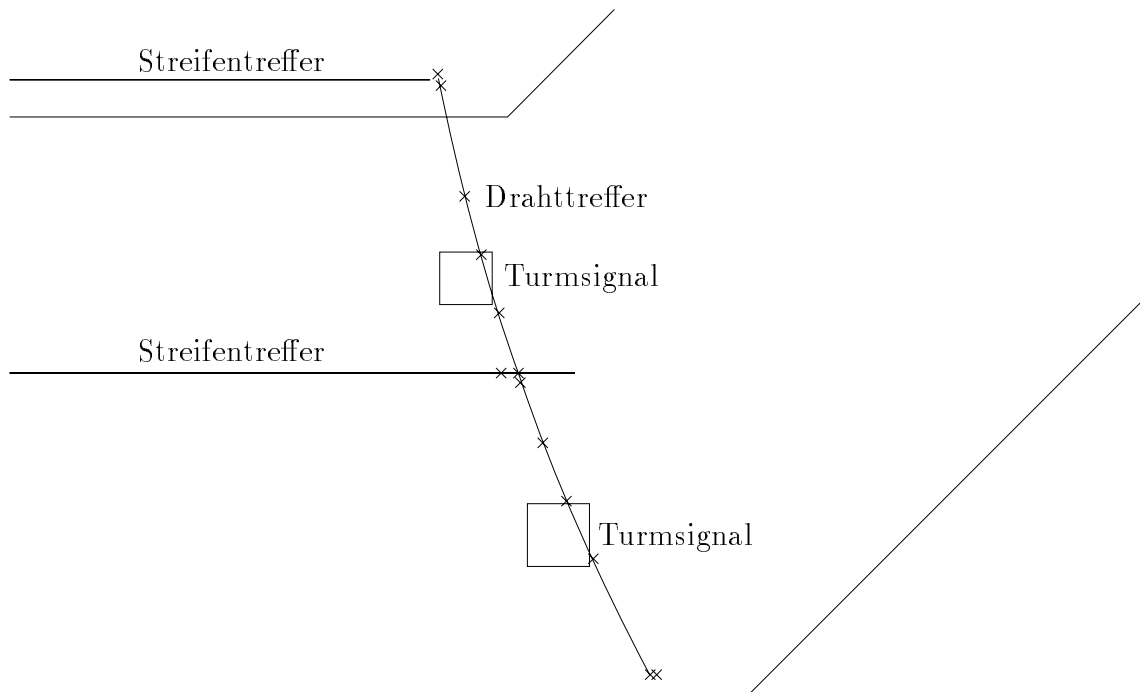
Abbildung 4.9: Beispiel einer angepassten Spur im Barrelbereich.
