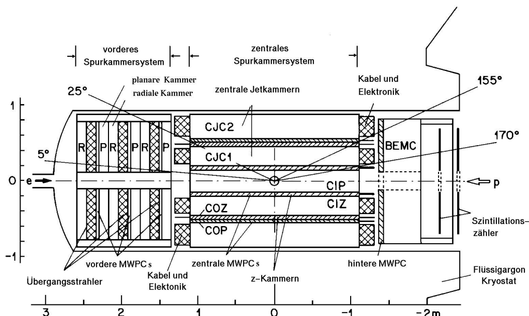
Abbildung 3.4: Das Spurkammersystem.
