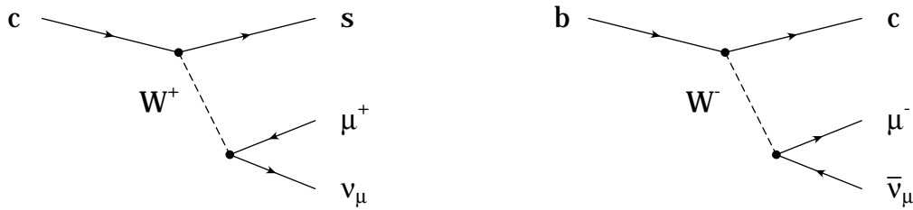
Abbildung 1.9: Der semimyonische Zerfall schwerer Quarks.
