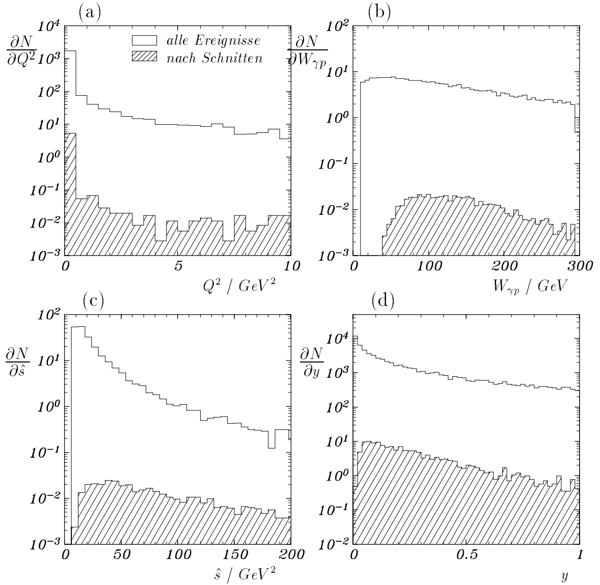
Abbildung 2.2: Kinematische Größen von Ereignissen mit c -Quarks. In (a) ist die Virtualität Q^2 , in (b) die Schwerpunktsenergie des \gamma - p -Systems W_{\gamma p} , in (c) das Quadrat der Schwerpunktsenergie des Q\bar{Q} -Systemes \hat{s} und in (d) y aufgetragen. N entspricht den nach den Wirkungsquerschnitten erwarteten Zahlen.
