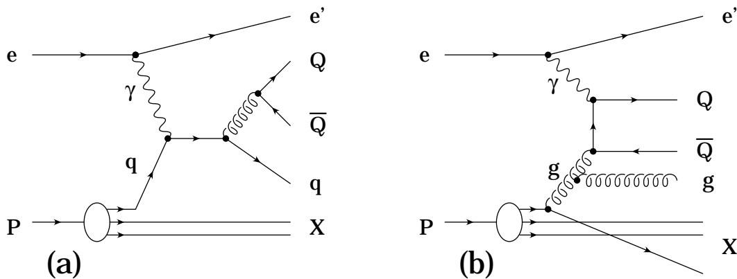
Abbildung 1.4: Beiträge höherer Ordnung in \alpha_s zur Produktion schwerer Quarks. Abbildung (a) zeigt die Erzeugung eines zusätzlichen leichten Quarks (QCD-Compton-Streuung), Abbildung (b) die Abstrahlung eines zusätzlichen Gluons.
