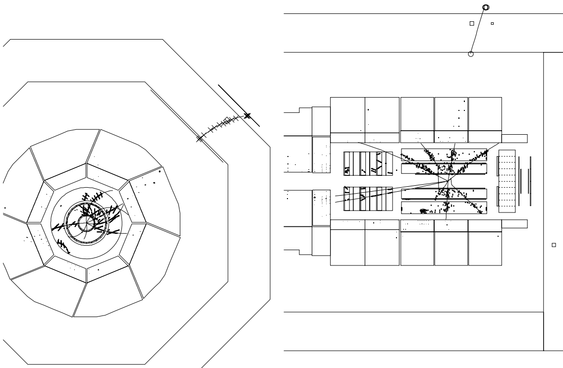
Abbildung 7.1: Beispiel eines Kandidaten für ein Ereignis mit einem prompten Myon.
