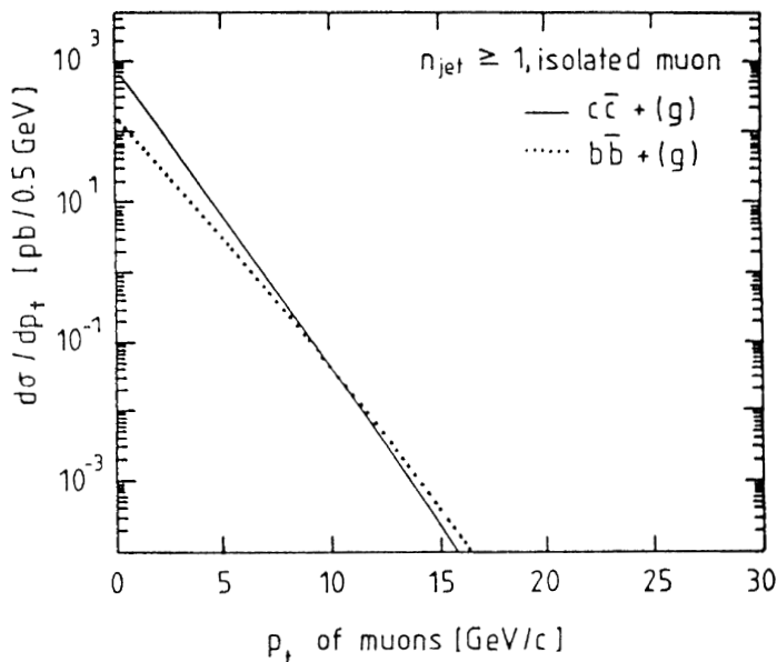
Abbildung 1.10: Verteilung des theoretisch berechneten Transversalimpulses der Myonen aus dem Zerfall schwerer Quarks [EKU88]. Es ist verlangt, daß der Fragmentationsjet des Quark gefunden worden ist und das Myon isoliert ist.
