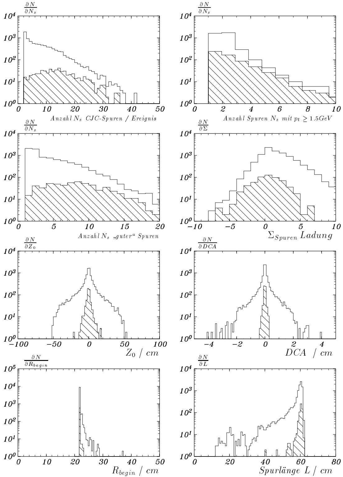
Abbildung 5.3: Verteilungen der Größen vor und nach Anwendung der Selektionskriterien 7–10.
