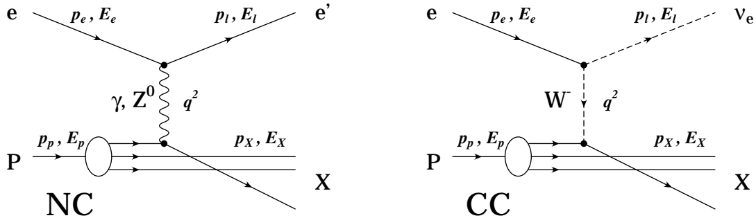
Abbildung 1.1: Feynman-Graphen für DIS-Prozesse.
