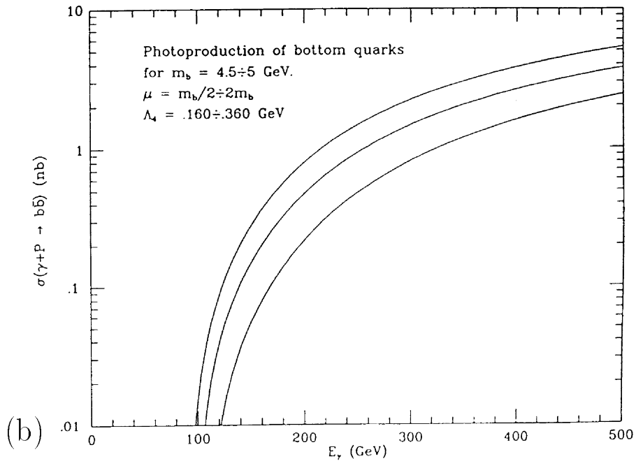
Abbildung 1.8: Totaler Wirkungsquerschnitt für c -Quark-Produktion bei der \gamma - p -Streuung als Funktion der Photonenergie E_\gamma mit gemessenen Werten mehrerer Experimente (a), totaler Wirkungsquerschnitt für b -Quark-Produktion als Funktion von E_\gamma für verschiedene m_b (b) [ELI89].
