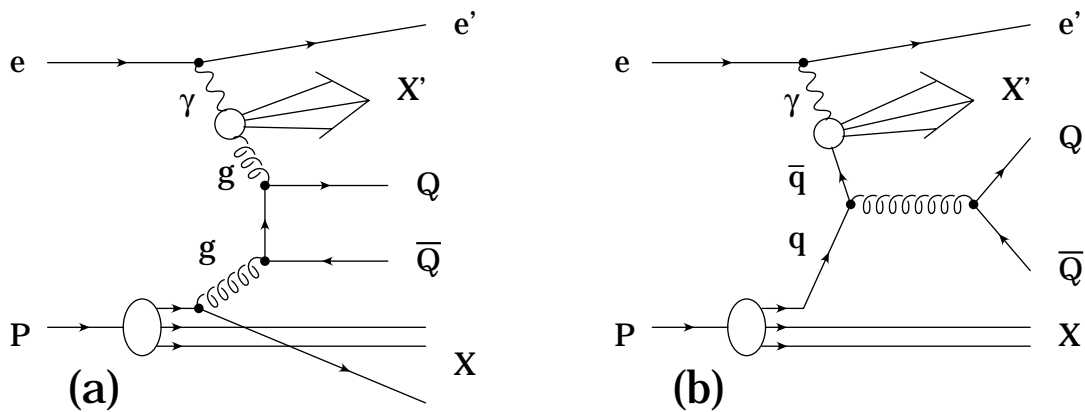
Abbildung 1.5: Feynman-Graphen für die Erzeugung schwerer Quarks mit aufgelöstem Photon. In Abbildung (a) ist der Prozeß gg \rightarrow Q\bar{Q} (Gluon-Gluon-Fusion), in Abbildung (b) der Prozeß q\bar{q} \rightarrow Q\bar{Q} gezeigt.
