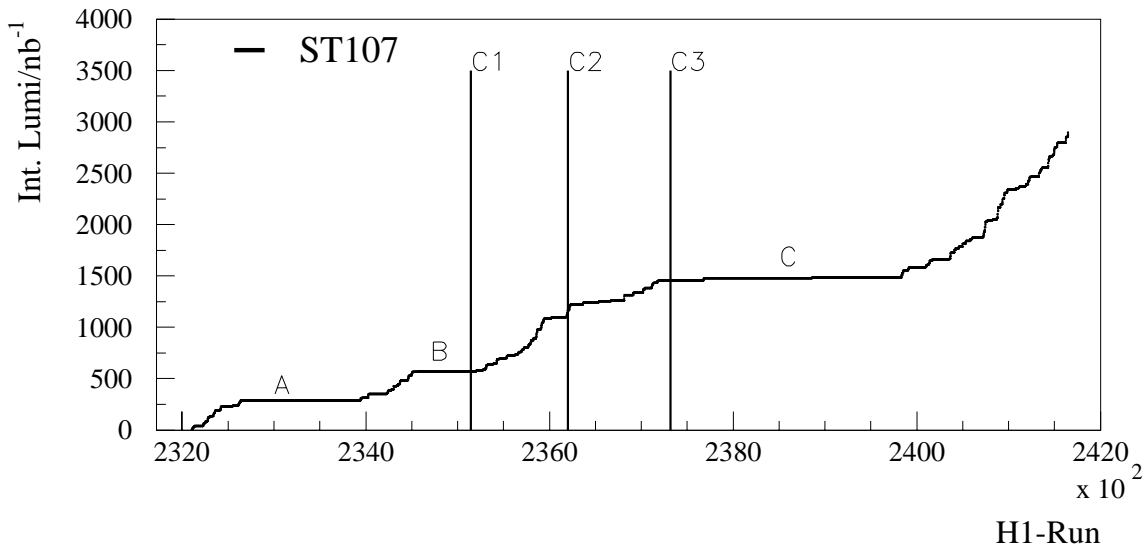
ABBILDUNG 5.1: Die integrierte Luminosität von ST107 und den Bedingungen I und II aus Tabelle 4.1 in Abhängigkeit von der H1-Runnummer für den Datennahmebereich der Analyse. Eingetragen sind zusätzlich die Zeitpunkte, an denen sich die Akzeptanz und Nachweiswahrscheinlichkeit durch zusätzliche abgeschaltete Sektoren in der zentralen Spurkammer (“C1” bis “C3”) ändert. Bereiche ohne Zunahme der Luminosität aufgrund von Problemen bei HERA (“A” und “B”) und der Hydraulik des FPS (“C”) sind ebenfalls vermerkt. Die integrierte Luminosität beträgt 2.98 \text{ pb}^{-1} .
