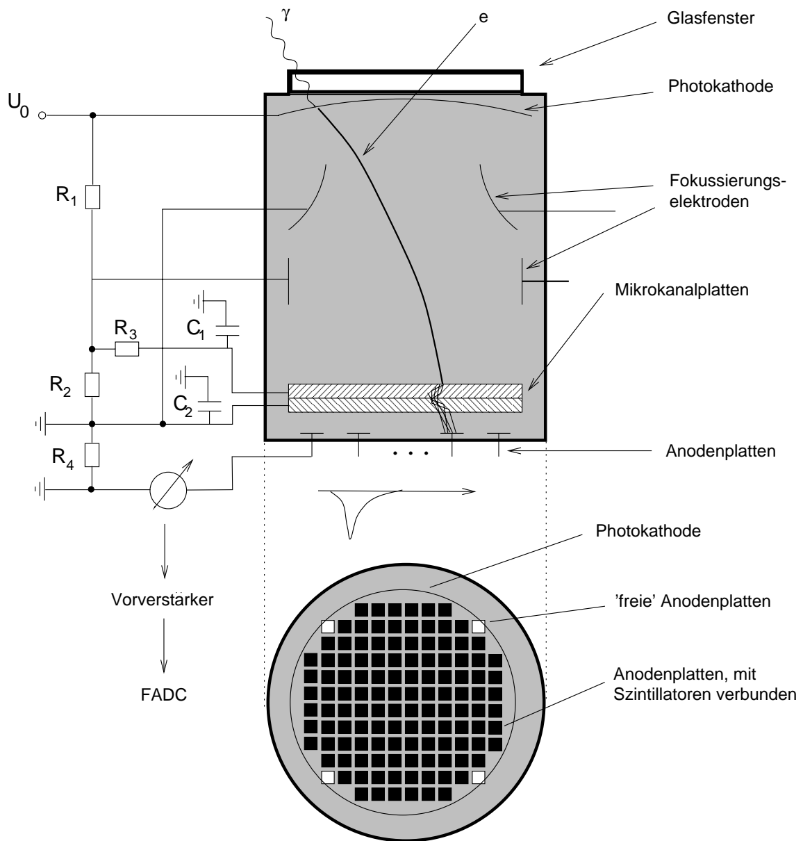
ABBILDUNG 3.8: Schematische Schnittzeichnung und Beschaltung eines MCPMs, wie er in den horizontalen Stationen verwendet wird (oben), sowie die Anordnung der Anodenplatten (unten). Ebenso ist beispielhaft der Signalweg von einem einfallenden Lichtquant aus den Lichtleitern bis hin zu den FADCs dargestellt. Die verschiedenen Widerstände und Kondensatoren haben folgende Spezifikationen: R_1 = 2 \text{ M}\Omega , R_2 = 7 \text{ M}\Omega , R_3 = 10 \text{ M}\Omega , R_4 = 1 \text{ M}\Omega , C_1 = 15 \text{ nF} und C_2 = 1.6 \text{ nF} . Die angelegte Hochspannung beträgt etwa U_0 = 2800 \text{ V} .
