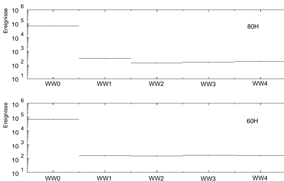
ABBILDUNG 4.5: FPS-Triggersignale in den beiden horizontalen Stationen, in Abhängigkeit von der e\gamma -Wechselwirkung. Das Triggersignal in der e\gamma -Wechselwirkung 0 (WW0) ist ein Koinzidenzsignal beider Stationen, die aus den nachfolgenden WW1 bis WW4 sind Einzelzählraten jeder Station. Für eine Untergrundabschätzung müssen diese bezüglich des Koinzidenzsignals beider Detektoren korrigiert werden.
