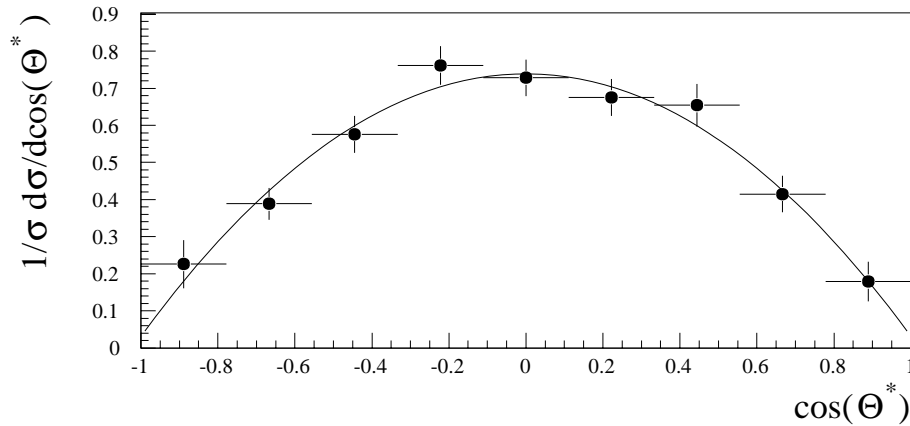
ABBILDUNG 6.14: Der differentielle Wirkungsquerschnitt d\sigma/d\cos(\theta^*) normiert auf den Gesamtwirkungsquerschnitt. Die eingezeichnete Funktion ergibt sich aus einer Anpassung gemäß Gleichung 6.11 und liefert einen Wert für r_{00}^{04} von 0.030 \pm 0.030(\text{stat.}) \pm 0.010(\text{syst.}) .
