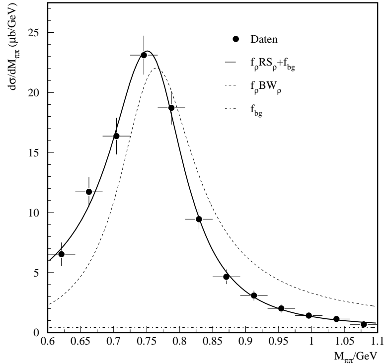
ABBILDUNG 6.3: Dargestellt ist die Verteilung des differentiellen Wirkungsquerschnittes d\sigma/dM_{\pi\pi} sowie die Anpassung der Resonanzkurve nach der Parametrisierung von Ross-Stodolsky (durchgezogene Linie, siehe Gleichung 6.6). Die strichpunktierte Linie zeigt den Untergrundanteil und die unterbrochene Linie den resonanten Anteil BW_\rho(M_{\pi^+\pi^-}) . Dieser wird erhalten, indem n = 0 gesetzt wird. Es sind nur die statistischen Fehler eingezeichnet.
