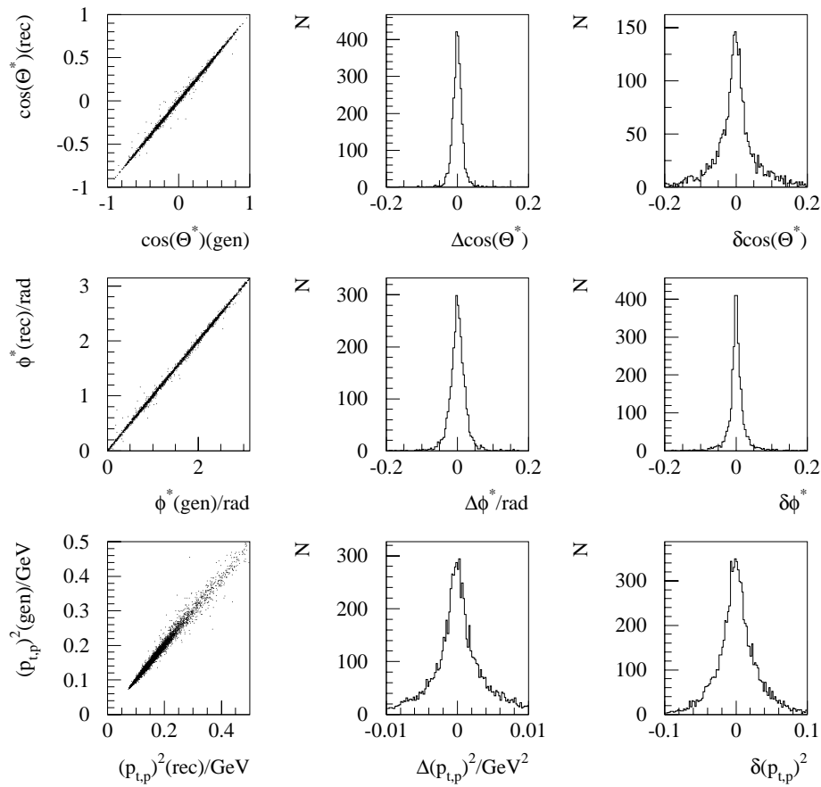
ABBILDUNG 5.28: Die Korrelationen der generierten und rekonstruierten Meßgrößen \cos(\Theta^*) , \phi^* und p_{t,p}^2 , sind in der linken Spalte dargestellt. Die daraus berechneten absoluten und relativen Auflösungen sind in der mittleren und rechten Spalte zusehen. Die Werte sind in Tabelle 5.1 aufgelistet.
