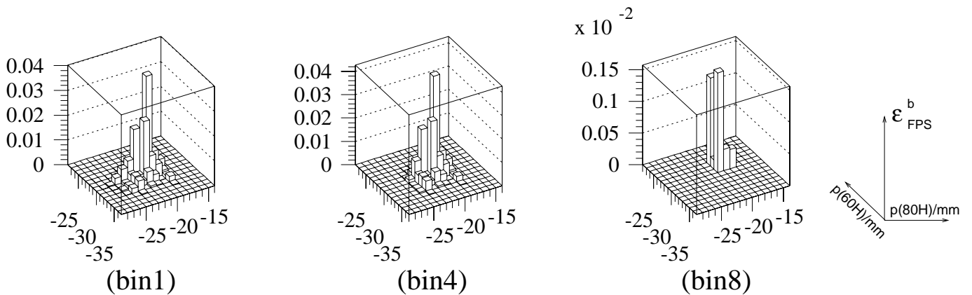
ABBILDUNG 5.13: Akzeptanz des FPS \epsilon_{FPS}^b bei realen Detektorpositionen in 3 Intervallen für p_x, p'_x . Für die hier dargestellten Verteilungen wurden die Rekonstruktionseffizienz aus Abbildung 5.12 mit den relativen Häufigkeiten der Positionen beider Detektoren multipliziert. Die Summe aller Einträge in diesen Häufigkeitsverteilungen aller Intervalle 1 bis 8 ergibt 100% und damit die Verteilung aller Detektorpositionen.
