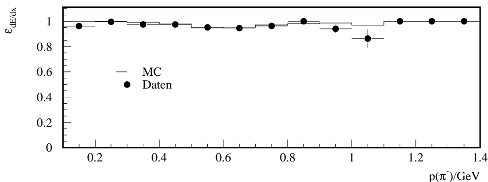
ABBILDUNG 5.6: Ansprechwahrscheinlichkeit \epsilon_{dE_\pi/dx} der Erkennung von negativen Pionen mit der im Text erklärten Methode in Abhängigkeit vom Impuls der Pionen. Der Vergleich zwischen der Monte-Carlo-Simulation (MC) und den Daten zeigt eine gute Übereinstimmung.
