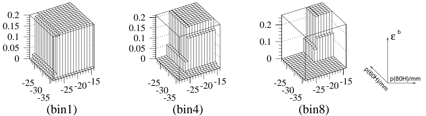
ABBILDUNG 5.12: Rekonstruktionseffizienz \epsilon^b für Protontrajektorien des FPS bei variablen Detektorpositionen in 3 Intervallen für p_x, p'_x . Für die hier dargestellten Verteilungen wurde die Anzahl der rekonstruierten Protontrajektorien (aus Abbildung 5.11) durch die Anzahl in dem jeweiligen Intervall generierten Protontrajektorien dividiert.
