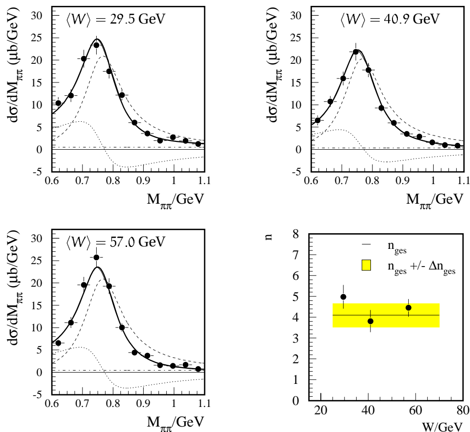
ABBILDUNG 6.5: Die Verteilung der invarianten Masse für die drei W -Intervalle. Das Söding-Modell wurde für die Anpassungen wie in Abbildung 6.2 herangezogen. Der Schiefe-Parameter für diese Verteilungen ist unten rechts dargestellt. Es sind nur statistische Fehler eingezeichnet. Die durchgezogene Linie entspricht dem angepassten Parameter für die gesamte Datenmenge n_{\text{ges}} , das graue Band zeigt den Bereich des statistischen Fehlers \Delta n_{\text{ges}} um den Mittelwert (siehe Tabelle 6.1).
