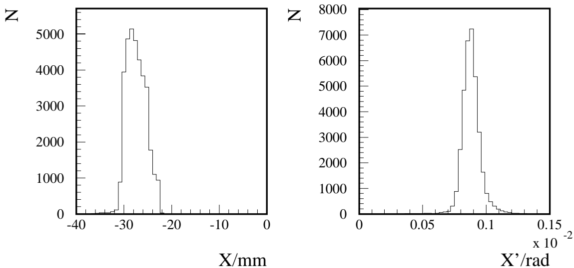
ABBILDUNG 3.12: Verteilung der rekonstruierten Protontrajektorien im FPS. Dargestellt ist die X -Koordinate des Durchstoßpunktes sowie die Steigung X' in der horizontalen Ebene der Spuren bei z = 72 m im HERA-Koordinatensystem. Deutlich wird der begrenzte Akzeptanzbereich der horizontalen Stationen.
