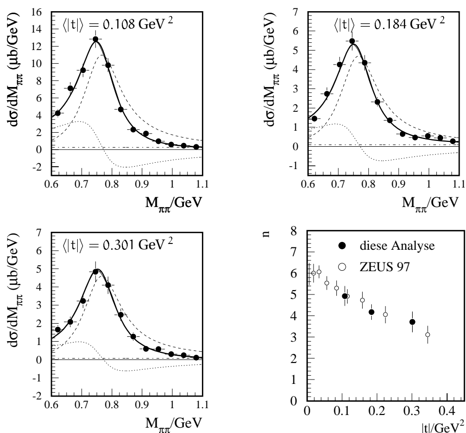
ABBILDUNG 6.4: Die Verteilung der invarianten Masse für die drei Intervalle in der Variablen |t| . Das Söding-Modell wurde für die Anpassungen wie in Abbildung 6.2 herangezogen. Der Schiefe-Parameter für diese Verteilungen ist unten rechts dargestellt. Neben den Punkten aus dieser Analyse sind Messungen von der ZEUS-Kollaboration aufgeführt [ZEU98]. Es sind nur statistische Fehler eingezeichnet.
