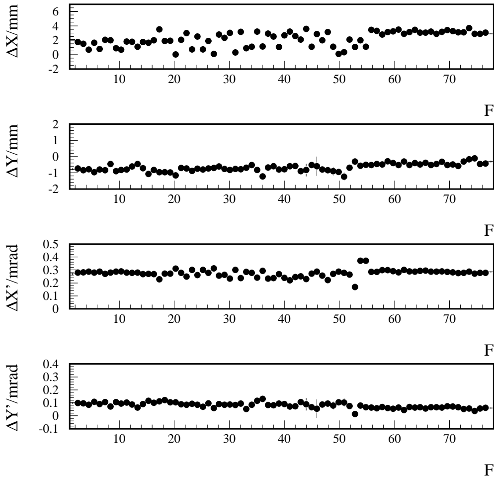
ABBILDUNG 3.15: Kalibrationskonstanten für die horizontalen Stationen. Sie sind gegenüber der Nummer der Luminositätsfüllung F dargestellt, in der die Bedingungen für die Datennahme mit dem FPS erfüllt waren. Die Fehler liegen im Mittel unter 5% und sind in der Abbildung nicht erkennbar.
