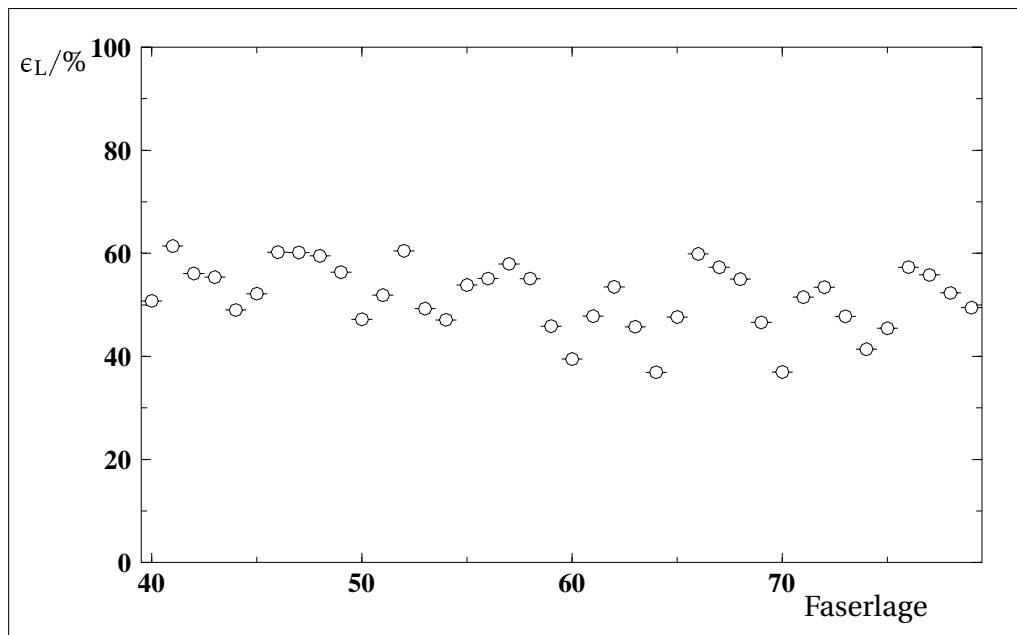
ABBILDUNG 5.8: Lagenansprechwahrscheinlichkeit \epsilon_L der Faserhodoskope der horizontalen Stationen. Pro Subdetektor gibt es 2 mal 5 Lagen, so daß insgesamt 40 Lagen ausgelesen werden. Die Lageneffizienz kann aufgrund des Hodoskopdesigns nicht größer werden als ca. 80% und beträgt hier im Mittel etwa 50%.
