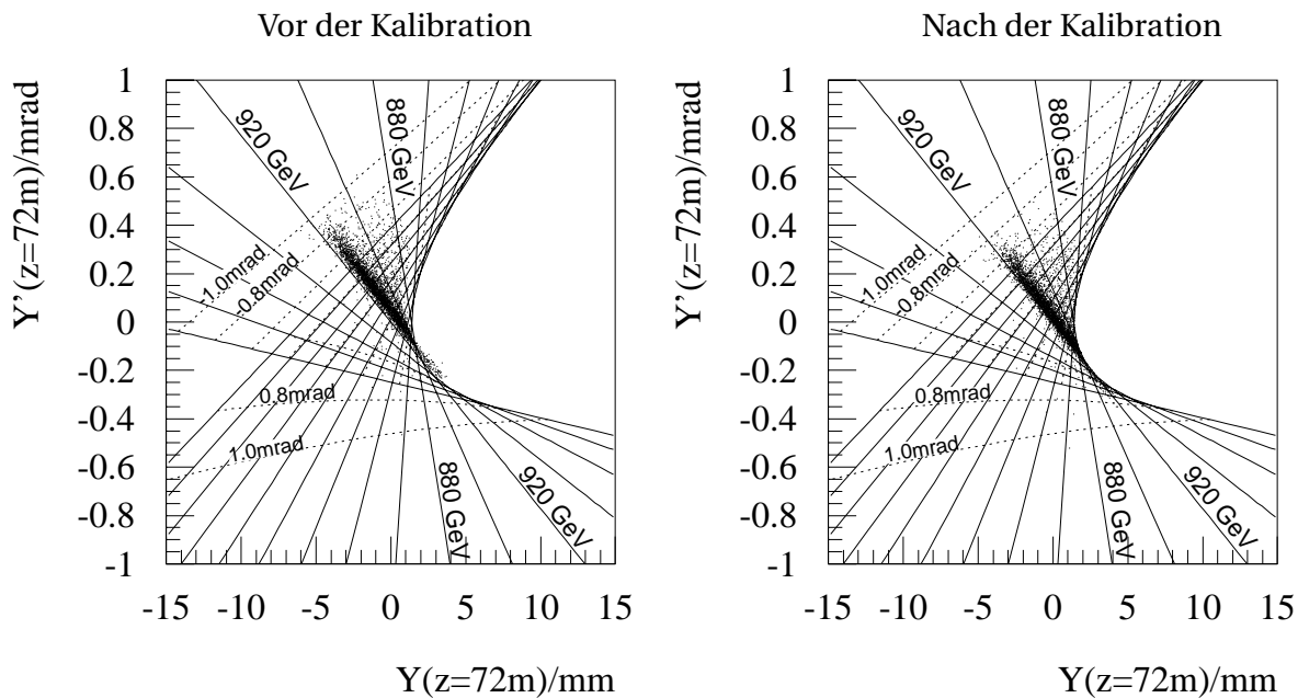
ABBILDUNG 3.13: Kalibration in der vertikalen Ebene. Dargestellt ist die Verteilung der Ablage Y und der Winkel Y' am Aufpunkt der Protontrajektorie bei z = 72 m. Eingezeichnet sind zudem die Linien mit konstanter Energie (durchgezogen). Beispielfhaft sind die mit E_{p'} = 900 GeV und E_{p'} = 880 GeV markiert. Der Abstand zweier aufeinander folgender durchgezogener Isoenergielinien beträgt 50 GeV. Die unterbrochenen Linien bezeichnen konstante Winkel \Theta_y der Protonen. Der Abstand zweier aufeinander folgender Isowinkellinien beträgt 0.5 mrad. Die Verteilungen vor der Kalibration finden sich links, die danach in der rechten Darstellung.
