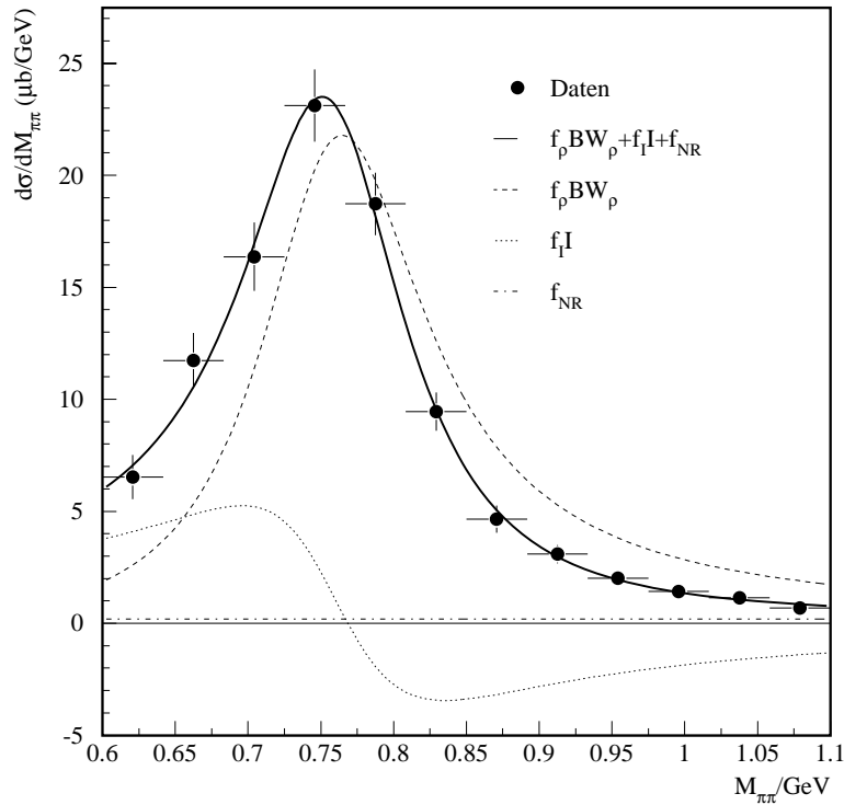
ABBILDUNG 6.2: Die Verteilung des differentiellen Wirkungsquerschnittes d\sigma/dM_{\pi\pi} . Die durchgezogene Linie stammt aus einer Anpassung nach dem Modell von Söding (siehe Gleichung 6.4). Die unterbrochene Linie zeigt den resonanten und die strichpunktirierte Linie den nichtresonanten Anteil. Die gepunktete Linie beschreibt die Interferenzverteilung. Es sind nur die statistischen Fehler eingezeichnet.
