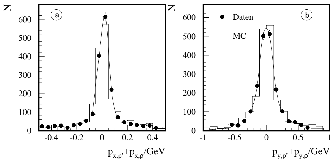
ABBILDUNG 5.22: Vergleich der Simulation mit den Daten. Dargestellt sind die Summen des Impulses des Protons ( p_{x,p'} bzw. p_{y,p'} ) und des \rho -Mesons ( p_{x,\rho} bzw. p_{y,\rho} ). Eine Anpassung mit einer Summe von zwei Gaußfunktionen liefert für die x -Koordinate in Abbildung a) einen Mittelwert \mu_x = (0.013 \pm 0.014) \text{ GeV} und für die Breite einen Wert von \sigma_x = (0.037 \pm 0.002) \text{ GeV} . Für die y -Koordinate in Abbildung b) ergeben sich \mu_y = (-0.0026 \pm 0.0037) \text{ GeV} und \sigma_y = (0.096 \pm 0.005) \text{ GeV} .
