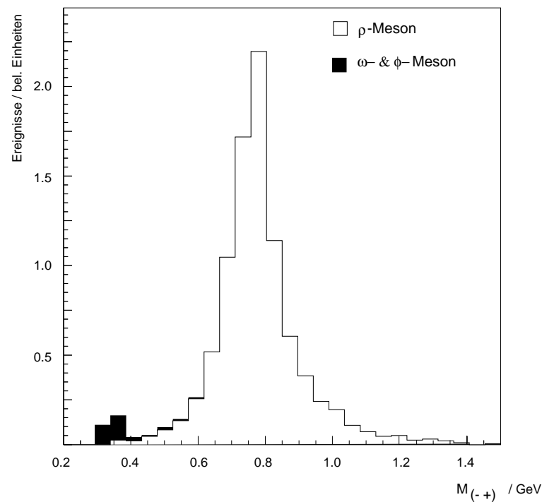
ABBILDUNG 4.6: Simulationstudie zum Untergrund durch die diffraktive elastische Photoproduktion von \omega - und \phi -Mesonen. Dargestellt ist die invariante Masse von ungleichgeladenen Teilchen unter der Annahme, daß es sich um Pionen handelt. Das offene Histogramm zeigt die Verteilung des \rho -Mesons, das schwarze zusätzlich die des \omega - und \phi -Mesons. Die benutzten Analyseschritte wurden auf alle Ereignisse angewendet, die relativen Wirkungsquerschnitte und Verzweungsverhältnisse der Vektormesonen wurden berücksichtigt.
