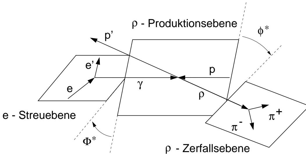
ABBILDUNG 2.3: Definition der Ebenen und Winkel für die Analyse der Zerfallswinkelverteilung bei ep \rightarrow e'\rho p' im Photon-Proton Ruhesystem.
