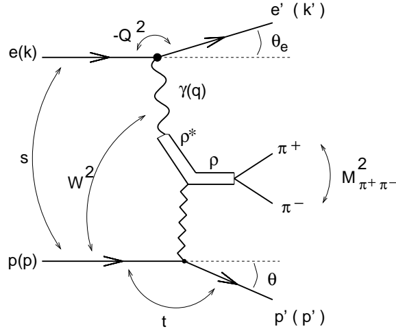
ABBILDUNG 2.2: Diffraktive elastische \rho^0 -Meson Photoproduktion bei HERA.
