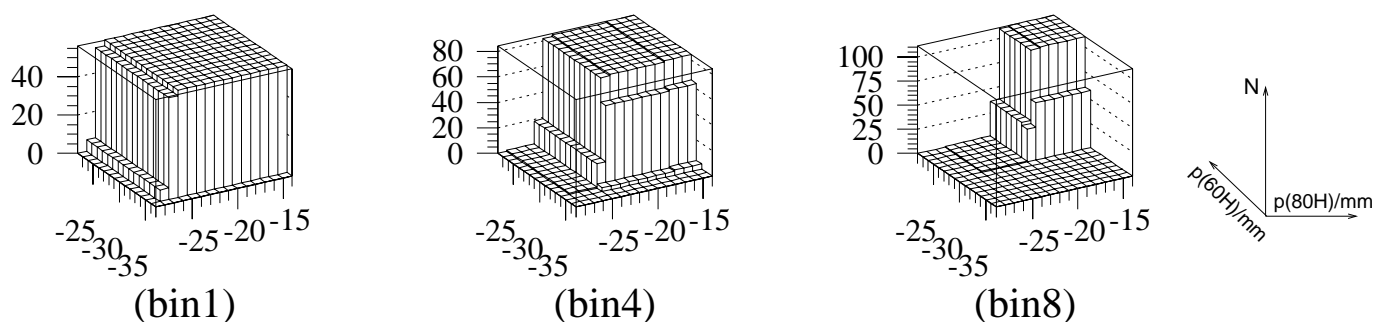
ABBILDUNG 5.11: Rekonstruktion von Protontrajektorien im FPS bei variablen Detektorpositionen. Es sind beispielhaft 3 Meßbereiche von p_{x,p'} dargestellt. Auf der x- und y-Achse sind die Positionen beider Detektoren dargestellt, bei 0 mm befindet sich der Protonenstrahl, die Impulse p_{x,p'} nähern sich dort einem Wert von p_{x,p'} = 0 GeV. In das dargestellte Histogramm wurde ein Eintrag gemacht, wenn bei den jeweiligen Detektorpositionen von 80H und 60H ein Protonimpuls im FPS rekonstruiert werden kann.
