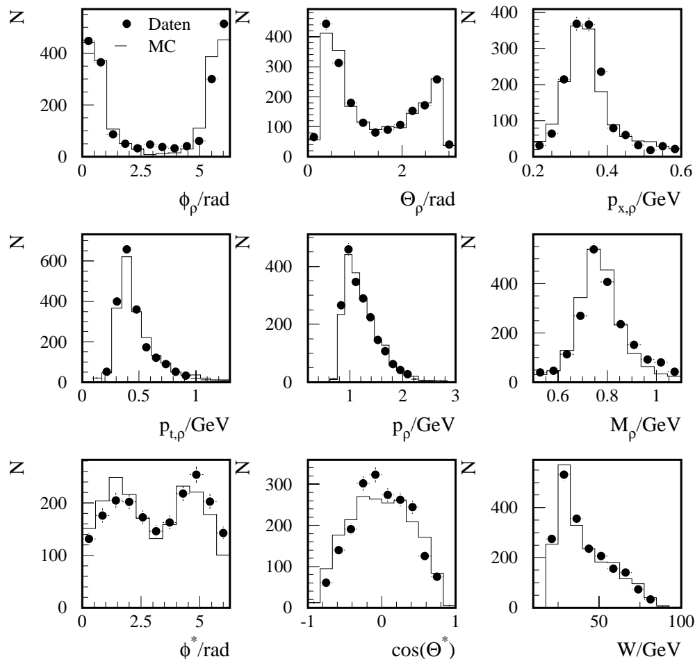
ABBILDUNG 5.19: Vergleich der Daten mit der Simulation. Dargestellt sind die Verteilungen für die kinematischen Variablen des rekonstruierten \rho -Mesons sowie W . Die Punkte beschreiben die Daten, das Histogramm die Simulation.
