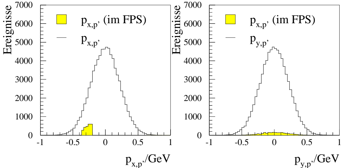
ABBILDUNG 5.10: Akzeptanz des FPS bei festen Detektorpositionen. Das offene Histogramm stellt die Impulsverteilung des gestreuten Protons auf Generatorniveau dar. Das graue Histogramm stammt von den Protonen, bei denen ein Impuls im FPS rekonstruiert wird.
