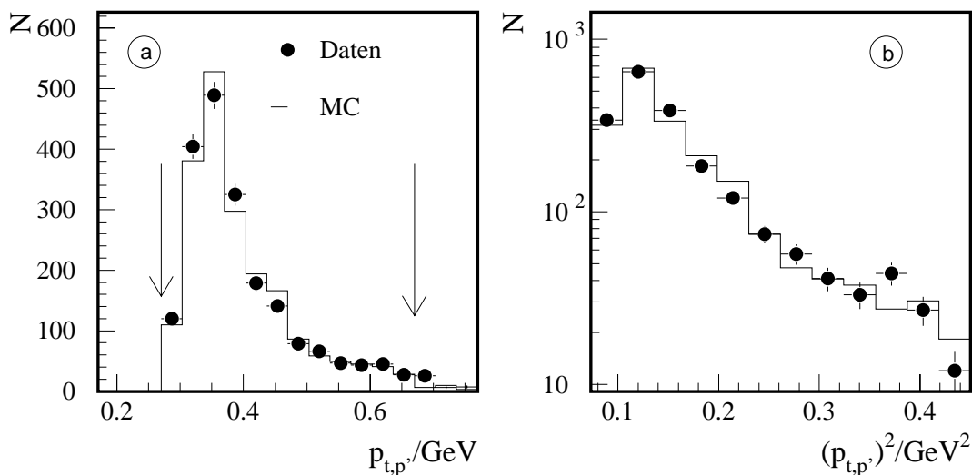
ABBILDUNG 5.21: Vergleich der Simulation und Daten. Dargestellt sind die Verteilungen der mit dem FPS gemessenen Transversalimpuls p_{t,p'} (Abbildung a). Eingezeichnet sind die Grenzen, innerhalb derer die Daten selektiert werden. In Abbildung b) ist die Verteilung von p_{t,p'}^2 in diesem Bereich ( 0.073 \text{ GeV}^2 < p_{t,p'}^2 < 0.450 \text{ GeV}^2 ) zu sehen.
