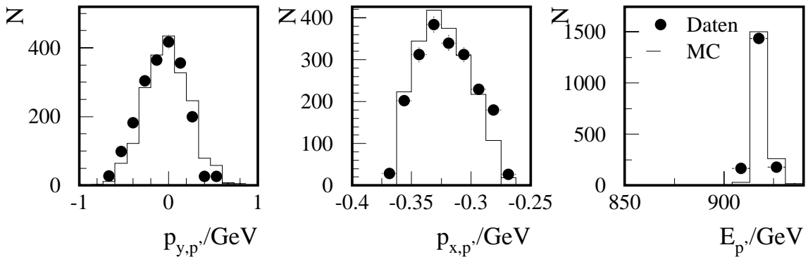
ABBILDUNG 5.20: Vergleich der Simulation und Daten. Dargestellt sind die Verteilungen der mit dem FPS gemessenen Impulse p_{y,p'} und p_{x,p'} und der Energie E_{p'} .
