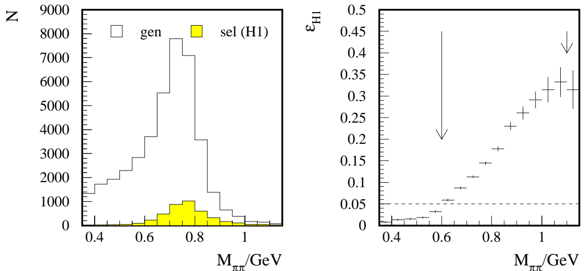
ABBILDUNG 5.23: Das offene Histogramm (“gen”) links zeigt die generierte Verteilung der invarianten Masse im Bereich von 25 \text{ GeV} < W < 70 \text{ GeV} und 0.073 \text{ GeV}^2 < p_{t,p'}^2 < 0.450 \text{ GeV}^2 . Nach den H1-relevanten Selektionskriterien verbleibt die graue Verteilung (“sel (H1)”). Rechts ist die sich daraus ergebende Effizienz dargestellt. Der Massenbereich, der in der Analyse betrachtet wird, ist mit Pfeilen gekennzeichnet. Der Wert \epsilon_{H1} = 5\% ist durch die unterbrochene Linie eingezeichnet.
