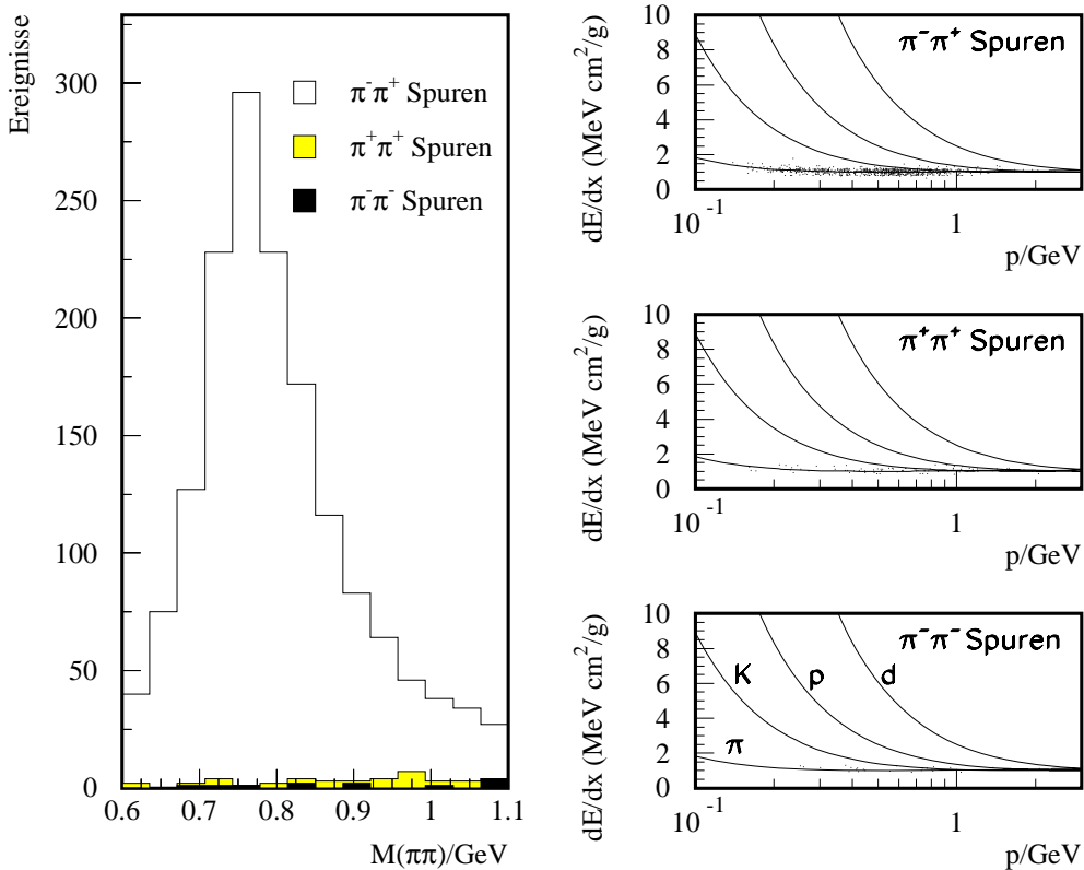
ABBILDUNG 4.3: Darstellung der invarianten Masse von Zweispurereignissen nach einer Auswahl auf LN_\pi > 0.05 (links). Mit dem hellen bzw. schwarzen Histogramm sind die doppelt positiv bzw. doppelt negativ geladenen Zweipion-Ereignisse gekennzeichnet. Rechts sind die dazugehörigen Energieverluste in Abhängigkeit der Impulse der Teilchen aufgezeigt.
