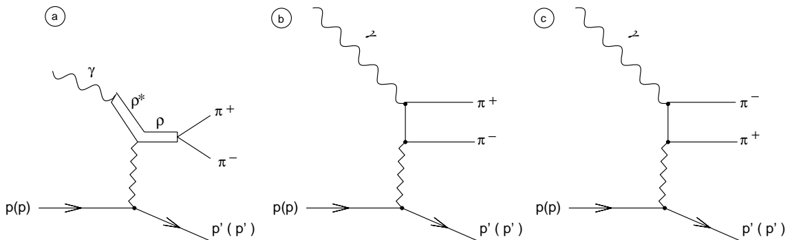
ABBILDUNG 6.1: Produktionsmechanismen von \pi^+\pi^- -Paaren, die in dem Modell von Söding betrachtet werden. In Abbildung a) ist der Prozeß der resonanten \rho -Produktion dargestellt sowie in b) und c) der Prozeß der nichtresonanten \pi^+\pi^- -Produktion. Experimentell sind die Prozesse in b) und c) nicht unterscheidbar.
