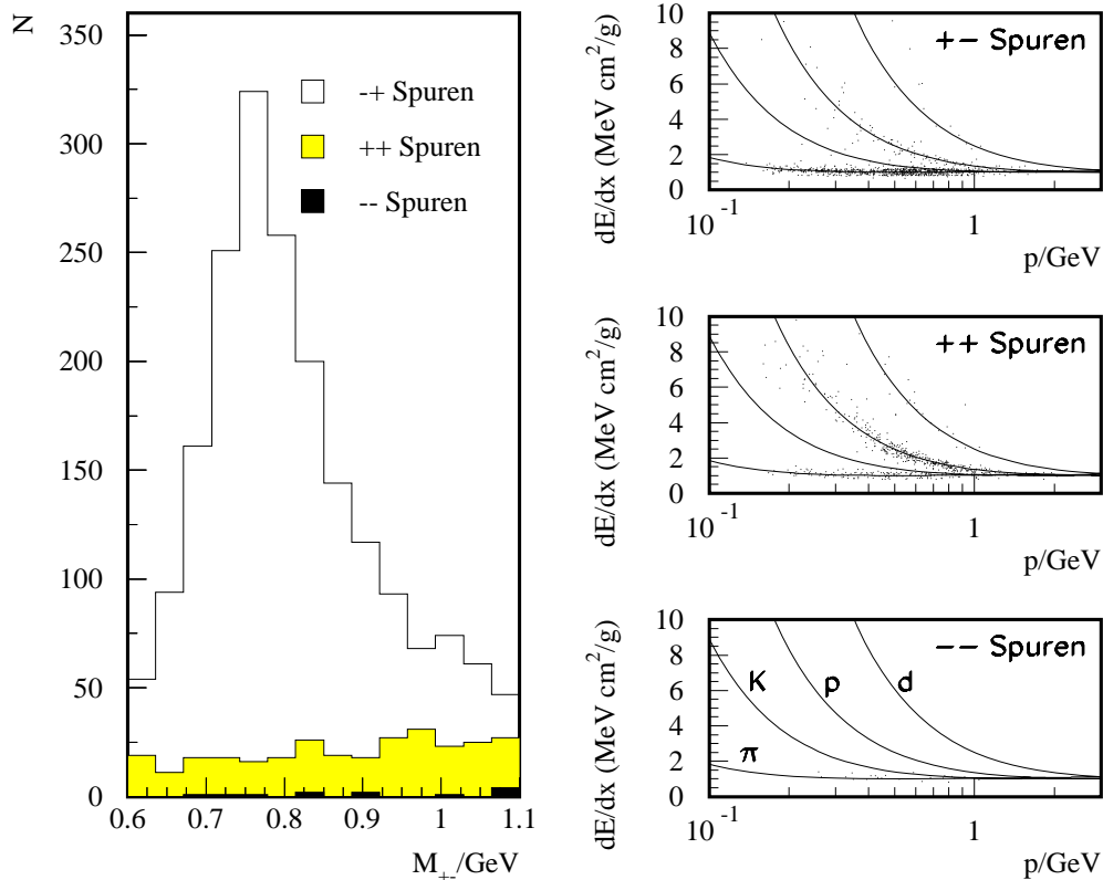
ABBILDUNG 4.2: Darstellung der invarianten Masse von Zweispurereignissen (links) nach den Auswahlkriterien I bis VII aus Abschnitt 4.1. Mit dem grauen und schwarzen Histogramm sind zusätzlich die doppelt positiv und doppelt negativ geladene Zweispurereignisse eingezeichnet. Rechts sind die dazugehörigen Energieverluste in Abhängigkeit von den Impulsen der Teilchen aufgetragen. Die gezeigten Funktionen ergeben sich mit den verschiedenen Massenhypothesen ( d -Deuterium, p -Proton, K -Kaon, \pi -Pion) aus der Bethe-Bloch -Formel 4.1.
