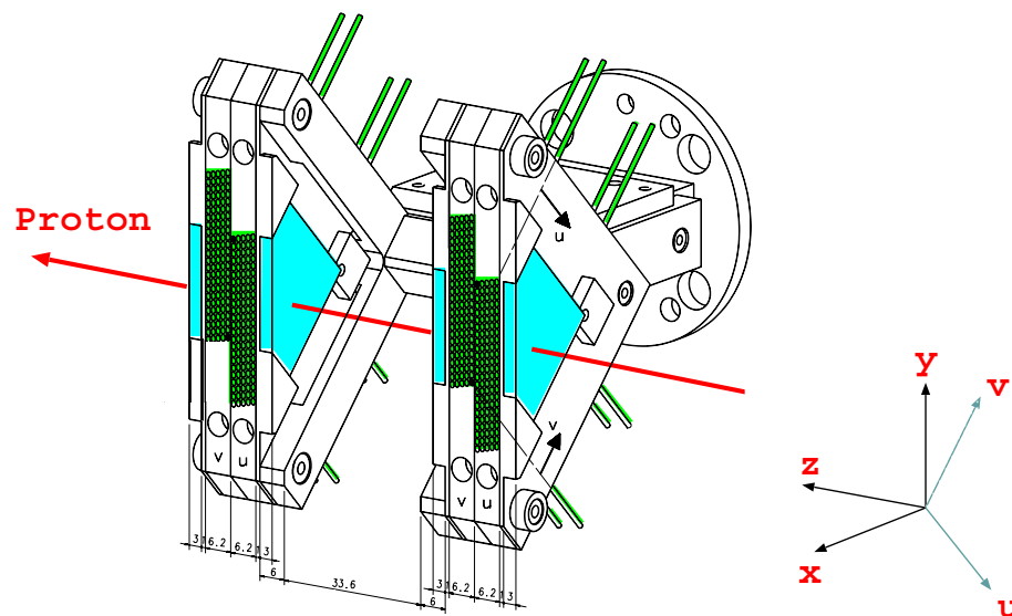
ABBILDUNG 3.6: Der Detektor der horizontalen Stationen mit dem Detektorträger, den Faserhodoskopen und flächigen Trigger-Szintillatoren. Die Flugrichtung eines nachzuweisenden Protons ist angedeutet. Die Angaben sind in mm.
