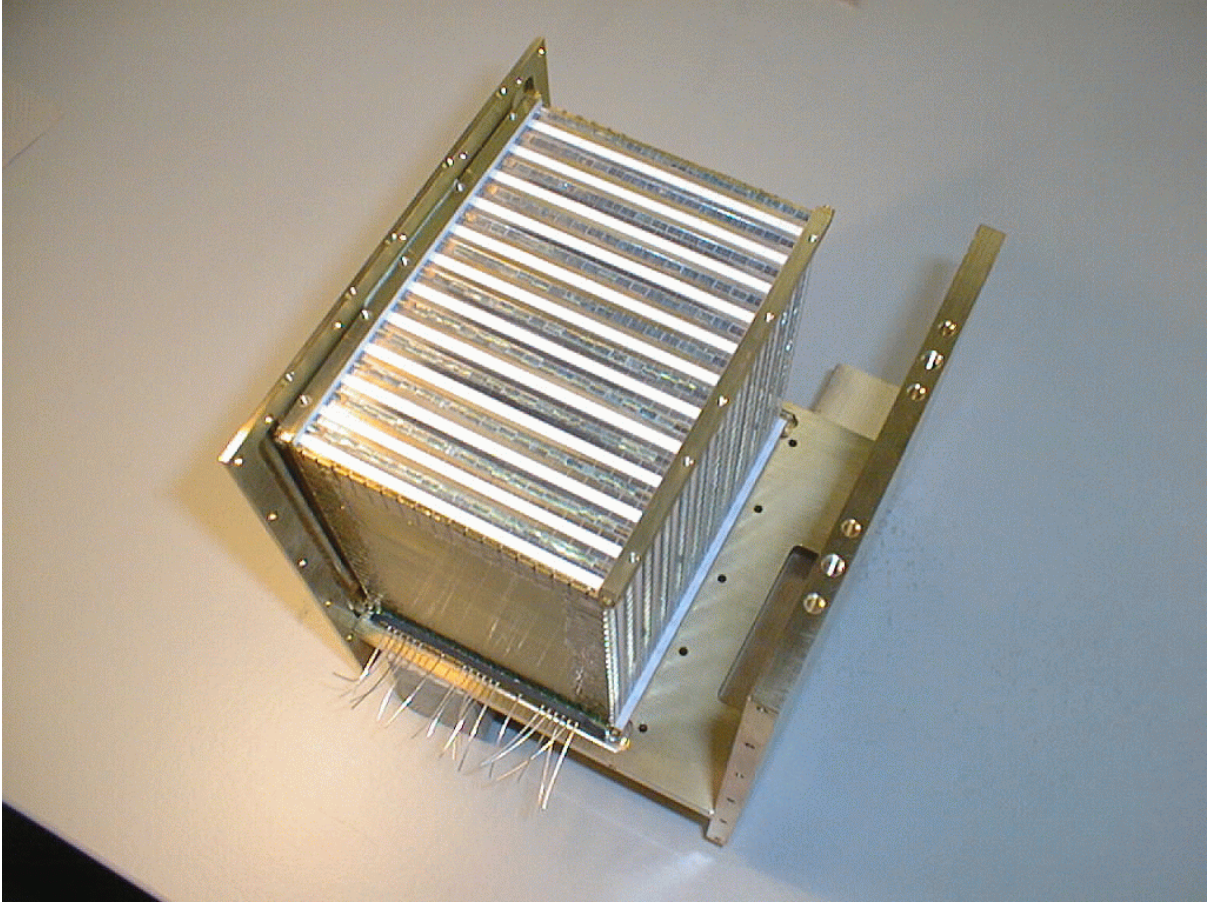
Abbildung 3.11: Foto der aktiven Struktur des VLQ-Kalorimeters. Zu erkennen ist die Haltestruktur bestehend aus den Führungsschienen und den Messingendplatten. Durch die Haltestruktur werden die Schichten aus Wolfram und den in Papier eingewickelten Szintillatorstreifen zusammengehalten.
