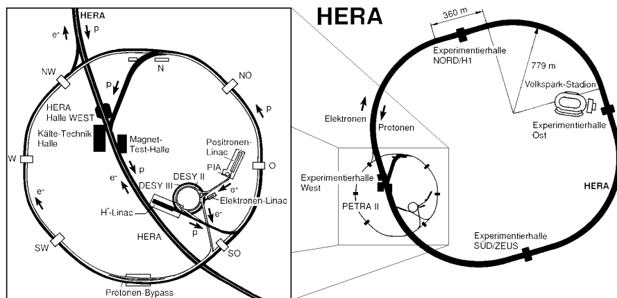
Abbildung 2.1: Die Speicherringanlage HERA mit den Experimentierhallen und vergrößert dargestellt die Vorbeschleuniger für HERA.
