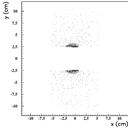
Abbildung 3.6: Trefferverteilung durch Synchrotronstrahlung im VLQ-Spurdetektor. Die Mehrzahl der Treffer ist nahe am Strahlrohr konzentriert [BERG96].
