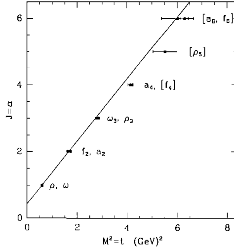
Abbildung 1.5: Die Regge-Trajektorie einiger Mesonen in einem Chew-Frautschi Diagramm [DON92].
