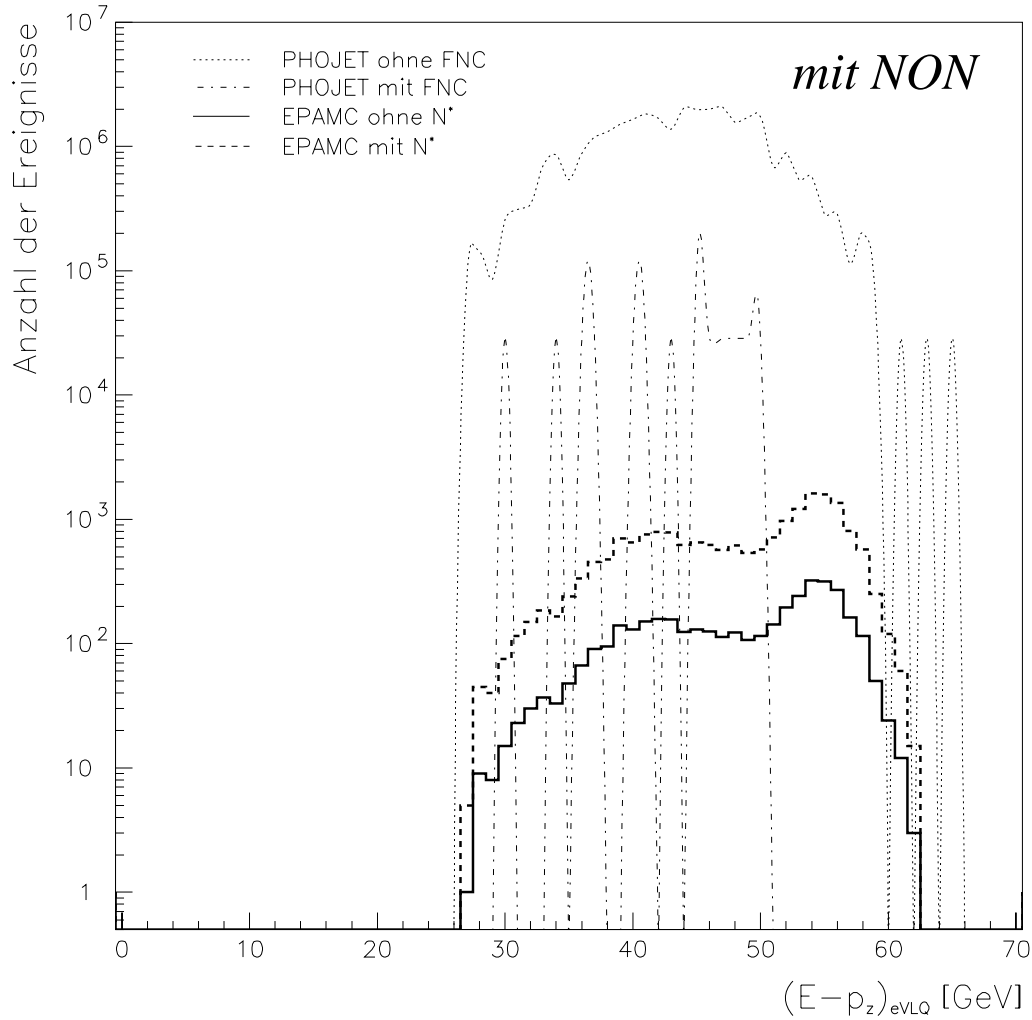
Abbildung 6.5: (E - p_z)_{eVLQ} -Verteilungen für die Triggerbedingung (6.5). Es sind sowohl die Verteilungen für den interessierenden Odderon-induzierten Prozeß (EPAMC mit N^* ) als auch der für den Untergrund aus Photoproduktionsereignissen (PHOJET mit FNC) dargestellt. Zum Vergleich sind die Verteilungen angegeben, bei denen die FNC-Bedingung nicht gestellt wurde (EPAMC ohne N^* , PHOJET ohne FNC).
