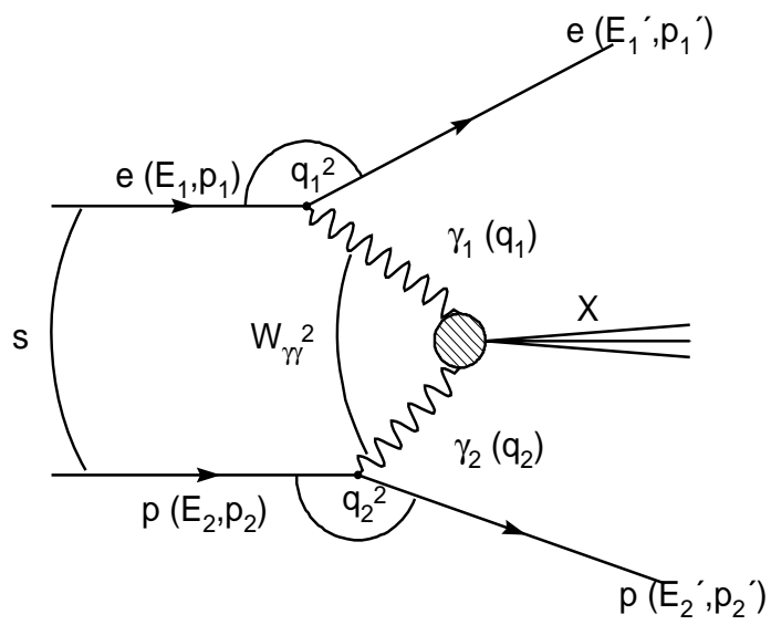
Abbildung 1.6: Bei dem Zwei-Photon Prozeß emittieren beide Strahlteilchen je ein Photon ( e + p \rightarrow e + p + \gamma_1 + \gamma_2 ), die miteinander wechselwirken, um den Endzustand X zu bilden ( \gamma_1 + \gamma_2 \rightarrow X ).
