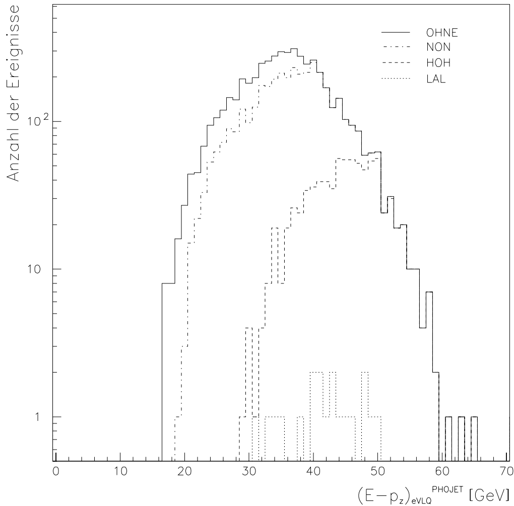
Abbildung 5.4: (E - p_z)_{eVLQ}^{PHOJET} -Verteilungen für die verschiedenen Triggerbedingungen (5.5) bis (5.8) für PHOJET-Ereignisse. Die Bedeutung der Abkürzungen OHNE, NON, HOH, LAL wird im Text beschrieben.
