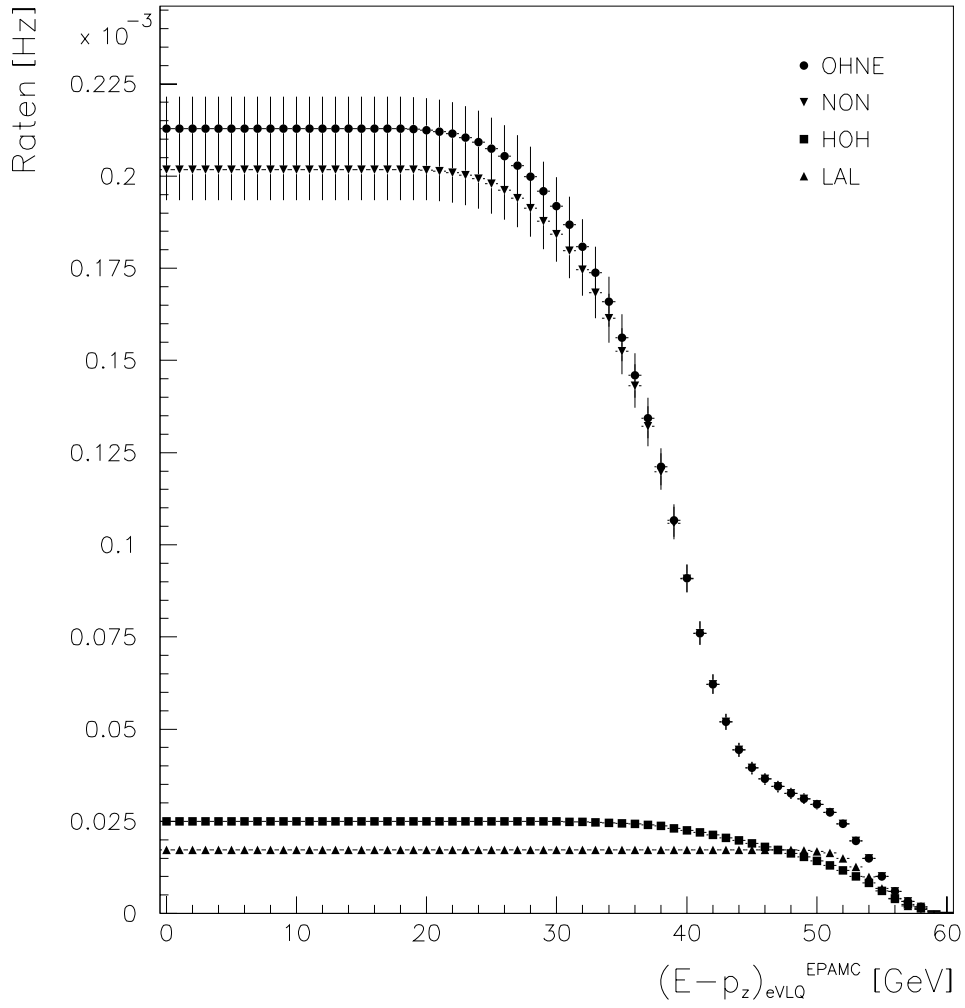
Abbildung 5.1: Ereignisraten im VLQ-Spektrometer aufgetragen gegen (E - p_z)_{eVLQ}^{EPAMC} für die verschiedenen Triggerbedingungen (5.5) bis (5.8) für EPAMC. Die Bedeutung der Abkürzungen OHNE, NON, HOH, LAL werden im Text beschrieben.
