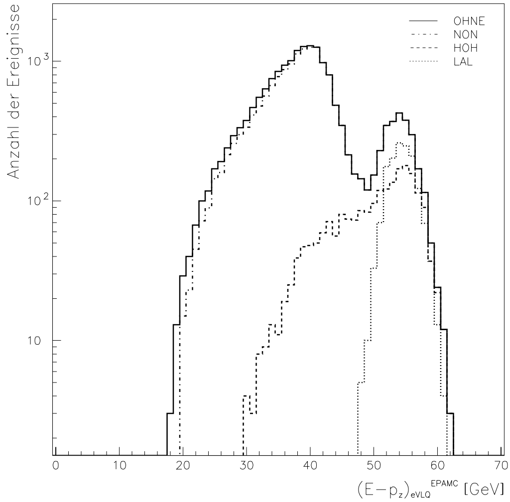
Abbildung 5.2: (E - p_z)_{eVLQ}^{EPAMC} -Verteilungen für die verschiedenen Triggerbedingungen (5.5) bis (5.8) für EPAMC-Ereignisse. Die Bedeutung der Abkürzungen OHNE, NON, HOH, LAL werden im Text beschrieben.
