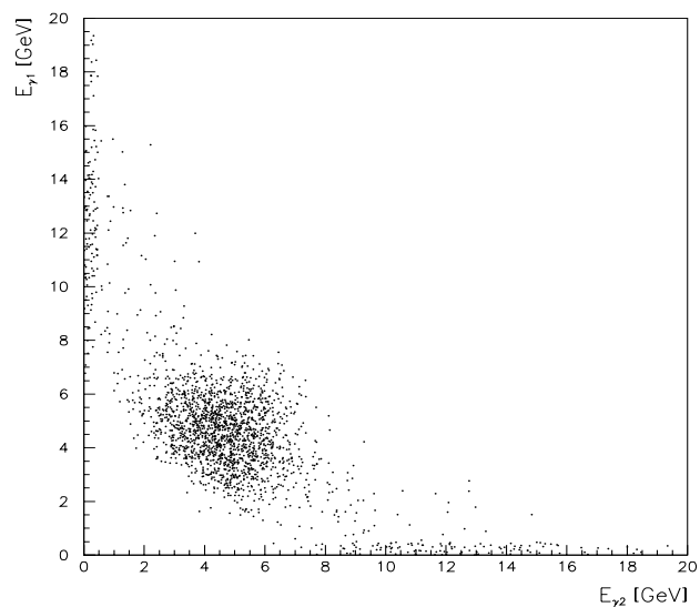
Abbildung 6.1: Energien der Photonen aus einem \pi^0 -Zerfall in einem Odderon-induzierten Prozeß gegeneinander aufgetragen für den Fall, daß beide Photonen im VLQ-Kalorimeter nachgewiesen wurden (EPAMC-Ereignisse). Die Photonen stammen aus dem Zerfall des \pi^0 's.
