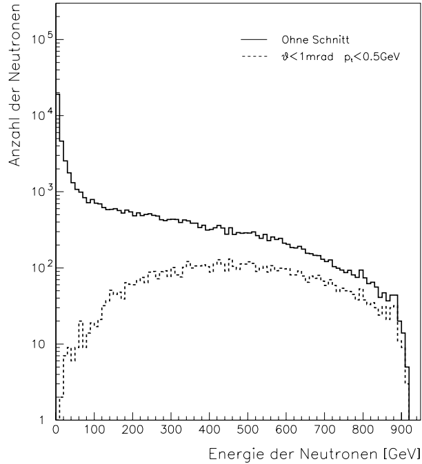
Abbildung 6.3: Energien der Neutronen aus 10^5 mit PHOJET generierten Ereignissen ohne jeglichen Schnitt (durchgezogene Kurve) und Energien der Neutronen mit einem p_t < 0.5 \text{ GeV} , die unter einem Winkel kleiner als 1 \text{ mrad} in Vorwärtsrichtung fliegen (gestrichelte Kurve).
