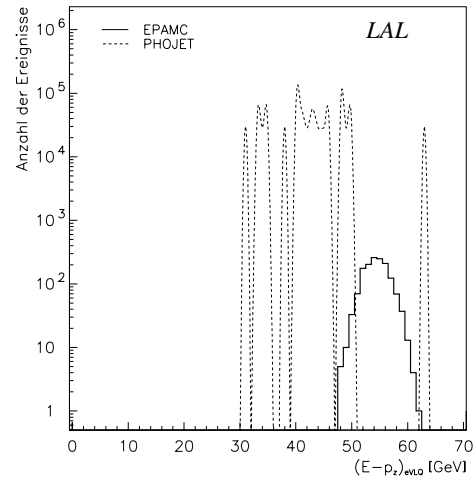
Abbildung 5.8: Vergleich der (E - p_z)_{eVLQ}^{EPAMC} - mit der (E - p_z)_{eVLQ}^{PHOJET} -Verteilung für Triggerbedingung LAL. Die Verteilungen sind auf dieselbe Luminosität normiert.
