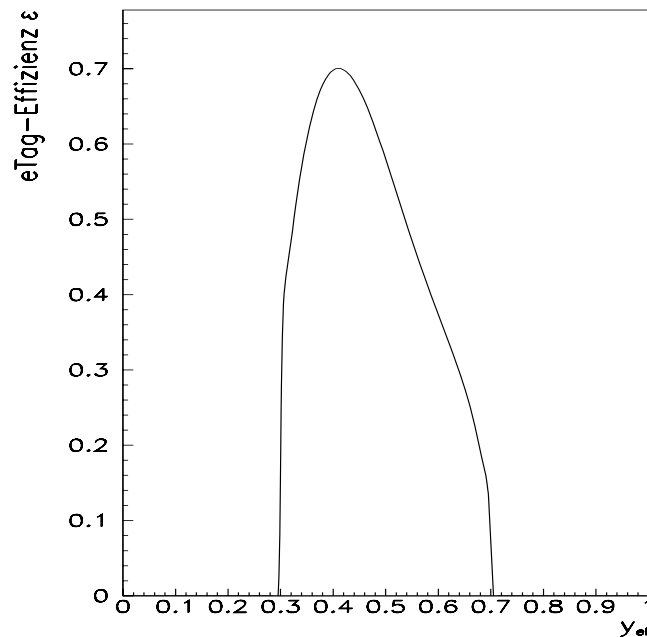
Abbildung 4.2: Effizienz des Elektron-Taggers als Funktion der Inelastizität y . Die Kurve ist durch Gleichung (4.5) an die Daten angepaßt.
