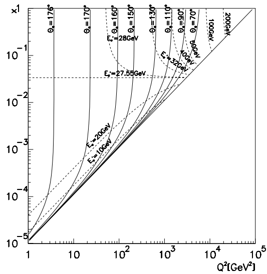
Abbildung 1.2: Die kinematische Ebene. Sie zeigt die Winkel (durchgezogen) und Energien (gestrichelt) des gestreuten Elektrons in Abhängigkeit von Q^2 und x (vgl. auch Abb. 3.9).
