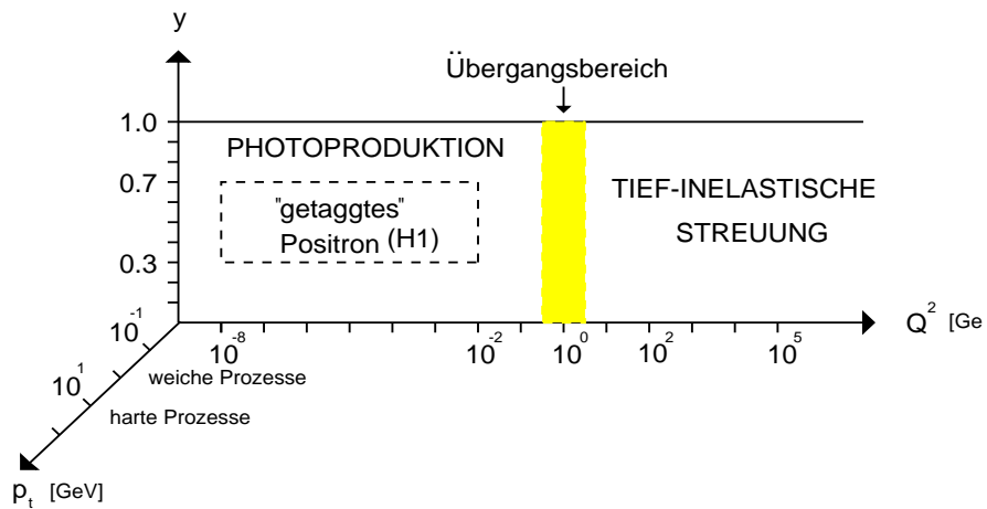
Abbildung 1.3: Kinematische Unterteilung der ep -Streuung in weiche und harte Prozesse in der Variablen p_t , sowie die Unterteilung in tief inelastische Streuung und Photoproduktion in der Variablen Q^2 .
