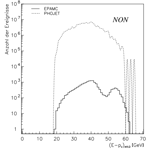
Abbildung 5.6: Vergleich der (E - p_z)_{eVLQ}^{EPAMC} - mit der (E - p_z)_{eVLQ}^{PHOJET} -Verteilung für Triggerbedingung NON. Die Verteilungen sind auf dieselbe Luminosität normiert.
