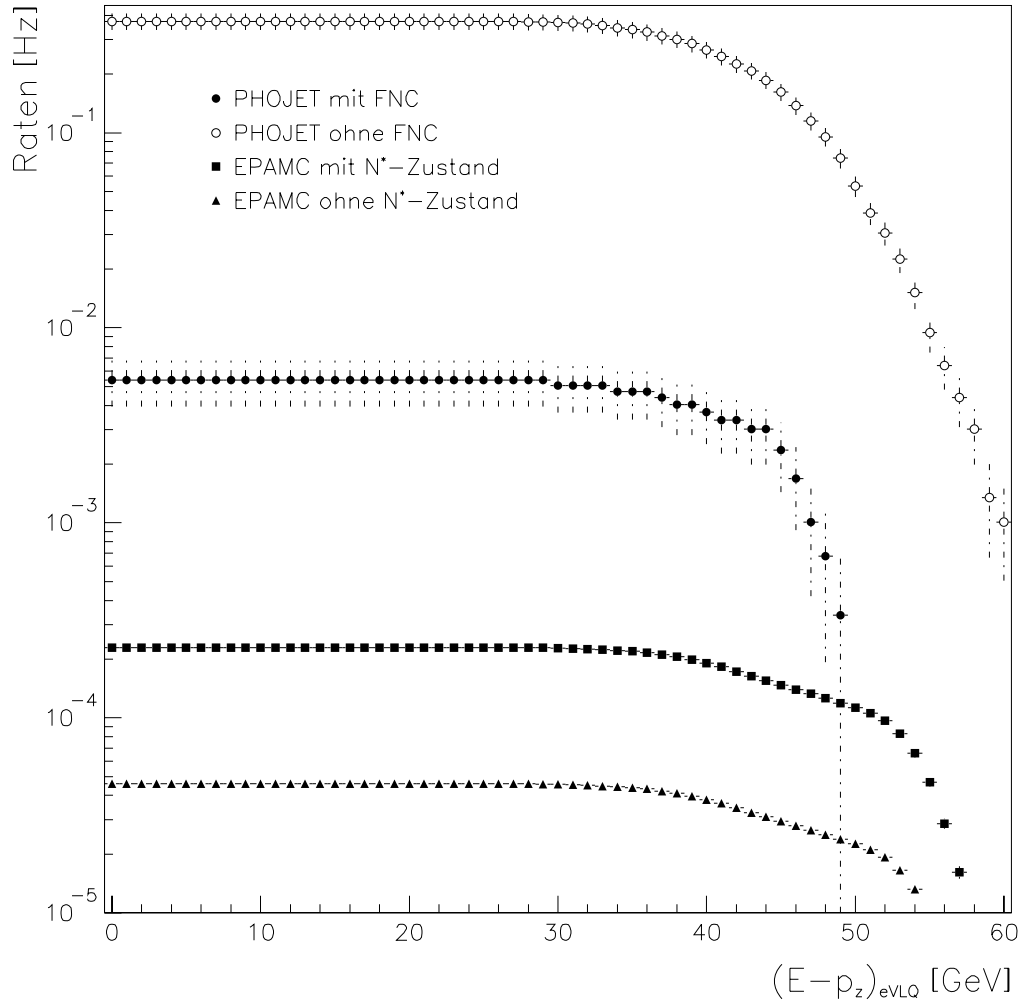
Abbildung 6.4: Ereignisraten im VLQ-Spektrometer aufgetragen gegen (E - p_z)_{eVLQ} für die Triggerbedingung (6.5) für das „Signal“ (EPAMC mit N^* -Zustand) und den Untergrund (PHOJET mit FNC). Zum Vergleich sind die zugehörigen Kurven ohne die FNC-Bedingung (EPAMC ohne N^* , PHOJET ohne FNC) miteingezeichnet.
