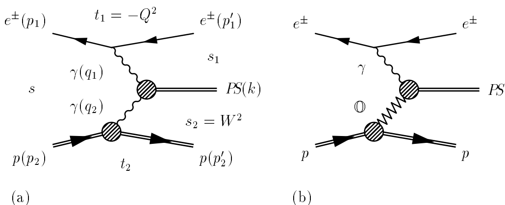
Abbildung 4.1: Feynman Diagramme zur Erzeugung pseudoskalarer Mesonen in der ep -Streuung bei hohen Energien mit (a) Photon- und (b) Odderon-Austausch.
