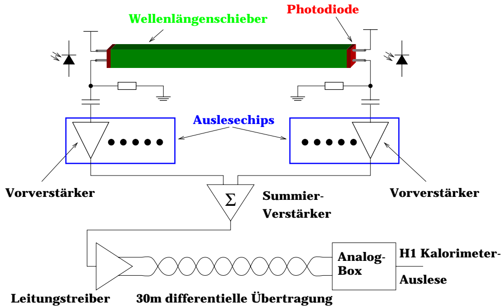
Abbildung 3.13: Die Ausleseketten des VLQ-Kalorimeters für einen Kanal. Jeder Wellenlängenschieber wird an beiden Enden von je einer Photodiode ausgelesen. Das Photodiodensignal wird durch die Ladungsverstärker auf den Auslesechips (FroPhoDiChi) verstärkt und anschließend die Signale von beiden Enden summiert. Das Summensignal wird dann über einen Leitungstreiber differentiell über ca. 30 m Kabel zur Analog-Box transportiert [STELL98].
