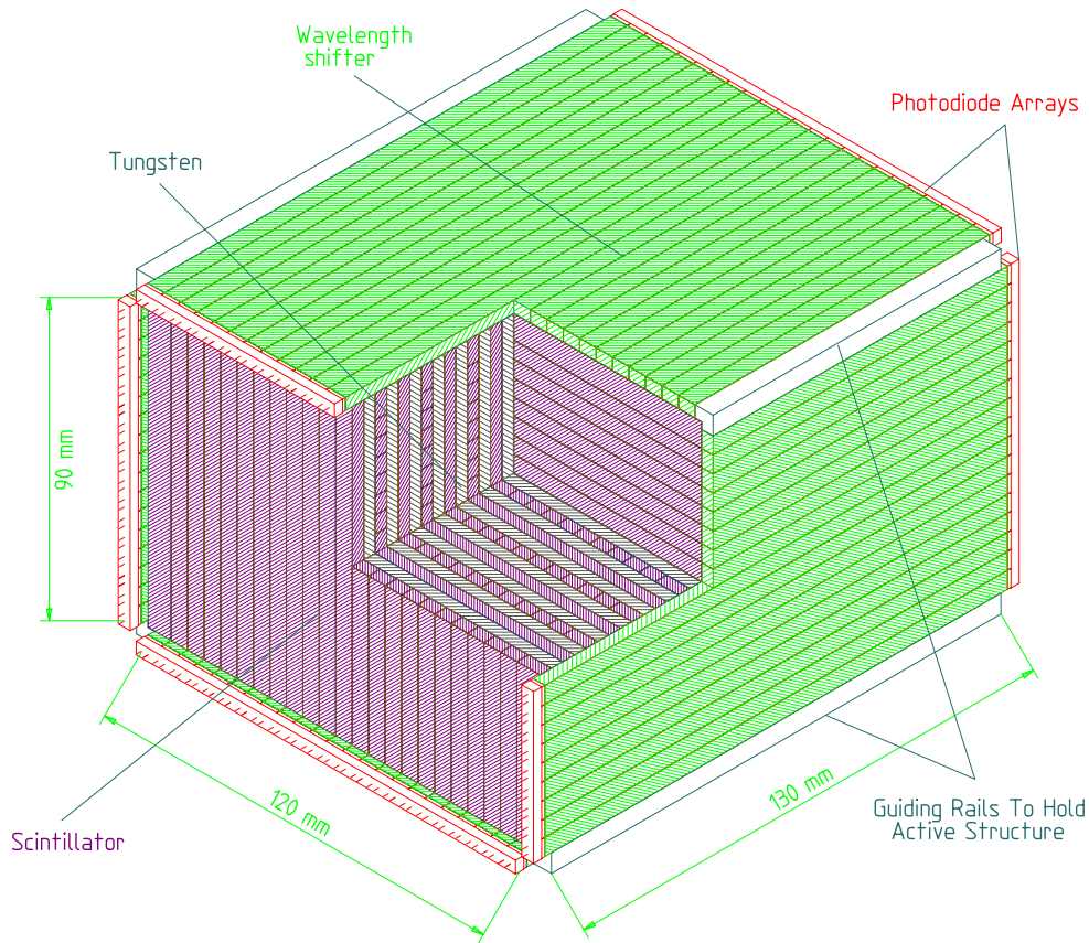
Abbildung 3.10: Die optimierte aktive Struktur des VLQ-Kalorimeters (s. Tabelle 3.1).
