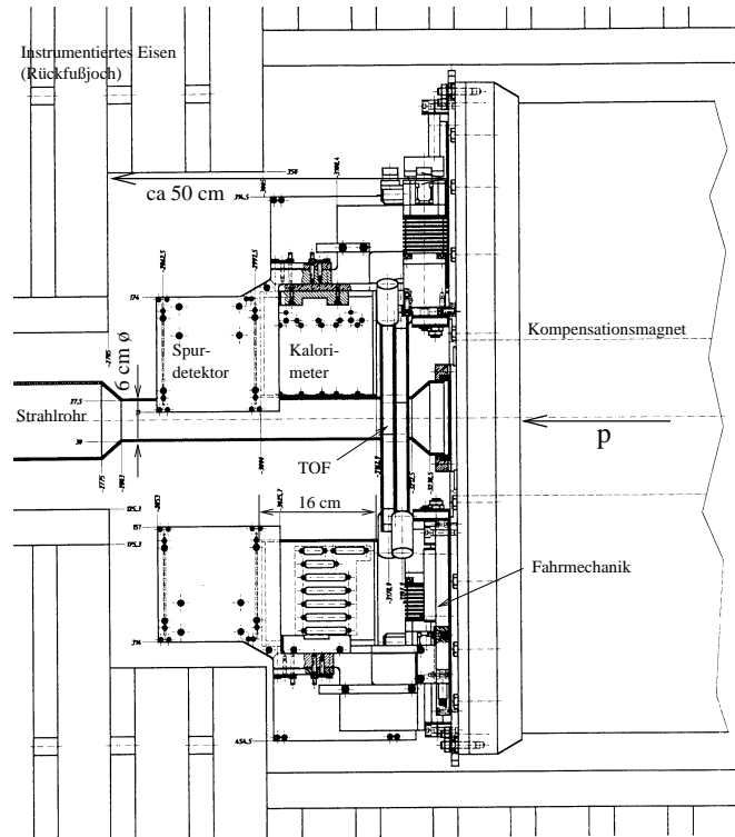
Abbildung 3.5: Der Einbaubereich des VLQ-Spektrometers im Detail. Rechts ist der Kompensationsmagnet zu erkennen, an dem das gesamte Spektrometer befestigt ist.
