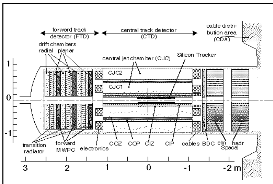
Abbildung 2.3: Schematischer Aufbau der Spurkammern von H1 im Längsschnitt.
