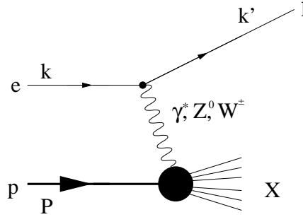
Abbildung 1.1: Feynman-Diagramm der Elektron-Proton-Streuung in Bornscher Näherung.
