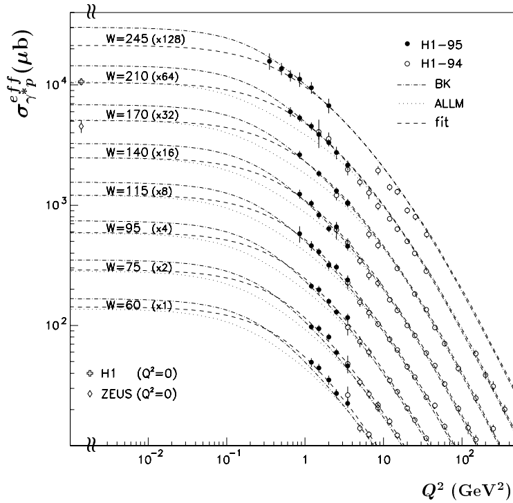
Abbildung 3.1: Der vom Detektor H1 gemessene Photon-Proton-Wirkungsquerschnitt als Funktion von Q^2 mit der invarianten Masse W als Parameter. Die Kurven sind mit den in Klammern angegebenen Faktoren skaliert [BERG96].
