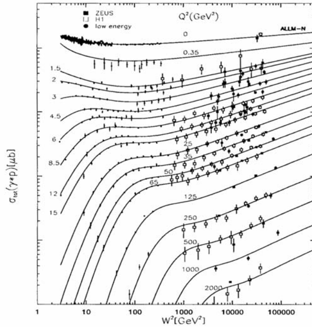
Abbildung 3.3: Der totale Photoabsorptions-Wirkungsquerschnitt aufgetragen gegen W^2 für verschiedene Q^2 .
