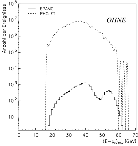
Abbildung 5.5: Vergleich der (E - p_z)_{eVLQ}^{EPAMC} - mit der (E - p_z)_{eVLQ}^{PHOJET} -Verteilung für Triggerbedingung OHNE. Die Verteilungen sind auf dieselbe Luminosität normiert.
