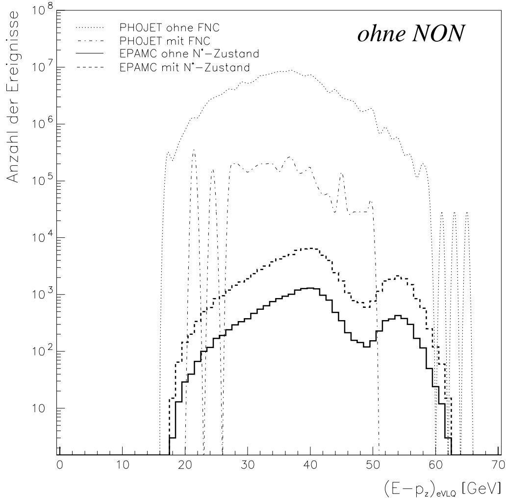
Abbildung 6.6: (E - p_z)_{eVLQ} für die Triggerbedingung (6.5) ohne die darin enthaltene Energieforderung ( TOPNOISE.OR.TOPNOISE ). Es sind sowohl die Verteilungen für den interessierenden Odderon-induzierten Prozeß (EPAMC mit N^* ) als auch der für den Untergrund aus Photoproduktionsereignissen (PHOJET mit FNC) dargestellt. Zum Vergleich sind die Verteilungen angegeben, bei denen die FNC-Bedingung nicht gestellt wurde (EPAMC ohne N^* , PHOJET ohne FNC).
