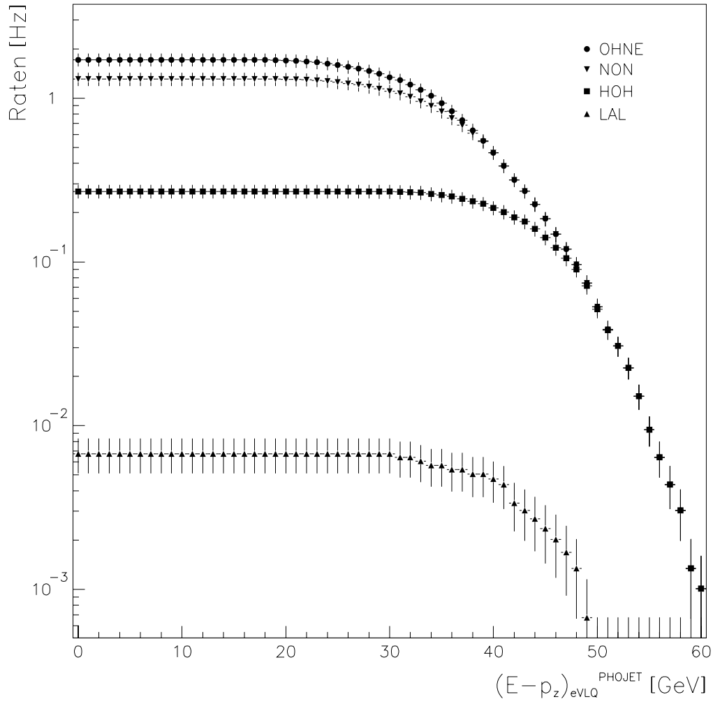
Abbildung 5.3: Ereignisraten im VLQ-Spektrometer aufgetragen gegen (E - p_z)_{eVLQ}^{PHOJET} für die verschiedenen Triggerbedingungen (5.5) bis (5.8) für PHOJET-Ereignisse. Die Bedeutung der Abkürzungen OHNE, NON, HOH, LAL wird im Text beschrieben.
