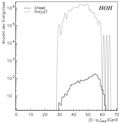
Abbildung 5.7: Vergleich der (E - p_z)_{eVLQ}^{EPAMC} - mit der (E - p_z)_{eVLQ}^{PHOJET} -Verteilung für Triggerbedingung HOH. Die Verteilungen sind auf dieselbe Luminosität normiert.
