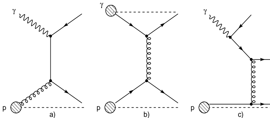
Abbildung 1.4: Verschiedene Klassen der Photoproduktion: a) der direkte Prozeß, b) der eigentliche VDM Prozeß und c) der anomale Prozeß
