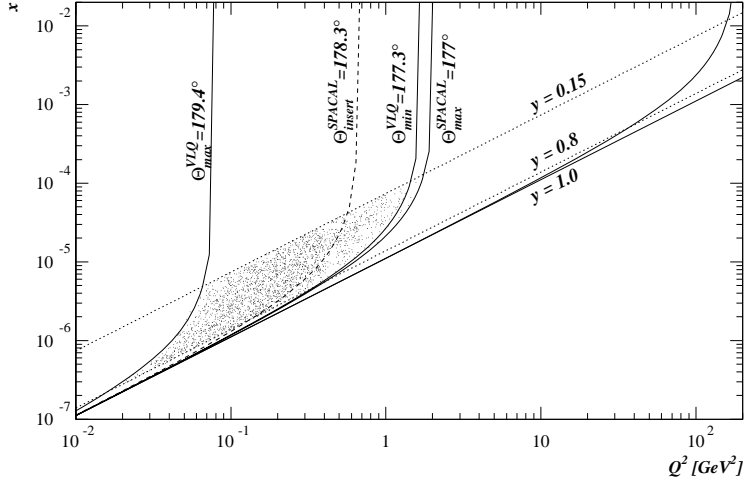
Abbildung 3.9: Akzeptanzbereich des VLQ-Spektrometers in der x - Q^2 Ebene. Es ist deutlich der Überlappbereich von VLQ und Spacal zu erkennen [BERG96] (vgl. auch Abbildung 1.2).
