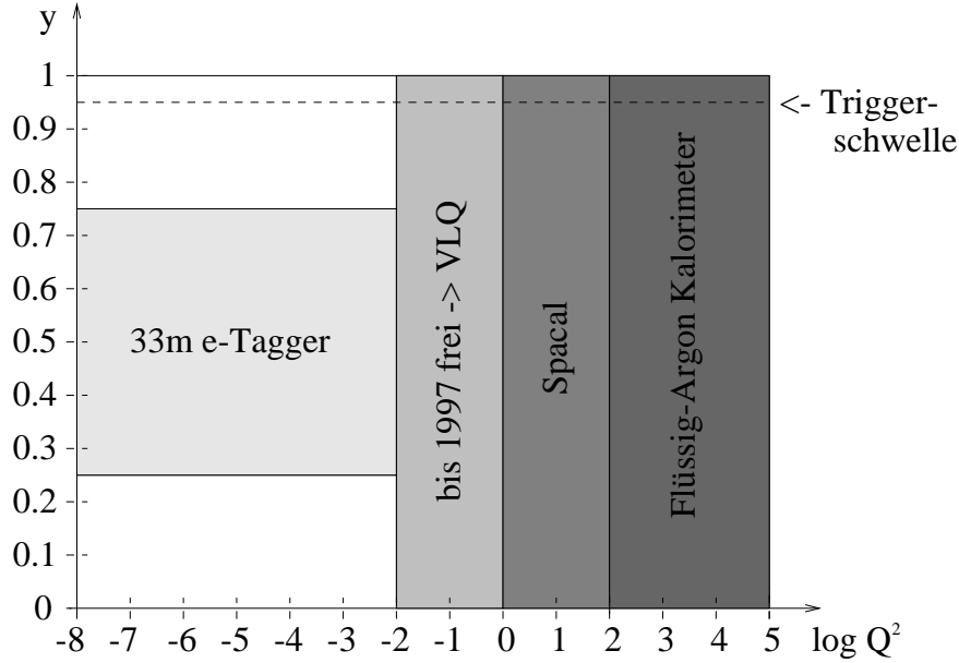
Abbildung 3.2: Akzeptanzbereiche der Subdetektoren des Detektors H1 in der y - Q^2 -Ebene aufgetragen.
