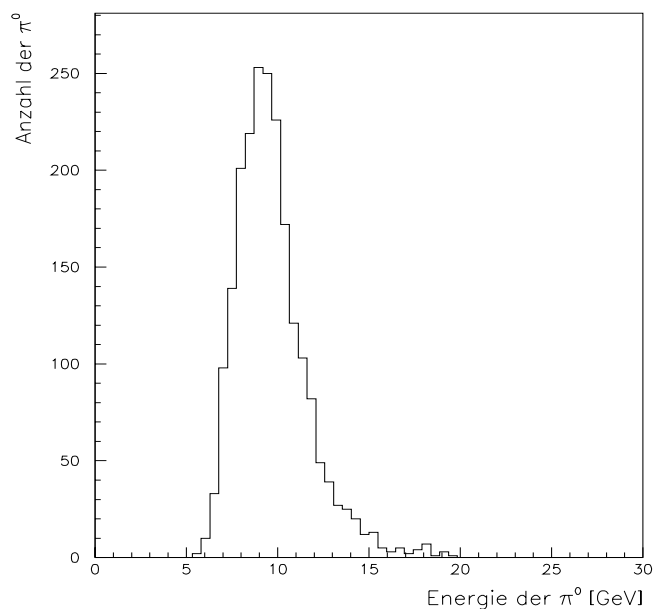
Abbildung 6.2: Energieverteilung der \pi^0 's aus einem Odderon-induzierten Prozeß (EPAMC-Ereignisse).
