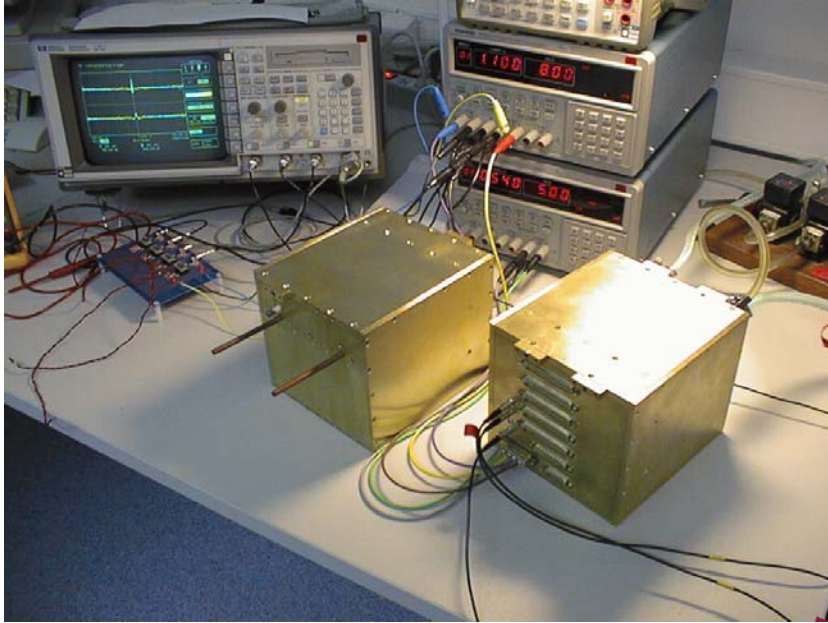
Abbildung 3.12: Die beiden fertiggestellten VLQ-Kalorimeter Module.
