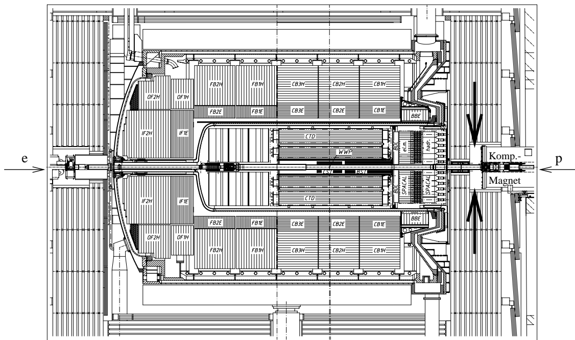
Abbildung 3.4: Querschnitt durch den Detektor H1. Die Pfeile verweisen auf die Stelle, an der das VLQ-Spektrometer eingebaut ist. Von der linken Seite kommen die Elektronen, von der rechten Seite die Protonen.
