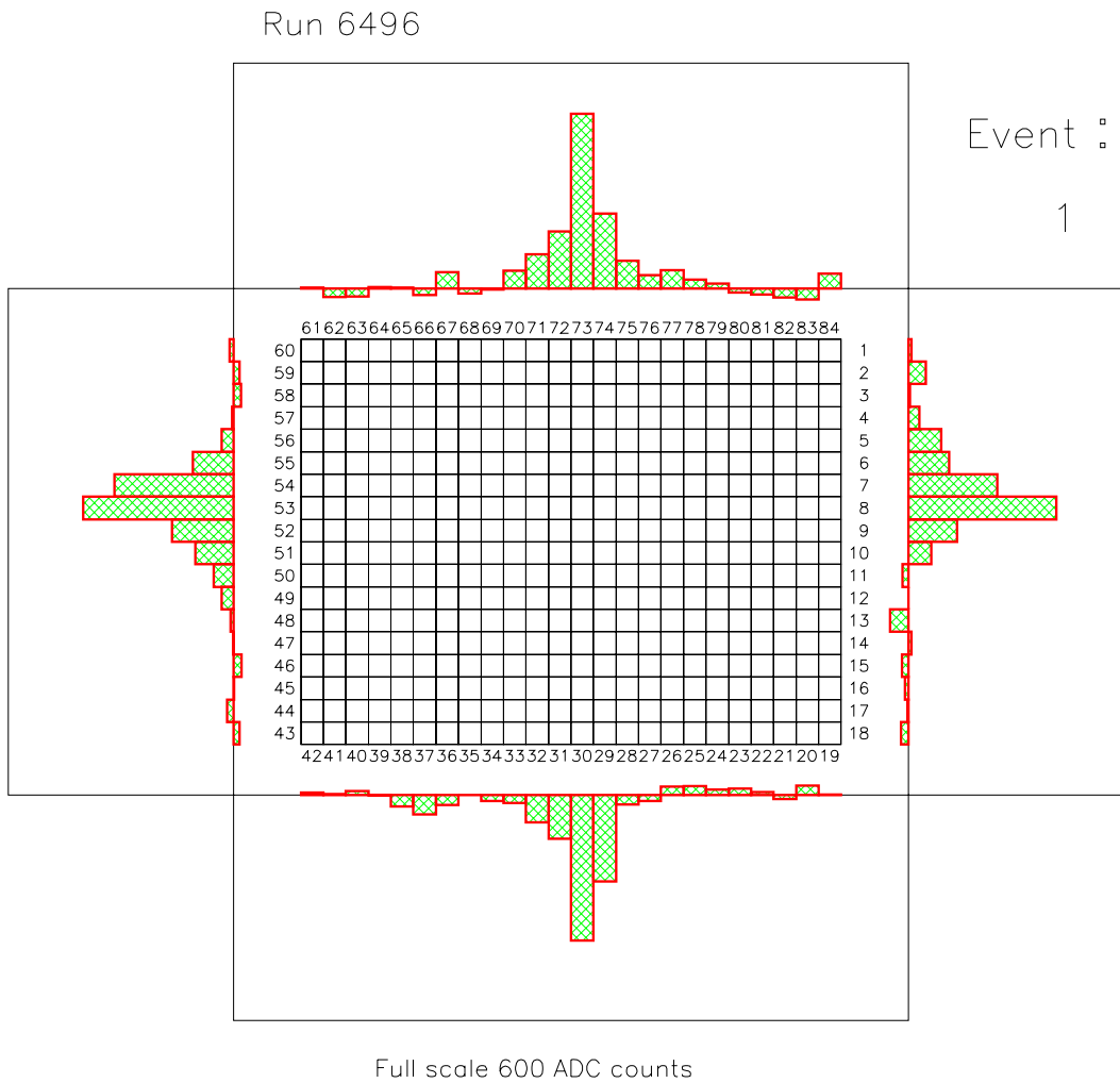
Abbildung 3.8: Eventdisplay eines Elektrons mit einer Energie von 5 GeV (DESY-Teststrahl).
