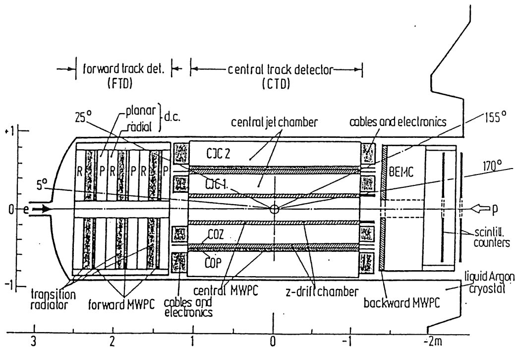
Abb. 1.3: Seitenansicht der Spurkammern des H1-Detektors mit Vorwärtsspurkammern, zentralen Spurkammern und rückwärtigen Detektoreinheiten aus [BÜR87].
