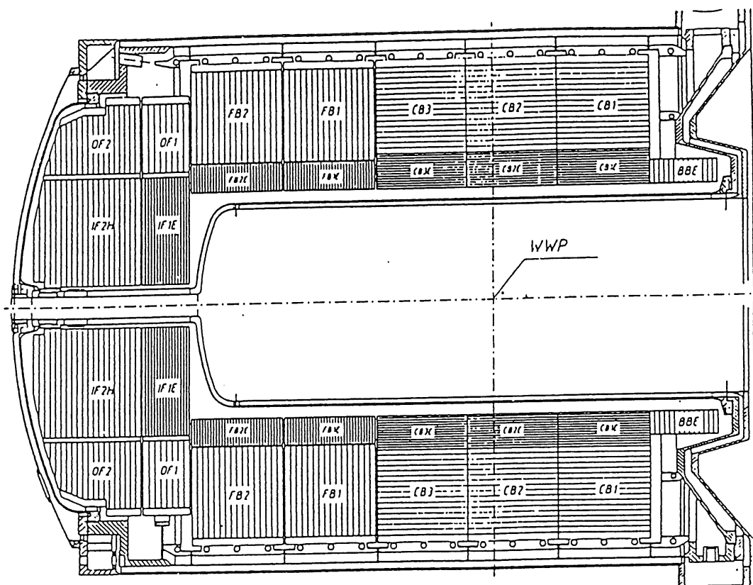
Abb. 1.5: Längsschnittansicht des H1-Flüssig-Argon-Kalorimeters (aus [TEC89]).
