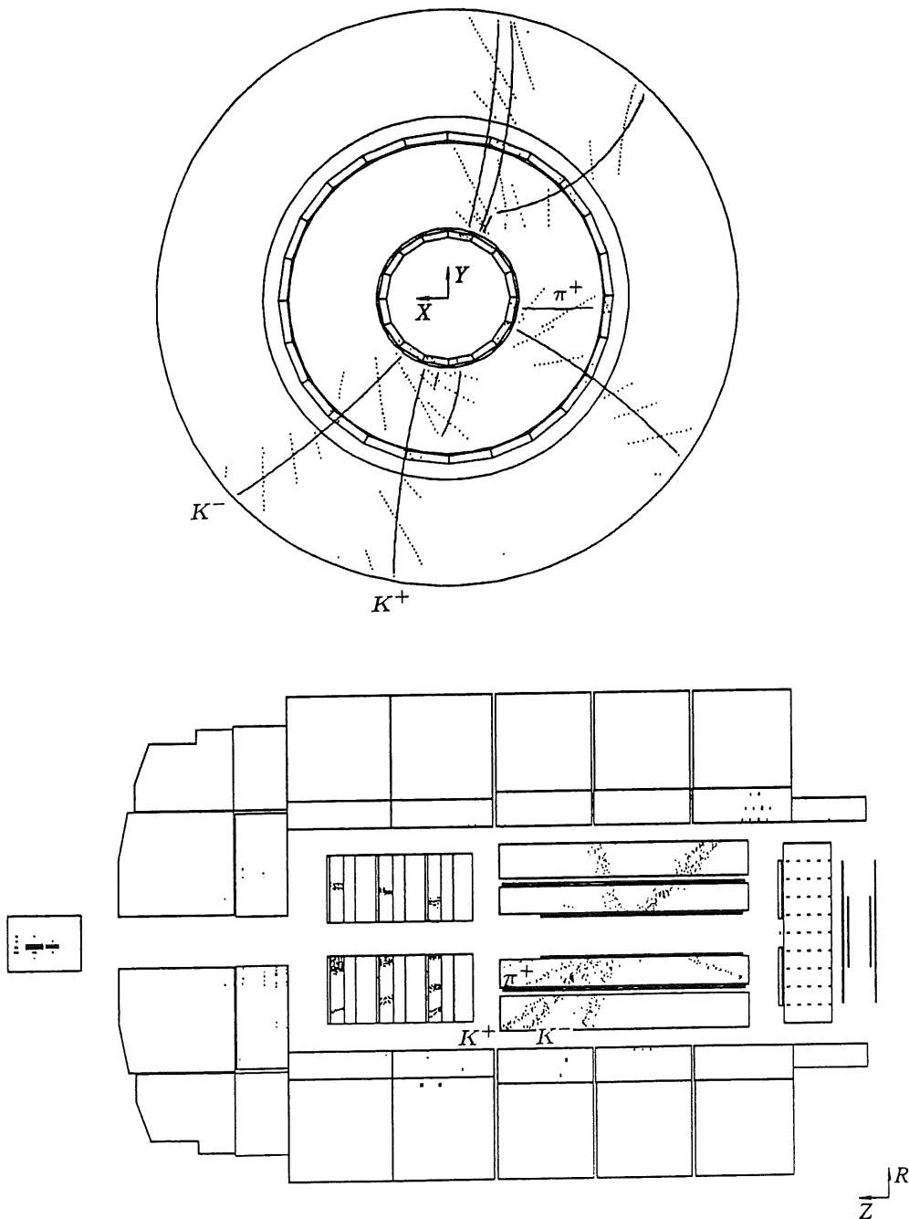
Abb. 4.2: Graphische Darstellung des Events mit der Run-Nummer 2 und der Event-Nummer 3807 aus dem Datensatz \Phi -Simulation. Das obere Teilbild zeigt eine radiale Ansicht der zentralen Spurkammern des H1-Detektors. Im unteren Teilbild ist eine Längsansicht des Detektors zu sehen, auf der man die zentralen Spurkammern, die Vorwärts-Spurkammern, sowie die LAr-, BEMC- und PLUG-Kalorimeter erkennt. Die Endzustandsteilchen des Zerfalls D_s^+ \rightarrow K^+ K^- \pi^+ sind gekennzeichnet.
