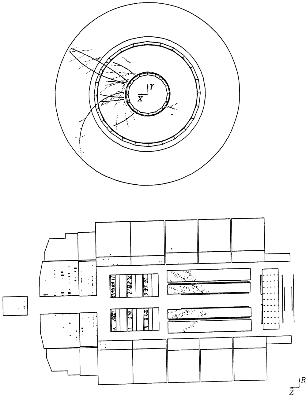
Abb. 8.3: Graphische Darstellung des Events mit der Run-Nummer 2 und der Event-Nummer 2 aus dem Datensatz \gamma -Gluon-Fusion. Das obere Teilbild zeigt eine radiale Ansicht der zentralen Spurkammern des H1-Detektors. Im unteren Teilbild ist eine Längsansicht des Detektors zu sehen, auf der man die zentralen Spurkammern, die Vorwärts-Spurkammern, sowie die LAr-, BEMC- und PLUG-Kalorimeter erkennt. Infolge seiner asymmetrischen Topologie wird dieses Ereignis durch den Schnitt auf die mittlere Pseudorapidität verworfen.
