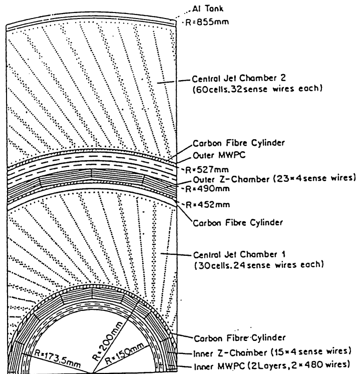
Abb. 1.4: Ausschnitt aus einer Querschnittsansicht der zentralen Spurkammern des H1-Detektors (aus [BÜR89]).
