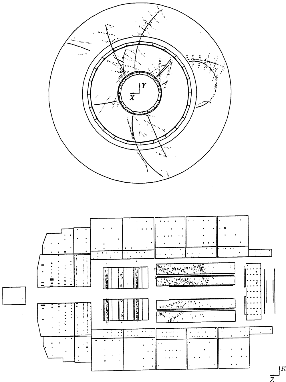
Abb. 7.3: Graphische Darstellung des Events mit der Run-Nummer 26207 und der Event-Nummer 24056 aus dem Datensatz Untergrund. Das obere Teilbild zeigt eine radiale Ansicht der zentralen Spurkammern des H1-Detektors. Im unteren Teilbild ist eine Längsansicht des Detektors zu sehen, auf der man die zentralen Spurkammern, die Vorwärts-Spurkammern, sowie die LAr-, BEMC- und PLUG-Kalorimeter erkennt. Dieses Ereignis wird durch die Energieflußschnitte verworfen.
