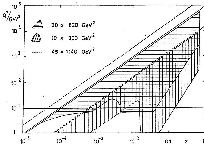
Abb. 2.2: Der bei HERA zugängliche Bereich in der x - Q^2 -Ebene für drei verschiedene Energie-Bereiche (Erläuterung siehe Text, Abb. aus [PRO91]).
